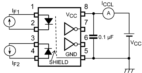
図 13.1.4 ICCL測定回路
