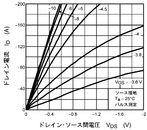
図 9.2 I_D - V_{DS}
