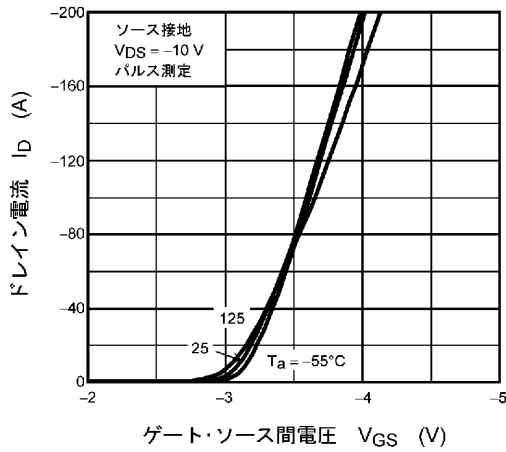
図 9.3 I_D - V_{GS}
