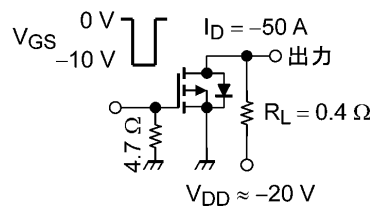
図 6.2.1 スwitchング時間の測定回路
