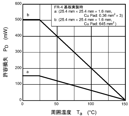
図 7.12 P_D - T_a
