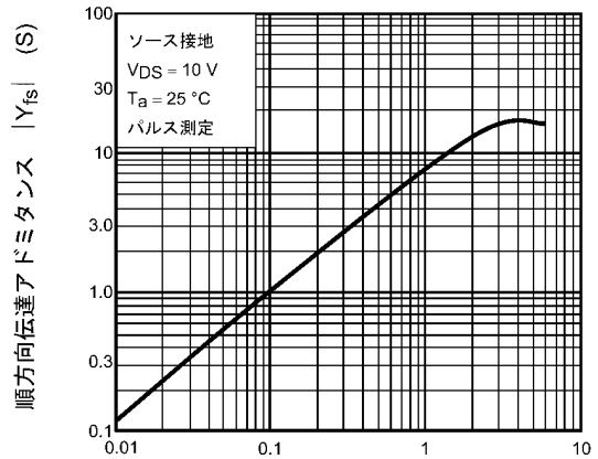
図 7.8 |Y_{fs}| - I_D
