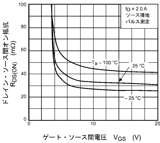
図 7.3 R_{DS(ON)} - V_{GS}
