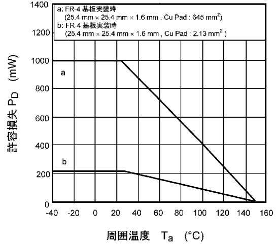
図 7.14 P_D - T_a
