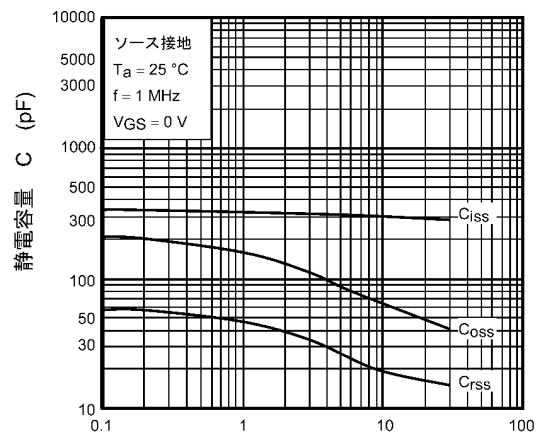
図 7.10 C - V_{DS}
