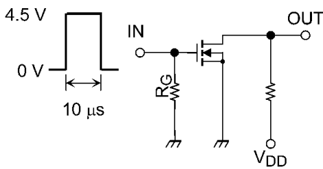
図 5.3.1 スwitching時間の測定回路
