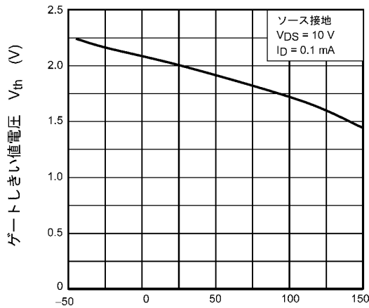
図 9.7 V_{th} - T_a
