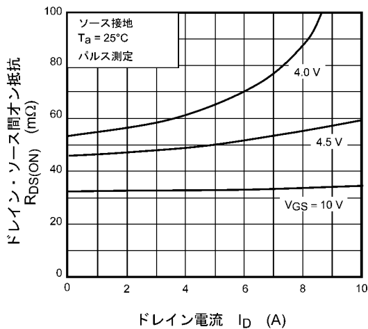
図 7.5 R_{DS(ON)} - I_D
