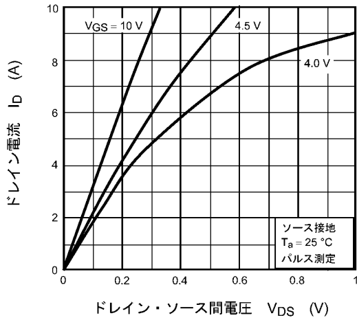
図 7.1 I_D - V_{DS}
