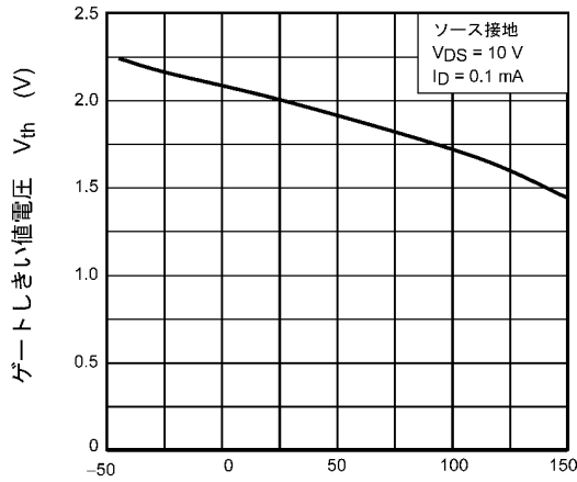
図 7.7 V_{th} - T_a
