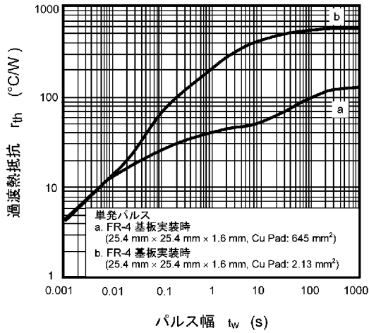
図 7.13 r_{th} - t_w
