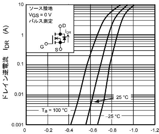
図 7.9 I_{DR} - V_{DS}
