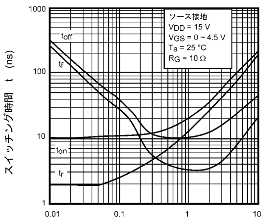
図 7.11 t - I_D
