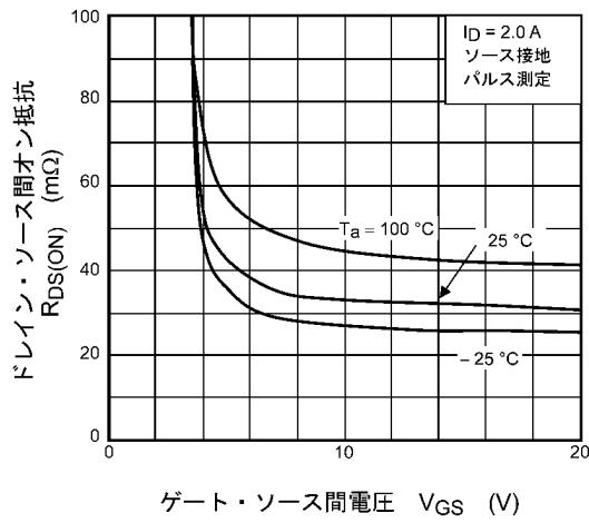
図 9.3 R_{DS(ON)} - V_{GS}
