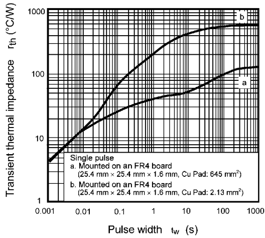
図 9.13 r_{th} - t_w
