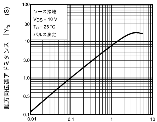
図 9.8 |Y_{fs}| - I_D
