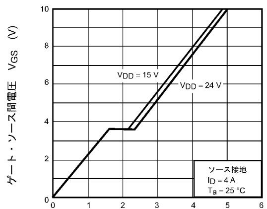
図 7.12 ダイナミック入力特性
