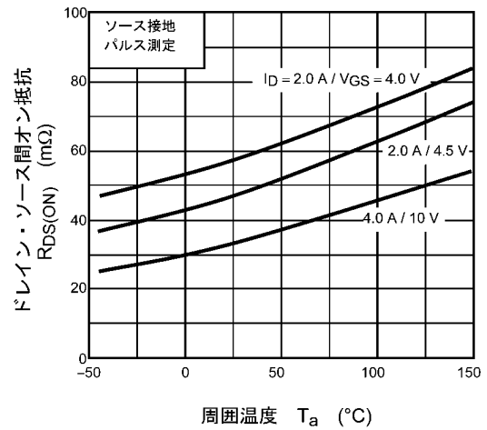
図 7.6 R_{DS(ON)} - T_a
