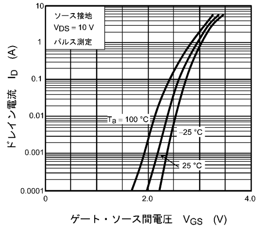
図 7.2 I_D - V_{GS}
