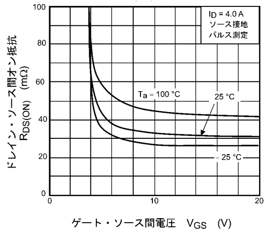
図 7.4 R_{DS(ON)} - V_{GS}
