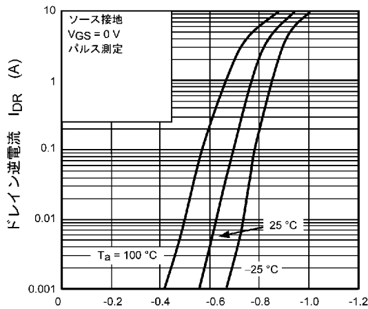
図 9.9 I_{DR} - V_{DS}
