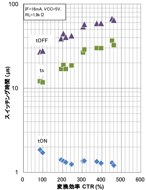
図 2.15 CTR-スイッチング時間 (飽和動作) 特性
