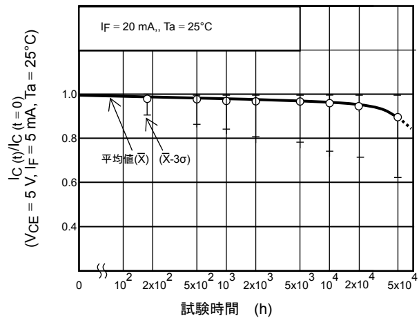
図 2.14 寿命試験データ例*
