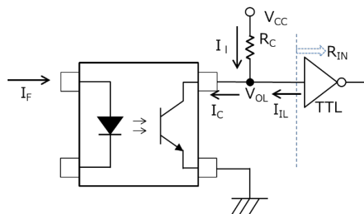
図 2.18 R_L は R_{IN} と R_C で表せる
