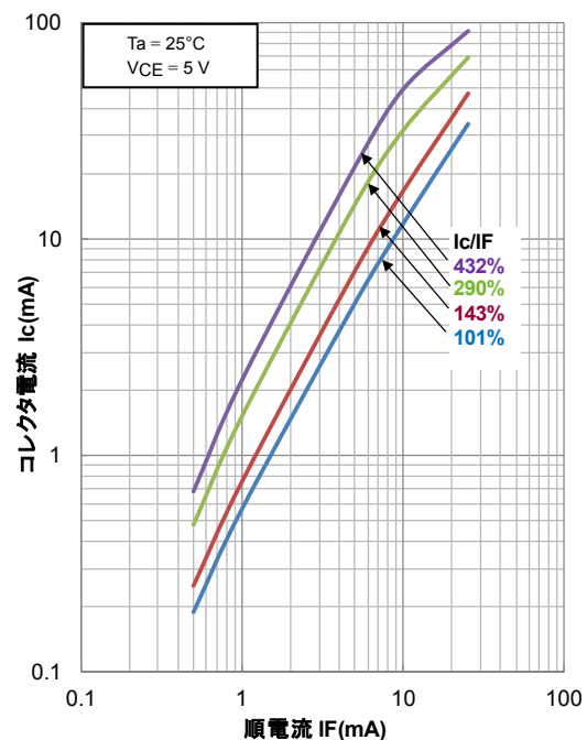
図 2.20 I_C/I_F をパラメータにした順電流-コレクタ電流特性
