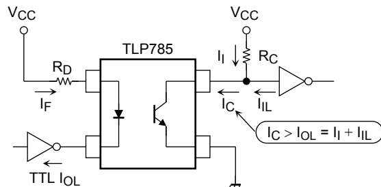
図 2.12 4 ピンの トランジスタカプラを使った TTL 間インタフェース回路
