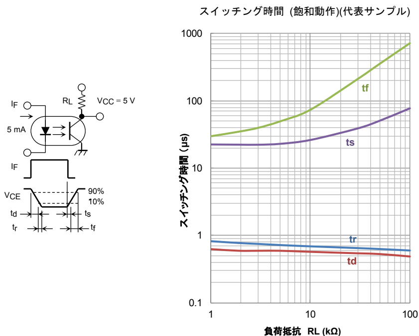
図 1.6 スwitching時間- R_L 特性
