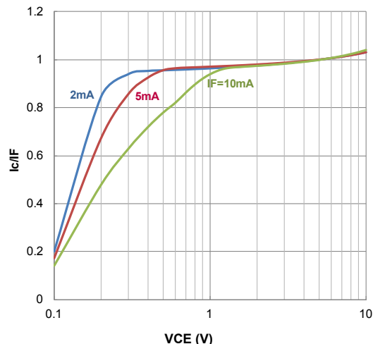
図 2.21 I_C/I_F - V_{CE} 特性
