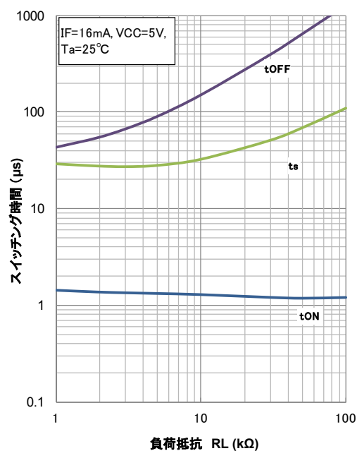
図 2.17 負荷抵抗-スイッチング時間 (飽和動作) 特性
