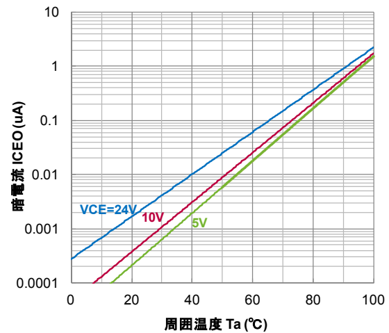
図 2.19 V_{CE} をパラメータにした周囲温度-暗電流特性
