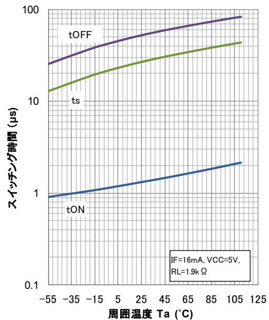
図 2.16 周囲温度-スイッチング時間 (飽和動作) 特性
