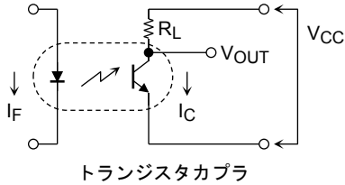
図 2.7 トランジスタカプラ
