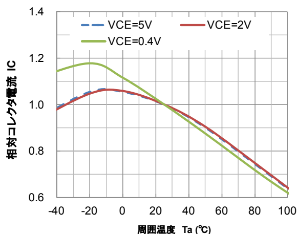
図 2.22 周囲温度-コレクタ電流特性
