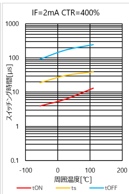
図 4.225 スイッチング時間 - Ta 特性(CTR=400%)
