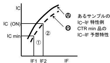
図 2.9 I_C-I_F 特性例
