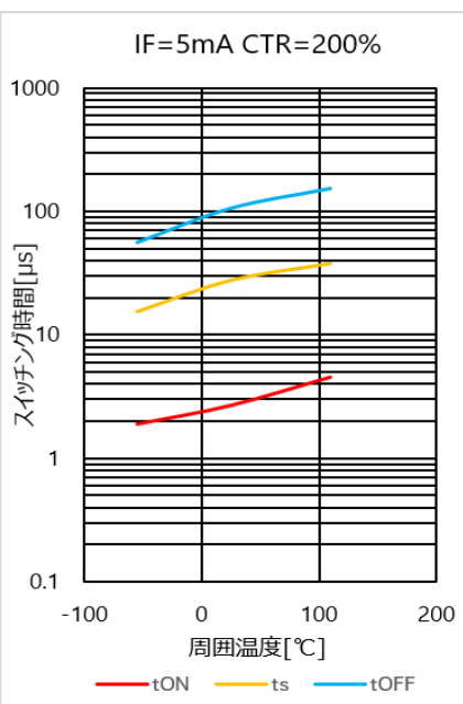
図 4.227 スイッチング時間 - Ta 特性(CTR=200%)
