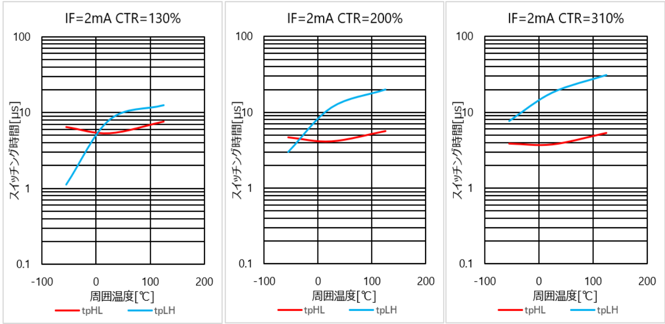
図 4.330 スwitchング時間 - Ta 特性(CTR=130%)
