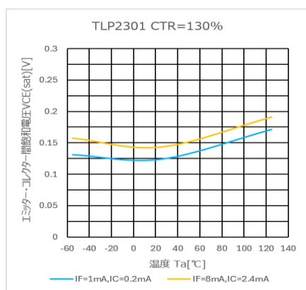
図 4.315 V_{CE} - T_a 特性 (CTR=130%)
