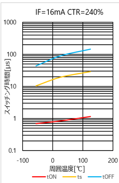
図 4.187 スイッチング時間 – Ta 特性(CTR=240%)
