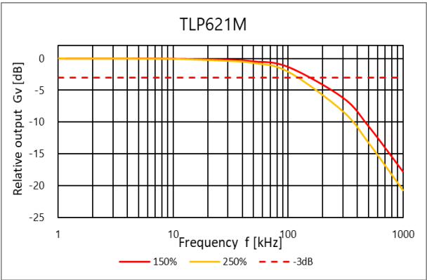
图 4.307 相对出力 G_v – 周波数
