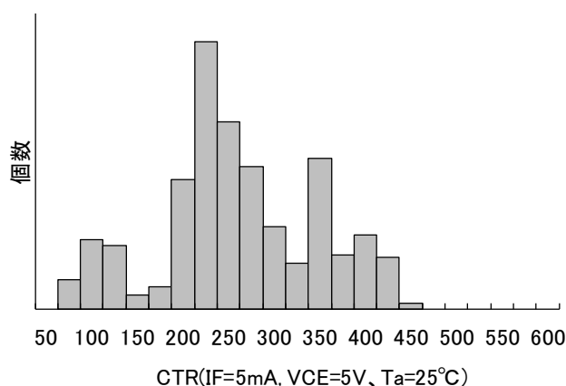
図 1.2 CTR 分布例
