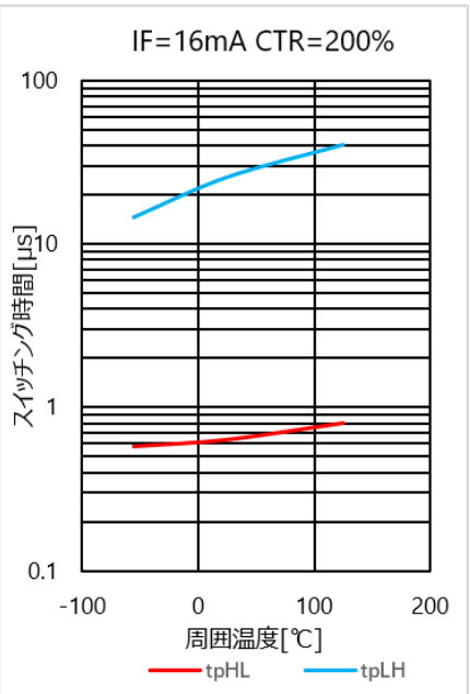
図 4.346 スイッチング時間 - Ta 特性(CTR=200%)
