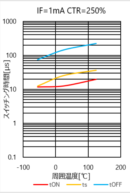
図 4.298 スイッチング時間 – Ta 特性(CTR=250%)
