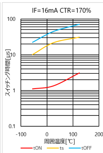
図 4.261 スwitchング時間 - T_a 特性(CTR=170%)
