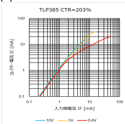
図 4.206 I_C - I_F 特性 (CTR=203%)
