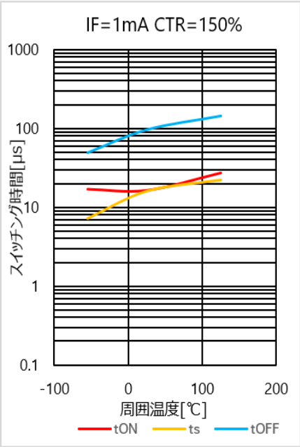
図 4.297 スイッチング時間 – Ta 特性(CTR=150%)
