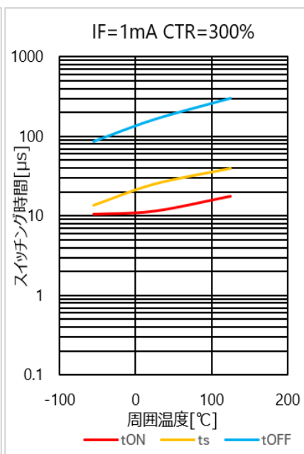
図 4.265 スイッチング時間 - Ta 特性(CTR=300%)
