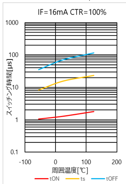
図 4.34 スイッチング時間 - T_a 特性(CTR = 100 %)
