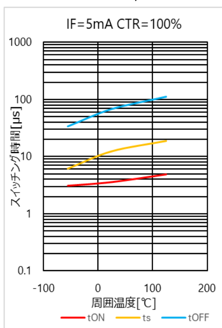
図 4.31 スイッチング時間 - T_a 特性(CTR = 100 %)
