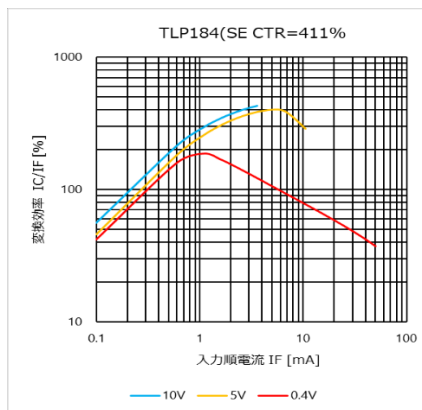
図 4.58 I_C/I_F - I_F 特性 (CTR=411%)
