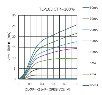
図 4.4 I_C - V_{CE} 特性 (CTR = 100 %)
