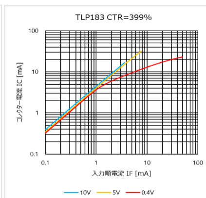
図 4.12 I_C - I_F 特性 (CTR = 399 %)
