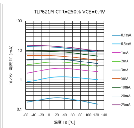
図 4.292 I_C - T_a 特性 (CTR=250%)
