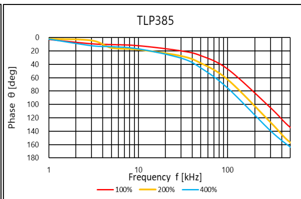
図 4.235 位相 \theta - 周波数
