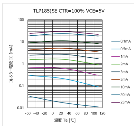
図 4.100 I_C - T_a 特性 (CTR=100%)
