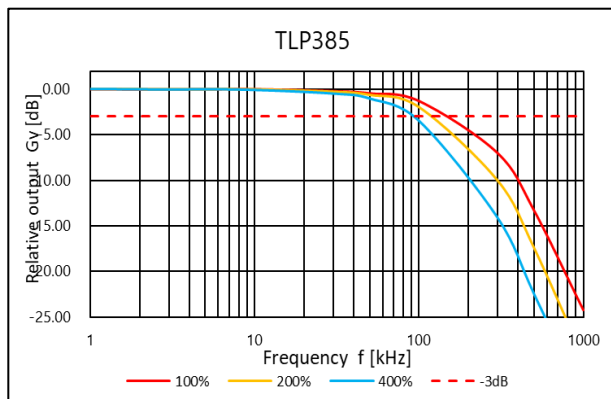
図 4.234 相対出力 G_v - 周波数
