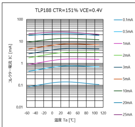
図 4.137 I_C - T_a 特性 (CTR=151%)
