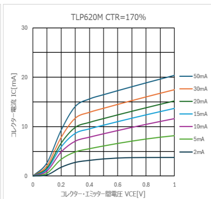
図 4.240 I_C - V_{CE} 特性 (CTR=170%)
