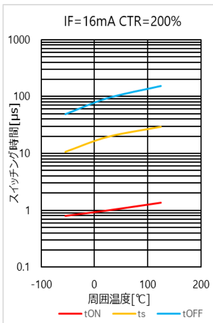
図 4.35 スイッチング時間 - T_a 特性(CTR = 200 %)
