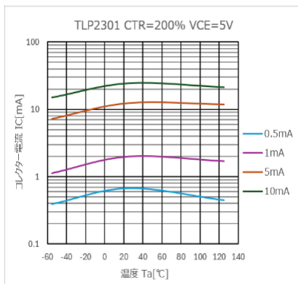
図 4.325 I_C - T_a 特性 (CTR=200%)
