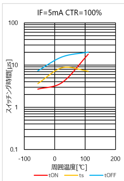
図 4.106 スwitchング時間 - T_a 特性(CTR=100%)
