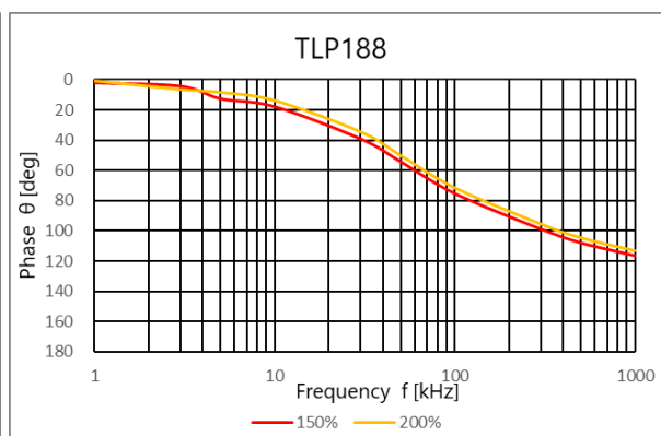
図 4.150 位相 \theta – 周波数
