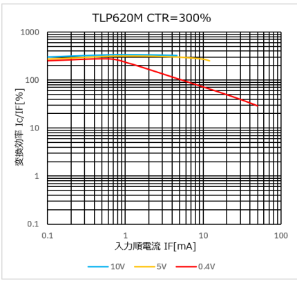
図 4.250 I c /I F – I F 特性 (CTR=300%)
