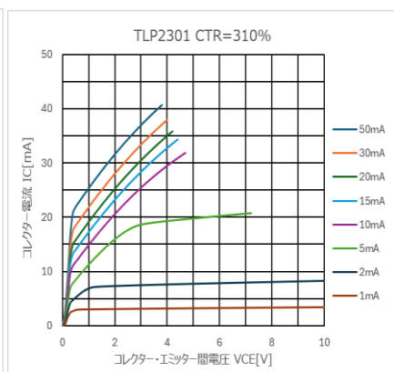
図 4.311 I_C - V_{CE} 特性 (CTR=310%)
