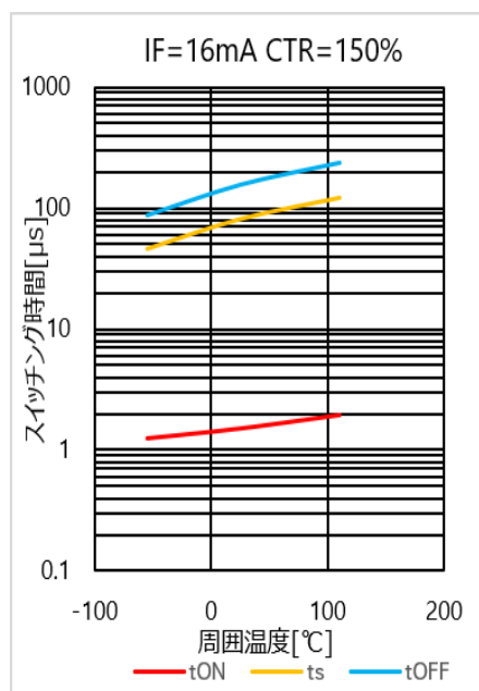
図 4.147 スイッチング時間 – Ta 特性(CTR=150%)
