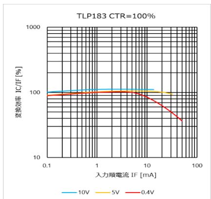
図 4.13 I_C / I_F - I_F 特性 (CTR = 100 %)
