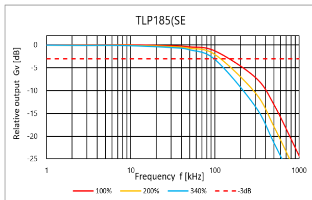
図 4.123 相対出力 G_v - 周波数
