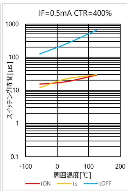
図 4.39 スイッチング時間 - T_a 特性(CTR = 400 %)
