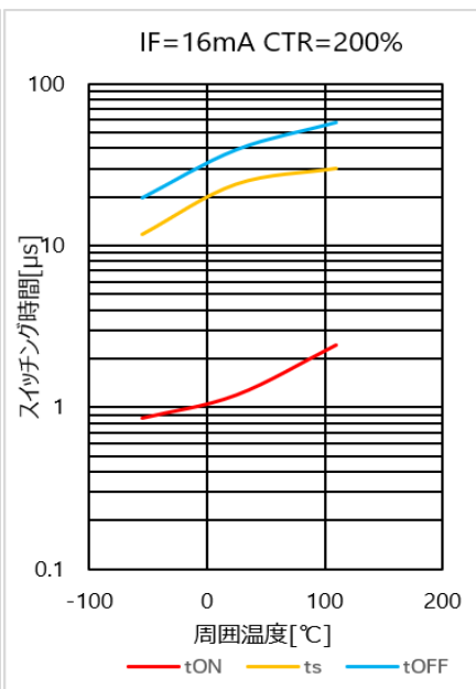
図 4.221 スwitchング時間 - T_a 特性( CTR=200\% )
