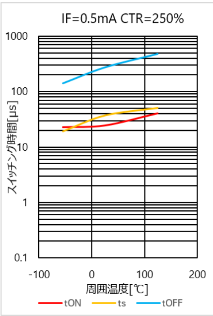
図 4.304 スイッチング時間 – Ta 特性(CTR=250%)
