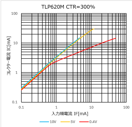
図 4.247 I c – I F 特性 (CTR=300%)
