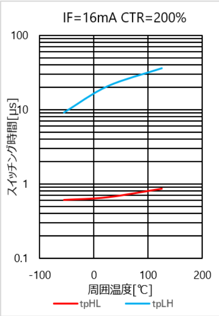
図 4.337 スイッチング時間 - Ta 特性(CTR=200%)
