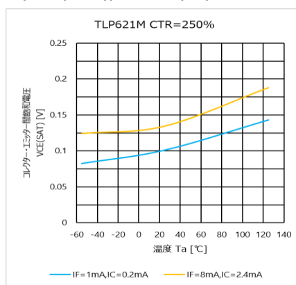
図 4.284 V_{CE} - T_a 特性 (CTR=250%)
