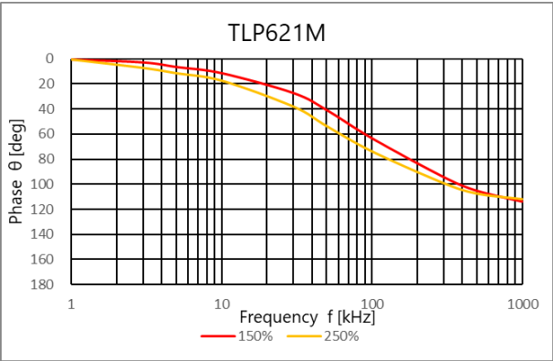
图 4.306 位相 \theta – 周波数
