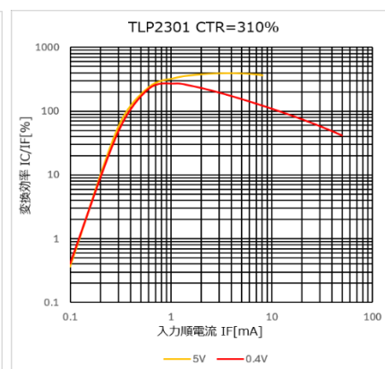
図 4.323 I_C/I_F - I_F 特性 (CTR=310%)
