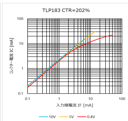
図 4.11 I_C - I_F 特性 (CTR = 202 %)
