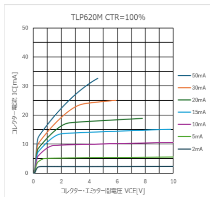
図 4.236 I_C - V_{CE} 特性 (CTR=100%)
