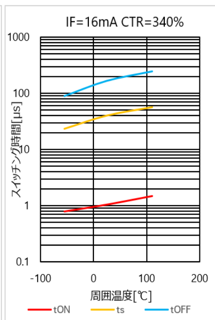
図 4.120 スイッチング時間 - T_a 特性(CTR=340%)
