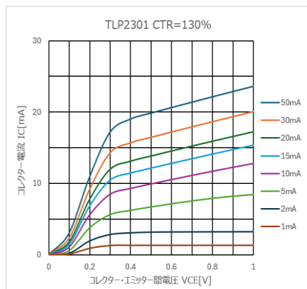
図 4.312 I_C - V_{CE} 特性 (CTR=130%)
