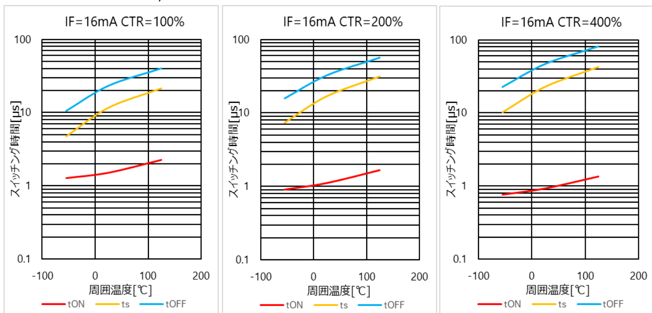
図 4.25 スwitchング時間 - T_a 特性( CTR = 100\% ) 図 4.26 スwitchング時間 - T_a 特性( CTR = 200\% ) 図 4.27 スwitchング時間 - T_a 特性( CTR = 400\% )
