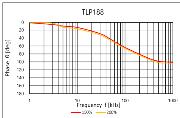
図 4.152 位相 \theta – 周波数
