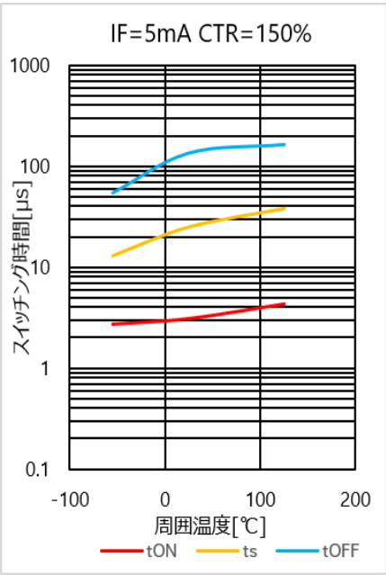
図 4.299 スイッチング時間 – Ta 特性(CTR=150%)
