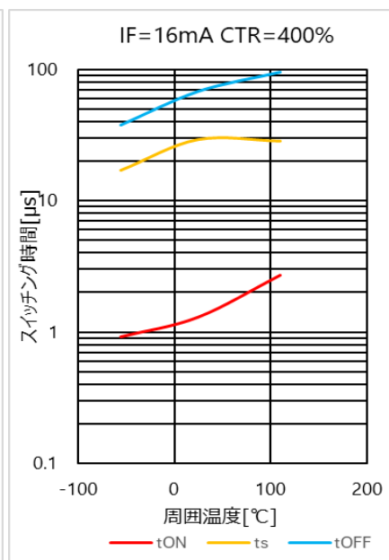
図 4.70 スwitchング時間 - T_a 特性( CTR=400\% )
