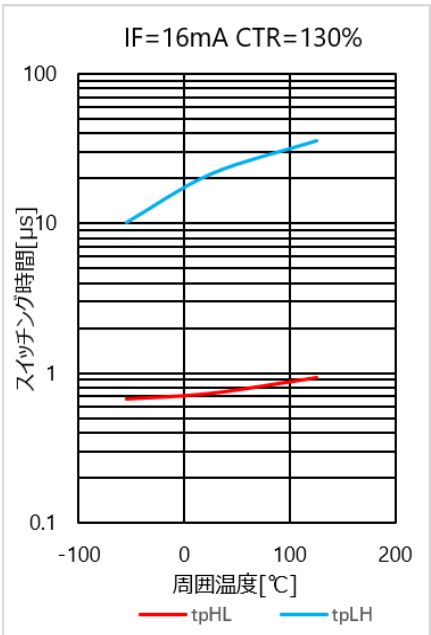
図 4.345 スイッチング時間 - Ta 特性(CTR=130%)
