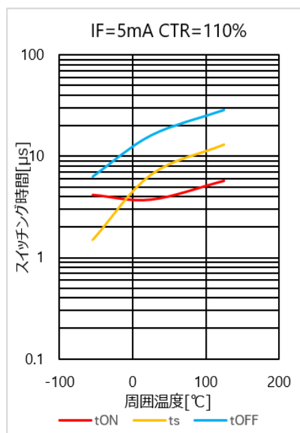
図 4.174 スwitchング時間 - T_a 特性(CTR=110%)
