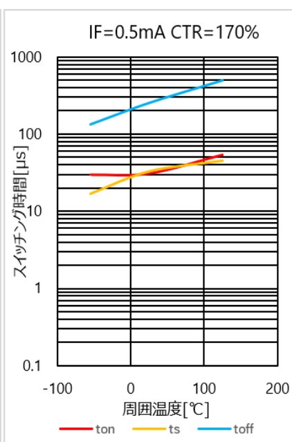
図 4.273 スイッチング時間 - Ta 特性(CTR=170%)
