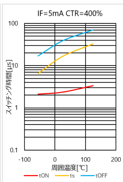
図 4.176 スwitchング時間 - T_a 特性(CTR=400%)
