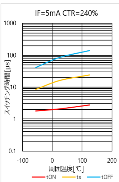
図 4.184 スイッチング時間 - Ta 特性(CTR=240%)
