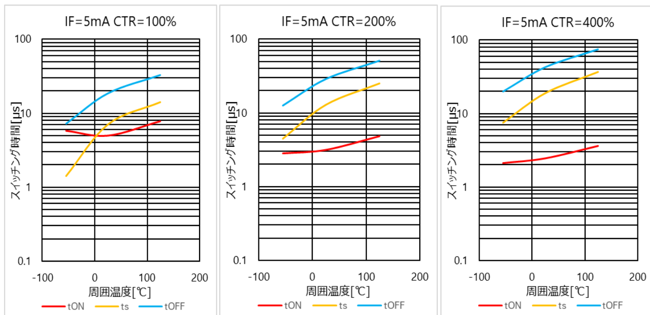
図 4.22 スwitchング時間 - T_a 特性( CTR = 100\% ) 図 4.23 スwitchング時間 - T_a 特性( CTR = 200\% ) 図 4.24 スwitchング時間 - T_a 特性( CTR = 400\% )
