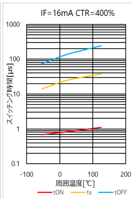
図 4.36 スイッチング時間 - T_a 特性(CTR = 400 %)
