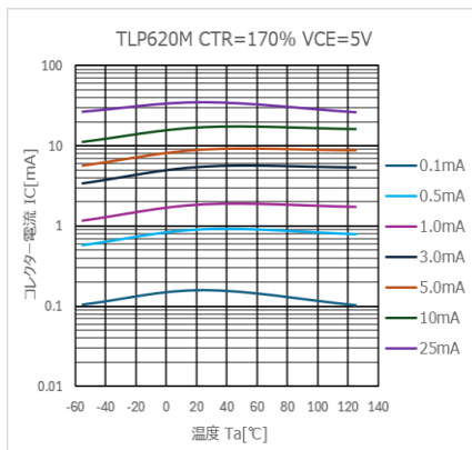
図 4.252 I_C - T_a 特性 (CTR=170%)
