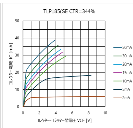
図 4.87 I_C - V_{CE} 特性 (CTR=344%)
