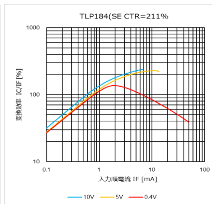
図 4.57 I_C/I_F - I_F 特性 (CTR=211%)
