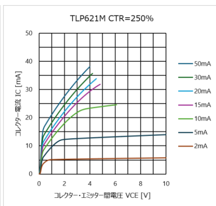
図 4.280 I_C - V_{CE} 特性 (CTR=250%)
