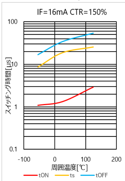
図 4.295 スwitchング時間 - T_a 特性(CTR=150%)
