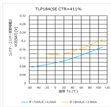
図 4.52 V_{CE} - T_a 特性 (CTR=411%)
