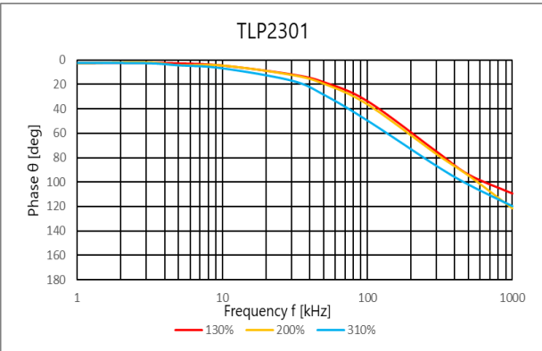
图 4.351 位相 \theta – 周波数
