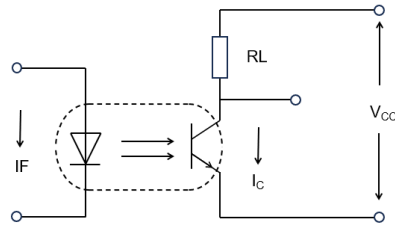
図 2.7 トランジスターカプラー
