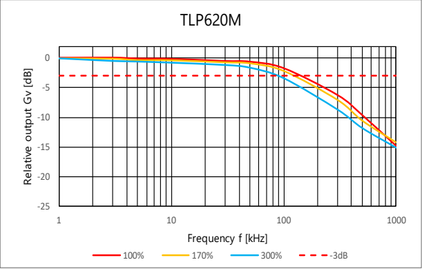
图 4.277 相对出力 Gv – 周波数
