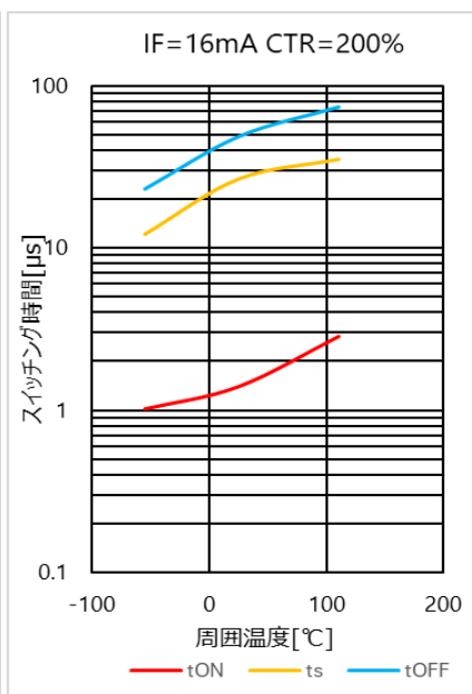
図 4.69 スwitchング時間 - T_a 特性( CTR=200\% )
