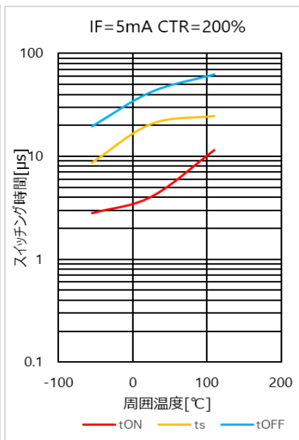
図 4.66 スwitchング時間 - T_a 特性( CTR=200\% )
