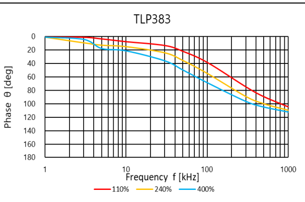
图 4.195 位相 \theta – 周波数
