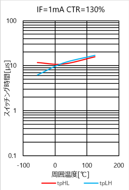
図 4.339 スイッチング時間 - Ta 特性(CTR=130%)
