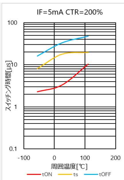
図 4.218 スwitchング時間 - T_a 特性( CTR=200\% )
