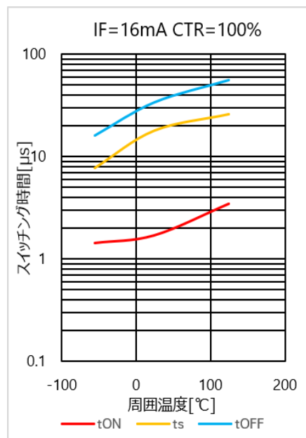
図 4.260 スwitchング時間 - T_a 特性(CTR=100%)
