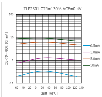
図 4.327 I_C - T_a 特性 (CTR=130%)
