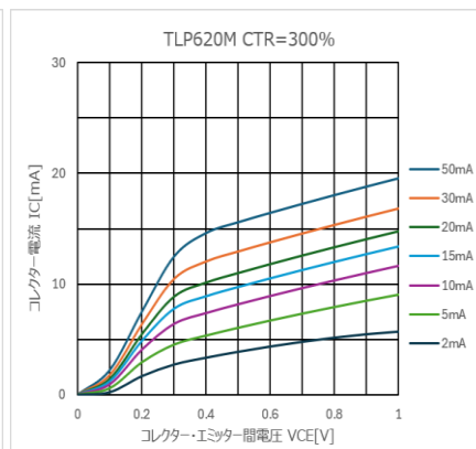
図 4.241 I_C - V_{CE} 特性 (CTR=300%)
