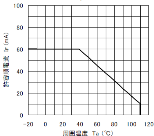
図 2.13 周囲温度-許容順電流例
