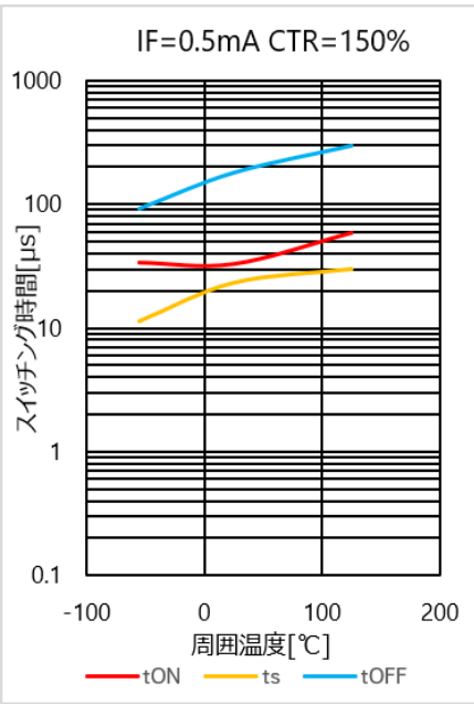
図 4.303 スイッチング時間 – Ta 特性(CTR=150%)
