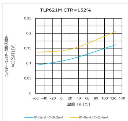
図 4.283 V_{CE} - T_a 特性 (CTR=152%)
