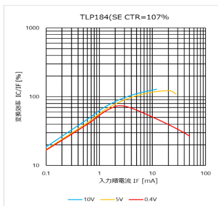
図 4.56 I_C/I_F - I_F 特性 (CTR=107%)
