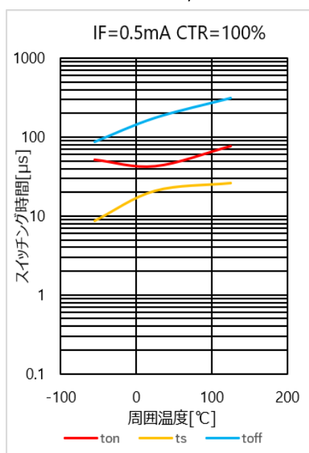
図 4.272 スイッチング時間 - Ta 特性(CTR=100%)
