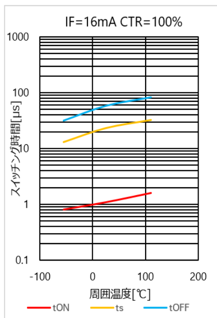
図 4.118 スイッチング時間 - T_a 特性(CTR=100%)
