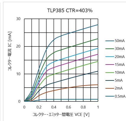
図 4.201 I_C - V_{CE} 特性 (CTR=403%)
