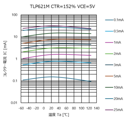
図 4.289 I_C - T_a 特性 (CTR=152%)
