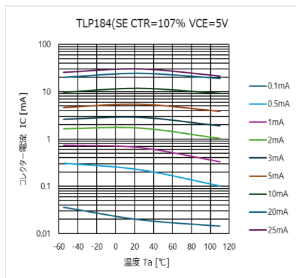
図 4.59 I_C – T_a 特性 (CTR=107%)
