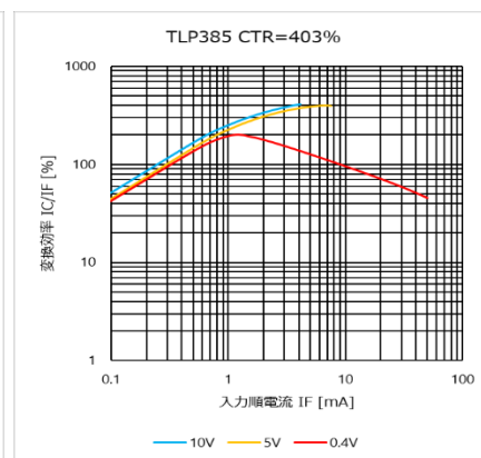
図 4.210 I_C/I_F - I_F 特性 (CTR=403%)
