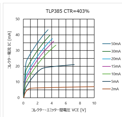
図 4.198 I_C - V_{CE} 特性 (CTR=403%)
