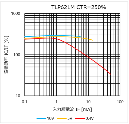
図 4.288 I C /I F – I F 特性 (CTR=250%)
