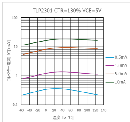
図 4.324 I_C - T_a 特性 (CTR=130%)
