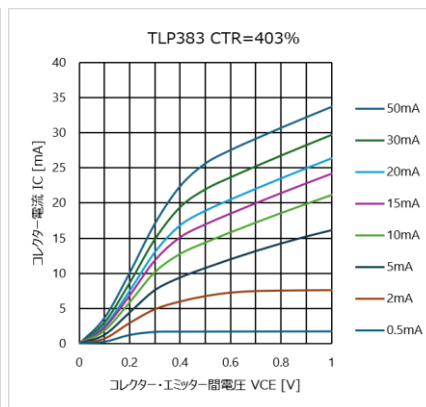
図 4.158 I_C - V_{CE} 特性 (CTR=403%)
