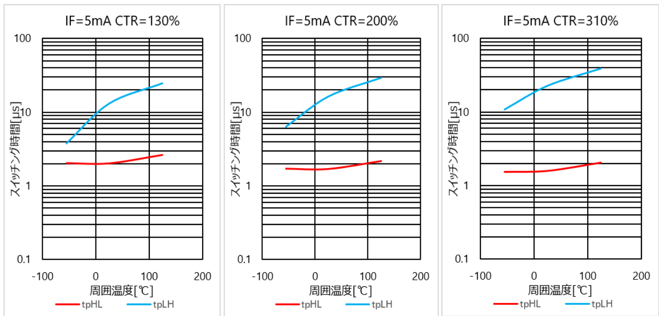
図 4.333 スwitchング時間 - Ta 特性(CTR=130%)
