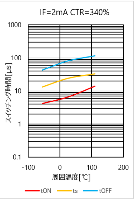
図 4.114 スイッチング時間 – Ta 特性(CTR=340%)
