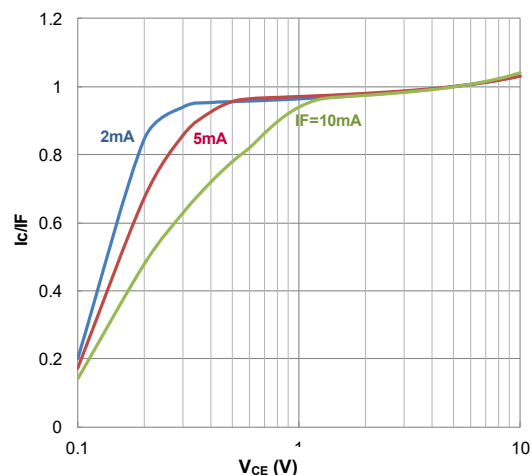
図 2.21 I_C/I_F - V_{CE} 特性
