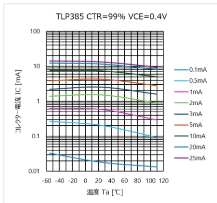
図 4.214 I_C - T_a 特性 (CTR=99%)
