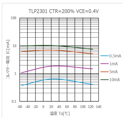
図 4.328 I_C - T_a 特性 (CTR=200%)
