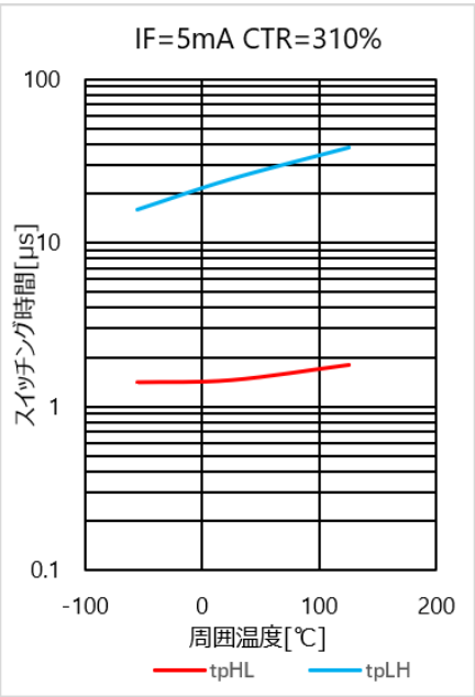
図 4.344 スイッチング時間 - Ta 特性(CTR=310%)
