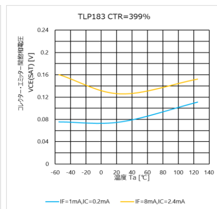
図 4.9 V_{CE} - T_a 特性 (CTR = 399 %)
