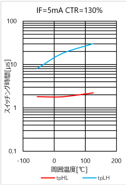
図 4.342 スイッチング時間 - Ta 特性(CTR=130%)
