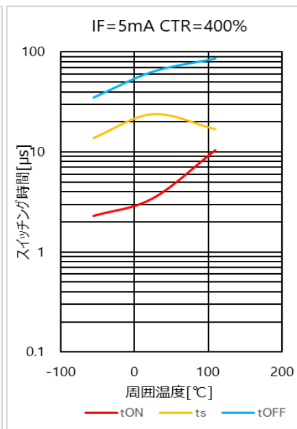
図 4.67 スwitchング時間 - T_a 特性( CTR=400\% )
