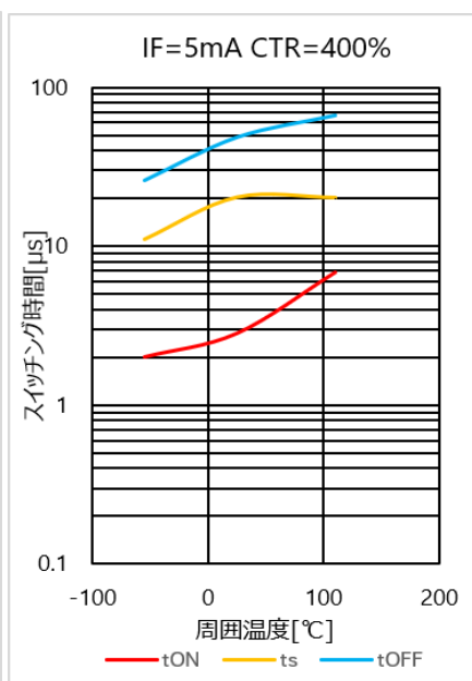
図 4.219 スwitchング時間 - T_a 特性( CTR=400\% )
