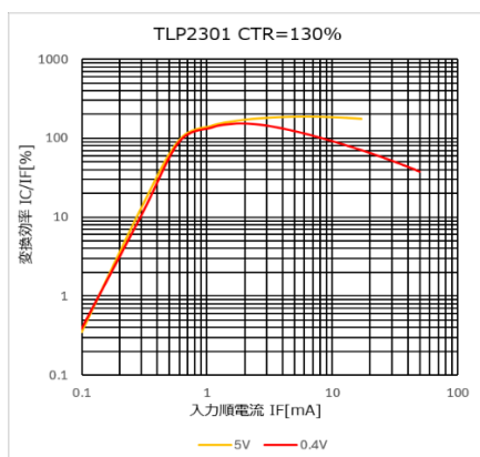
図 4.321 I_C/I_F - I_F 特性 (CTR=130%)
