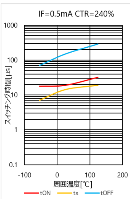
図 4.190 スイッチング時間 – Ta 特性(CTR=240%)
