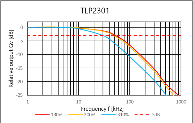
图 4.348 相对出力 G_v – 周波数
