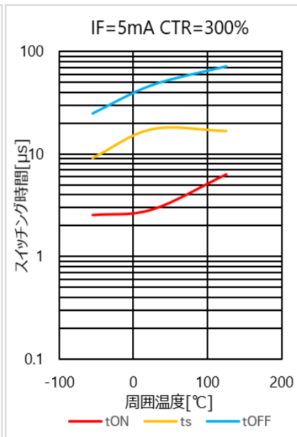
図 4.259 スwitchング時間 - T_a 特性(CTR=300%)
