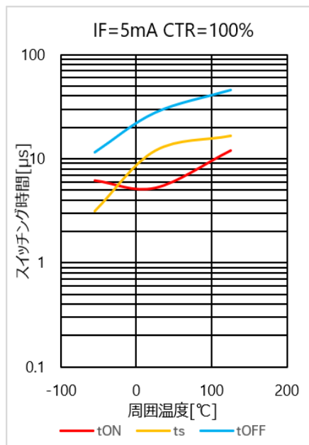
図 4.257 スwitchング時間 - T_a 特性(CTR=100%)
