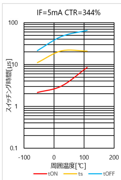
図 4.108 スwitchング時間 - T_a 特性(CTR=344%)
