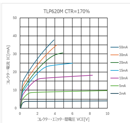
図 4.237 I_C - V_{CE} 特性 (CTR=170%)
