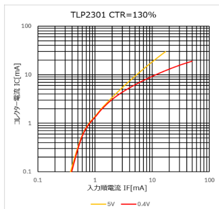
図 4.318 I_C - I_F 特性 (CTR=130%)
