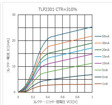
図 4.314 I_C - V_{CE} 特性 (CTR=310%)
