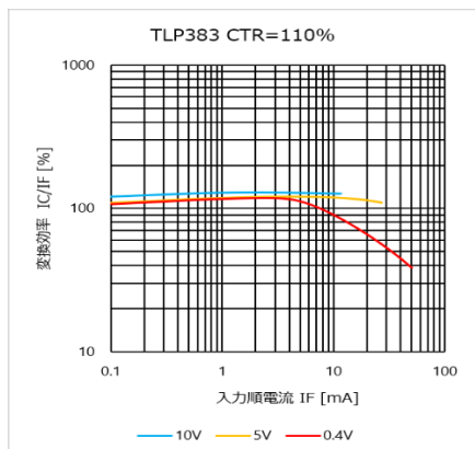
図 4.165 I_C/I_F - I_F 特性 (CTR=110%)
