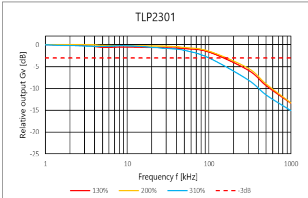
图 4.350 相对出力 G_v – 周波数
