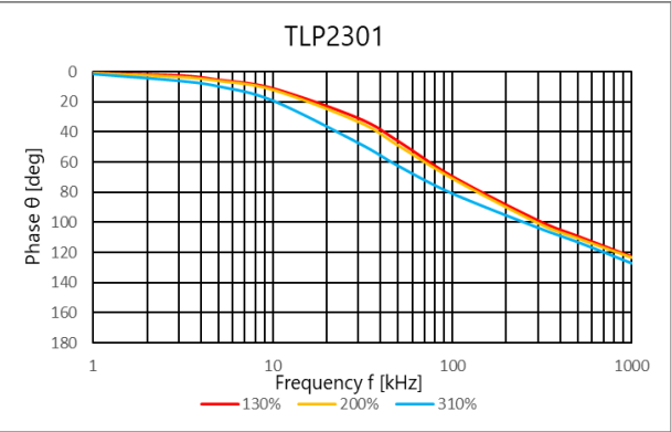
图 4.349 位相 \theta – 周波数
