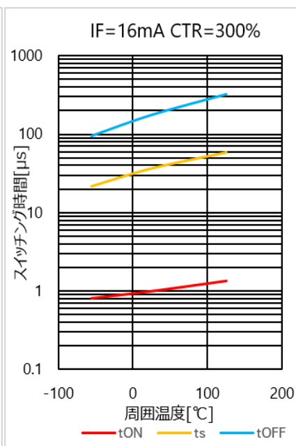
図 4.271 スイッチング時間 - Ta 特性(CTR=300%)
