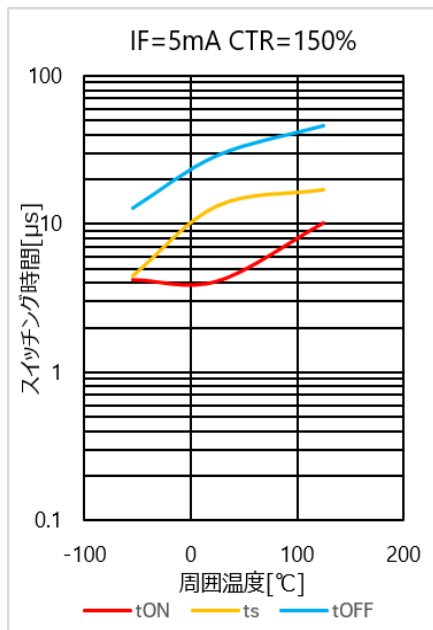
図 4.293 スwitchング時間 - T_a 特性(CTR=150%)
