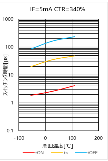
図 4.117 スイッチング時間 – Ta 特性(CTR=340%)
