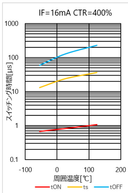
図 4.188 スイッチング時間 – Ta 特性(CTR=400%)
