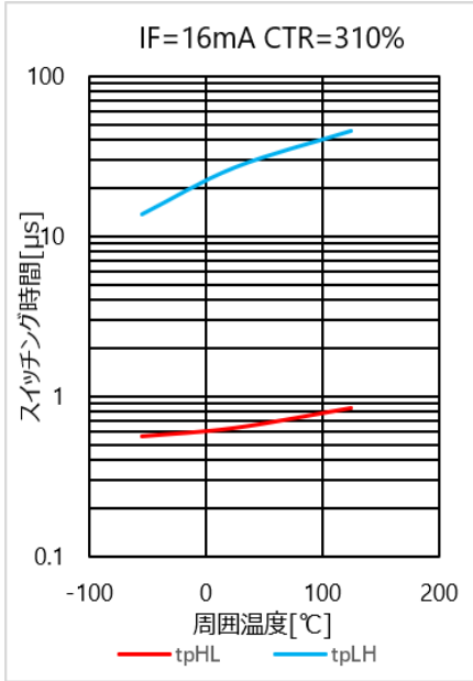
図 4.338 スイッチング時間 - Ta 特性(CTR=310%)
