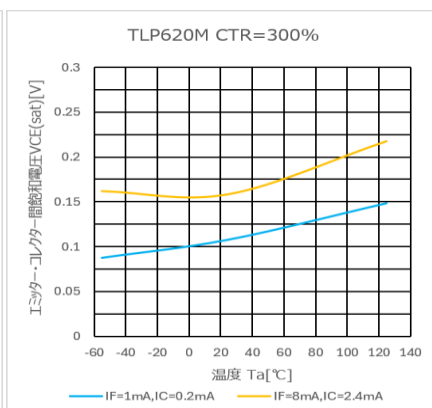
図 4.244 V_{CE} - T_a 特性 (CTR=300%)
