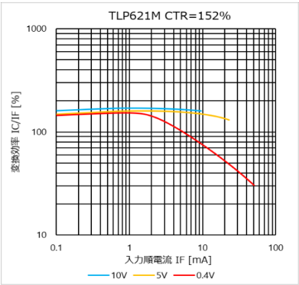
図 4.287 I C /I F – I F 特性 (CTR=152%)
