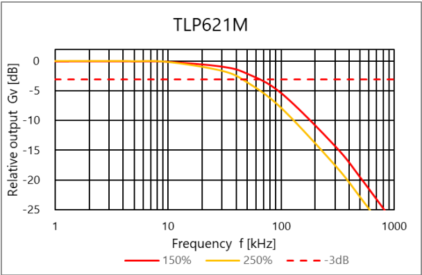
图 4.305 相对出力 G_v – 周波数
