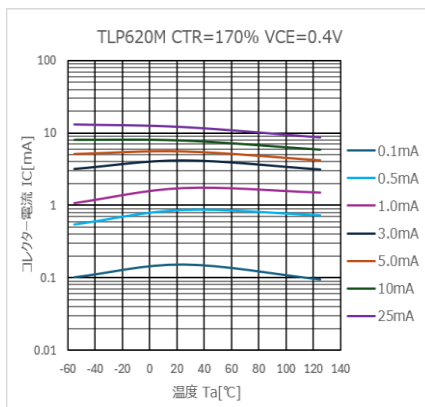
図 4.255 I_C - T_a 特性 (CTR=170%)
