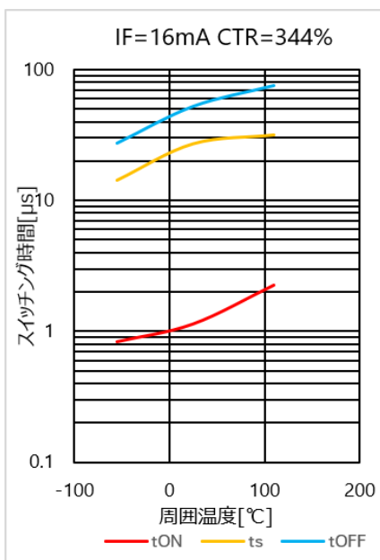
図 4.111 スwitchング時間 - T_a 特性(CTR=344%)
