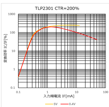
図 4.322 I_C/I_F - I_F 特性 (CTR=200%)
