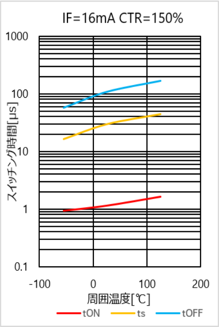
図 4.301 スイッチング時間 – Ta 特性(CTR=150%)
