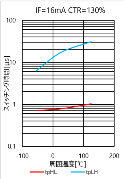
図 4.336 スイッチング時間 - Ta 特性(CTR=130%)
