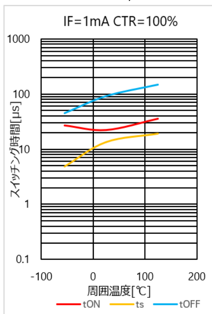
図 4.263 スイッチング時間 - Ta 特性(CTR=100%)
