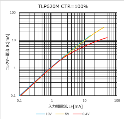
図 4.245 I c – I F 特性 (CTR=100%)
