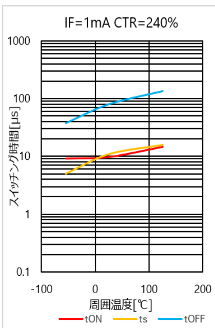
図 4.181 スイッチング時間 - Ta 特性(CTR=240%)
