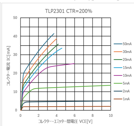
図 4.310 I_C - V_{CE} 特性 (CTR=200%)
