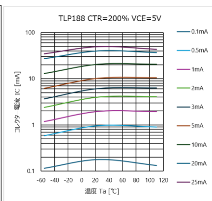
図 4.136 I_C - T_a 特性 (CTR=200%)
