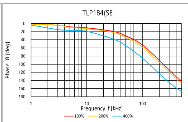
図 4.84 位相 \theta - 周波数
