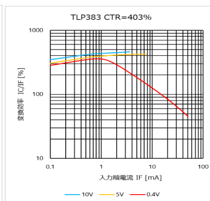
図 4.167 I_C/I_F - I_F 特性 (CTR=403%)
