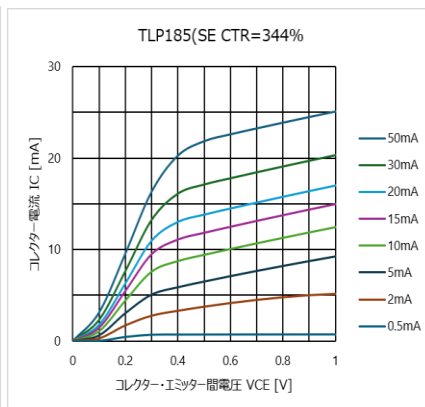
図 4.90 I_C - V_{CE} 特性 (CTR=344%)
