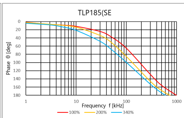
図 4.122 位相 \theta - 周波数
