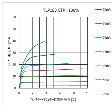
図 4.1 I_C - V_{CE} 特性 (CTR = 100 %)
