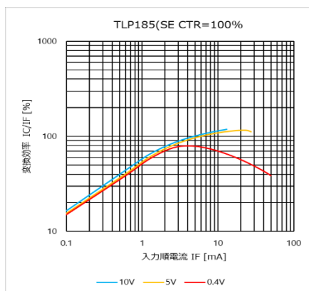
図 4.97 I_C/I_F - I_F 特性 (CTR=100%)
