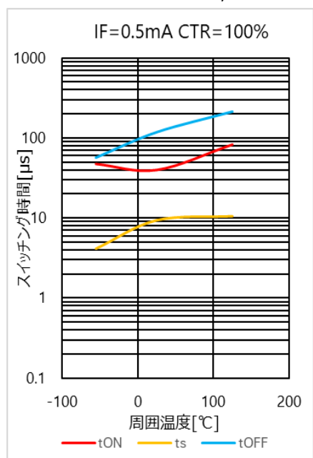
図 4.37 スイッチング時間 - T_a 特性(CTR = 100 %)
