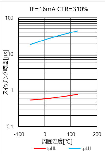
図 4.347 スイッチング時間 - Ta 特性(CTR=310%)
