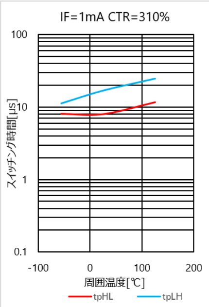
図 4.341 スイッチング時間 - Ta 特性(CTR=310%)
