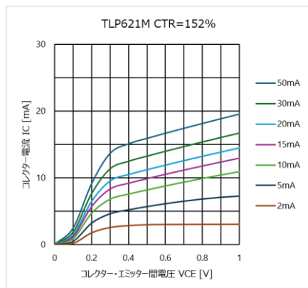
図 4.281 I_C - V_{CE} 特性 (CTR=152%)
