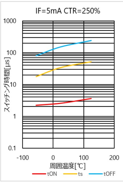
図 4.300 スイッチング時間 – Ta 特性(CTR=250%)
