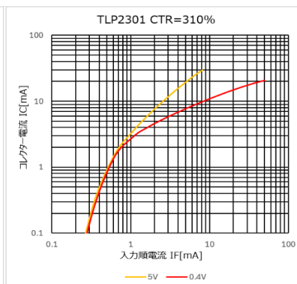
図 4.320 I_C - I_F 特性 (CTR=310%)
