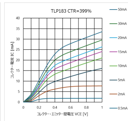
図 4.6 I_C - V_{CE} 特性 (CTR = 399 %)
