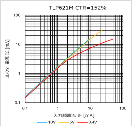
図 4.285 I C – I F 特性 (CTR=152%)
