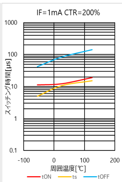
図 4.29 スイッチング時間 - T_a 特性(CTR = 200 %)
