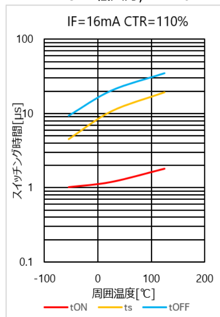
図 4.177 スwitchング時間 - T_a 特性(CTR=110%)
