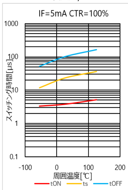
図 4.266 スイッチング時間 - Ta 特性(CTR=100%)
