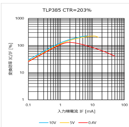
図 4.209 I_C/I_F - I_F 特性 (CTR=203%)
