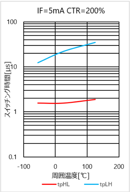
図 4.343 スイッチング時間 - Ta 特性(CTR=200%)
