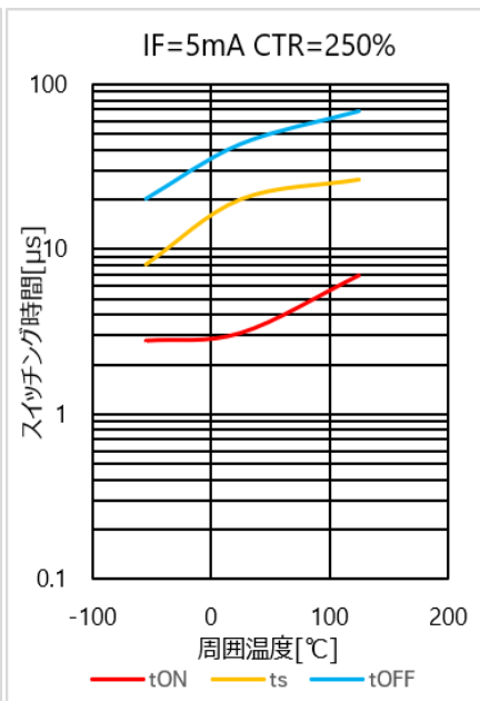
図 4.294 スwitchング時間 - T_a 特性(CTR=250%)
