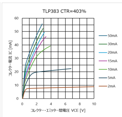
図 4.155 I_C - V_{CE} 特性 (CTR=403%)
