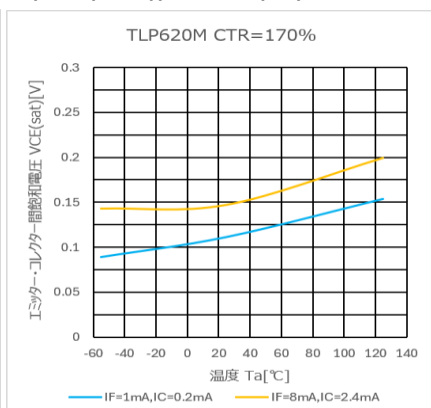
図 4.243 V_{CE} - T_a 特性 (CTR=170%)
