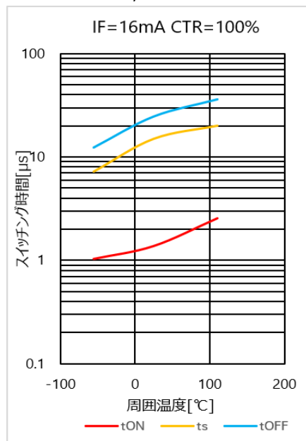
図 4.220 スwitchング時間 - T_a 特性( CTR=100\% )
