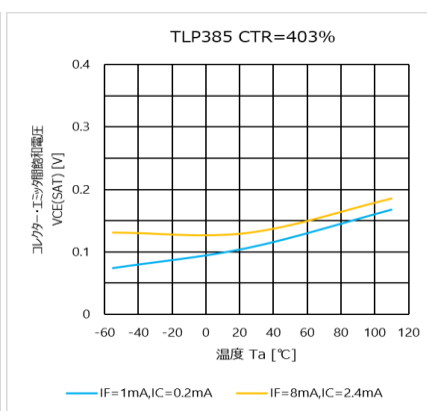
図 4.204 V_{CE} - T_a 特性 (CTR=403%)
