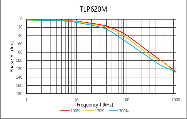
图 4.278 位相 θ – 周波数
