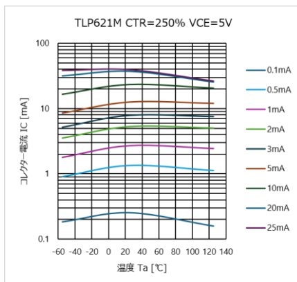
図 4.290 I_C - T_a 特性 (CTR=250%)
