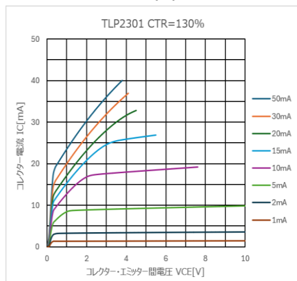
図 4.309 I_C - V_{CE} 特性 (CTR=130%)
