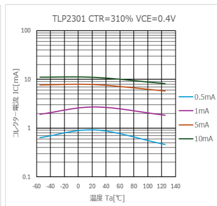
図 4.329 I_C - T_a 特性 (CTR=310%)
