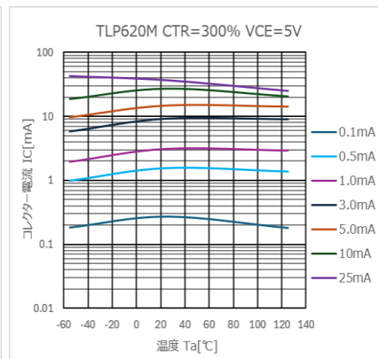
図 4.253 I_C - T_a 特性 (CTR=300%)
