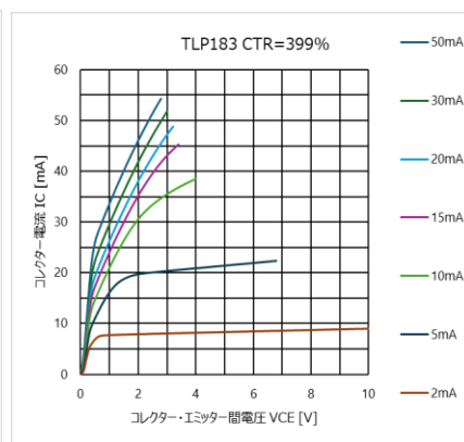
図 4.3 I_C - V_{CE} 特性 (CTR = 399 %)
