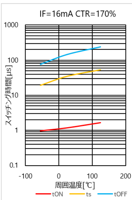
図 4.270 スイッチング時間 - Ta 特性(CTR=170%)
