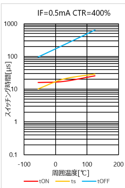
図 4.191 スイッチング時間 – Ta 特性(CTR=400%)
