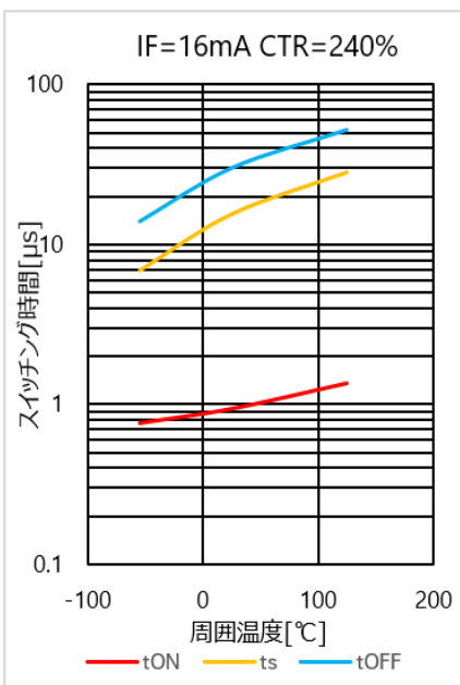
図 4.178 スwitchング時間 - T_a 特性(CTR=240%)
