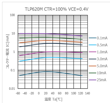
図 4.254 I_C - T_a 特性 (CTR=100%)
