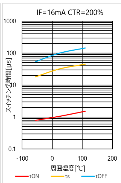
図 4.119 スイッチング時間 - T_a 特性(CTR=200%)
