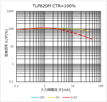
図 4.248 I c /I F – I F 特性 (CTR=100%)
