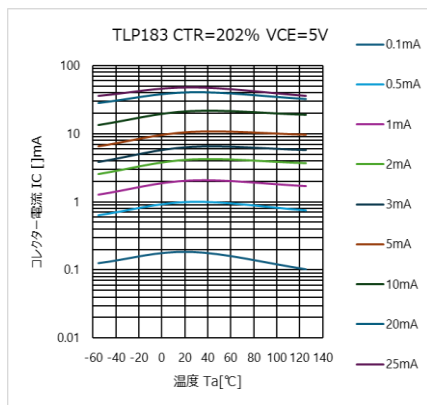
図 4.17 I_C - T_a 特性 (CTR = 202 %)
