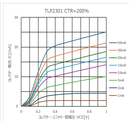
図 4.313 I_C - V_{CE} 特性 (CTR=200%)
