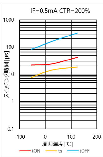
図 4.38 スイッチング時間 - T_a 特性(CTR = 200 %)
