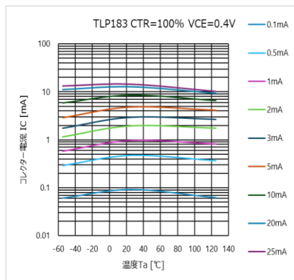
図 4.19 I_C - T_a 特性 (CTR = 100 %)
