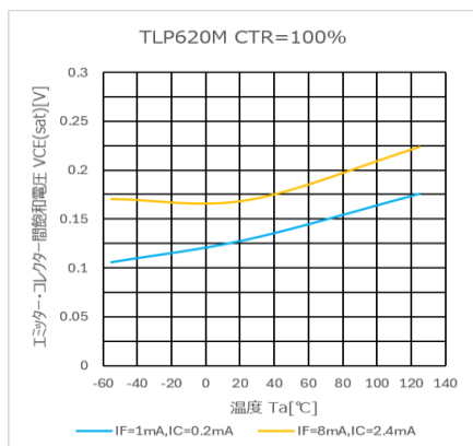
図 4.242 V_{CE} - T_a 特性 (CTR=100%)
