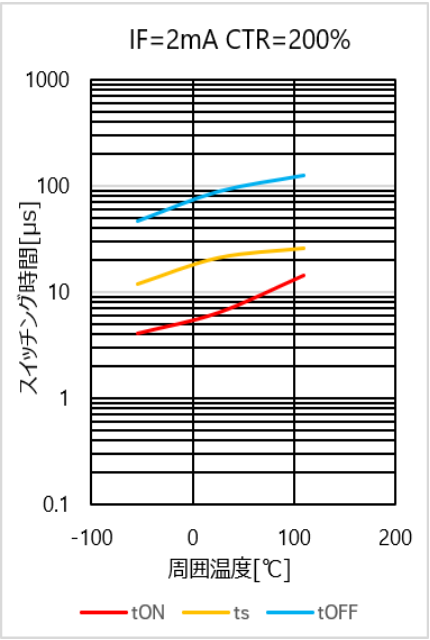
図 4.113 スイッチング時間 – Ta 特性(CTR=200%)
