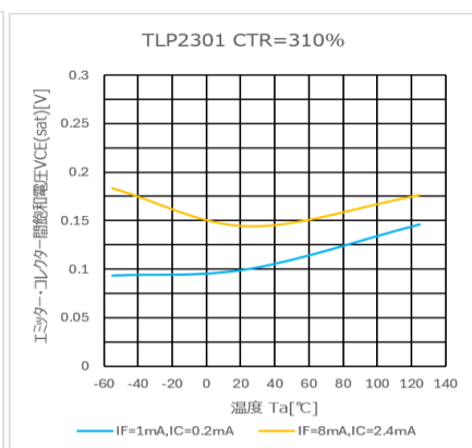
図 4.317 V_{CE} - T_a 特性 (CTR=310%)
