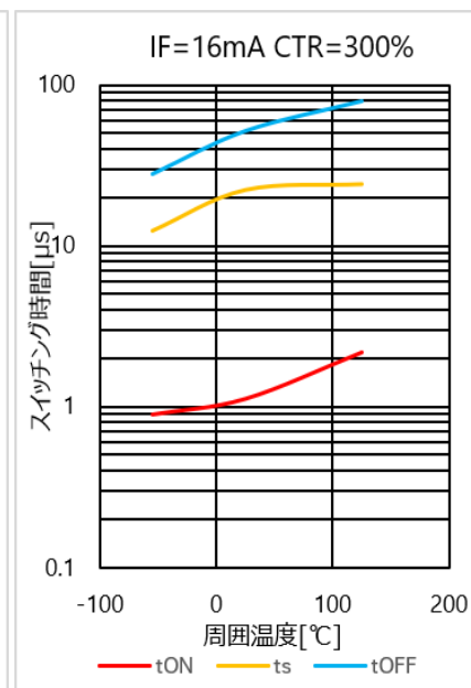
図 4.262 スwitchング時間 - T_a 特性(CTR=300%)
