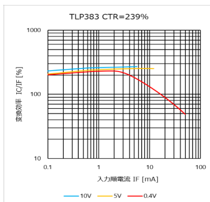
図 4.166 I_C/I_F - I_F 特性 (CTR=239%)
