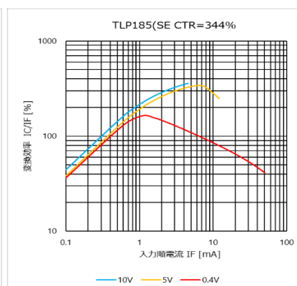
図 4.99 I_C/I_F - I_F 特性 (CTR=344%)
