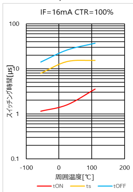
図 4.68 スwitchング時間 - T_a 特性( CTR=100\% )
