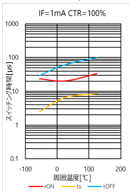
図 4.28 スイッチング時間 - T_a 特性(CTR = 100 %)
