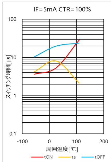
図 4.65 スwitchング時間 - T_a 特性( CTR=100\% )
