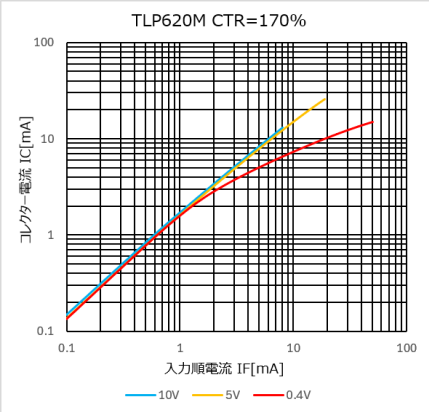
図 4.246 I c – I F 特性 (CTR=170%)
