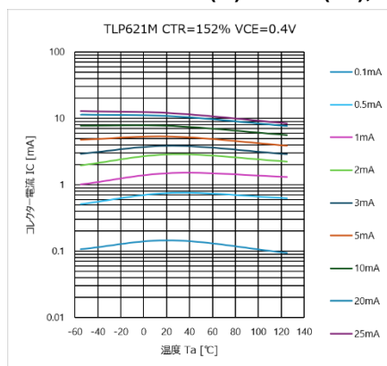
図 4.291 I_C - T_a 特性 (CTR=152%)
