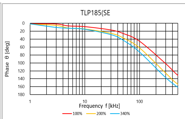
図 4.124 位相 \theta - 周波数
