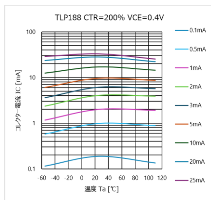
図 4.138 I_C - T_a 特性 (CTR=200%)
