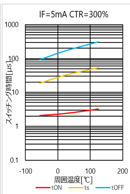
図 4.268 スイッチング時間 - Ta 特性(CTR=300%)
