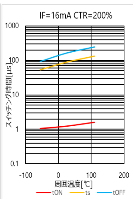
図 4.148 スイッチング時間 – Ta 特性(CTR=200%)
