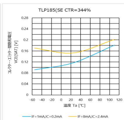
図 4.93 V_{CE} - T_a 特性 (CTR=344%)
