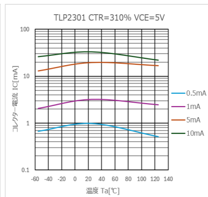
図 4.326 I_C - T_a 特性 (CTR=310%)
