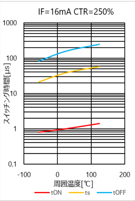
図 4.302 スイッチング時間 – Ta 特性(CTR=250%)
