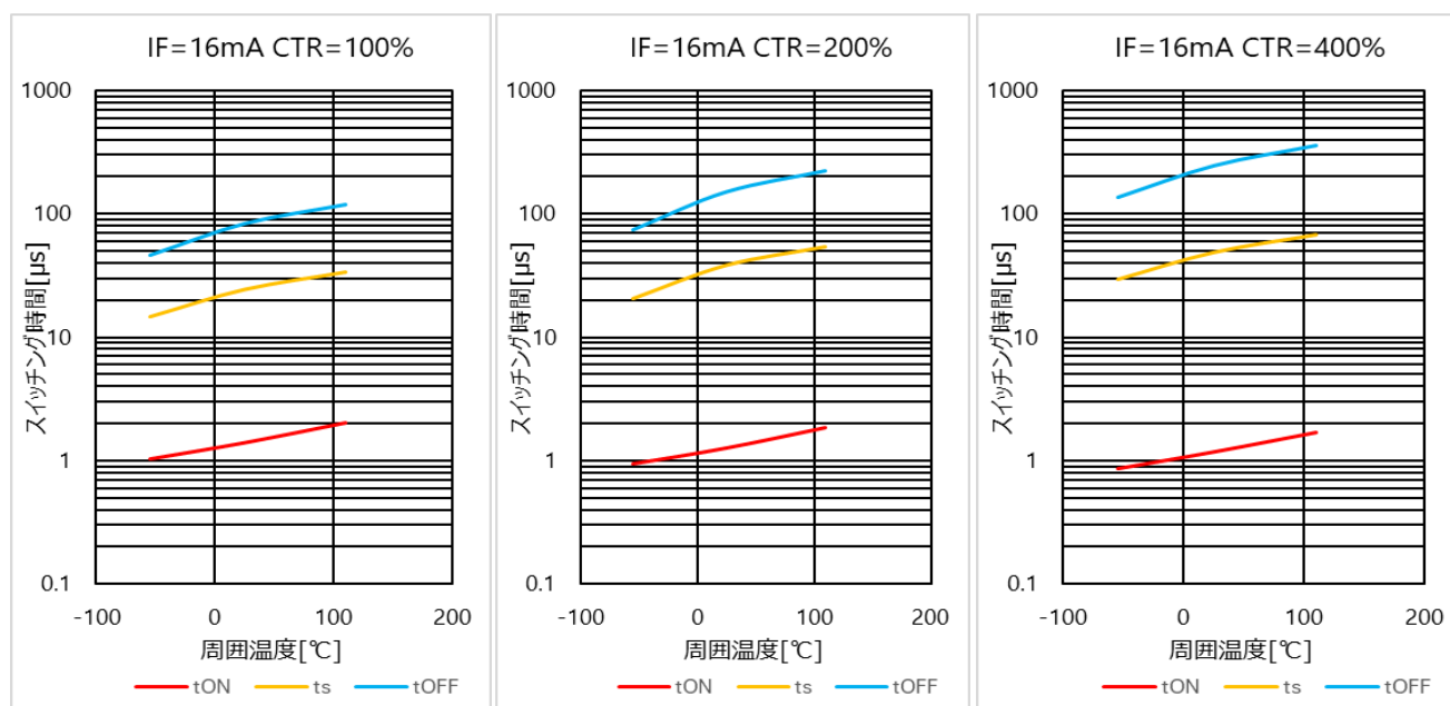
図 4.78 スウィッチング時間 - T_a 特性(CTR=100%) 図 4.79 スウィッチング時間 - T_a 特性(CTR=200%) 図 4.80 スウィッチング時間 - T_a 特性(CTR=400%)
