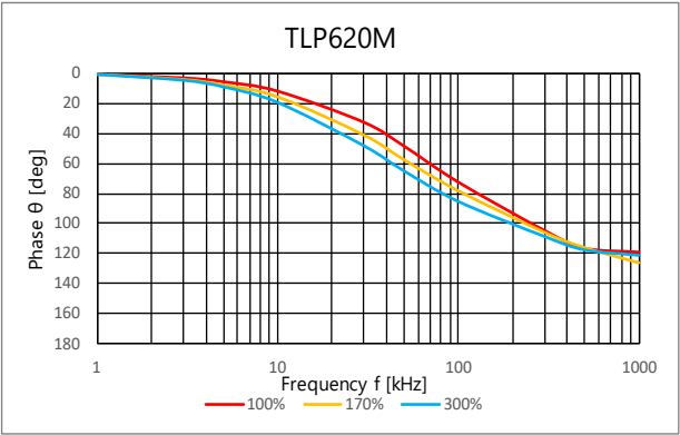
图 4.276 位相 θ – 周波数
