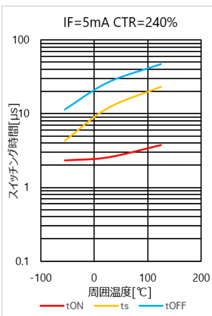
図 4.175 スwitchング時間 - T_a 特性(CTR=240%)
