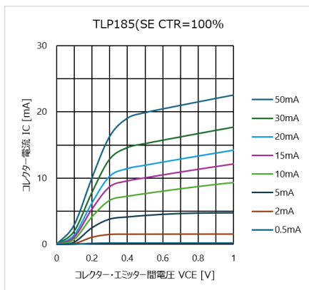
図 4.88 I_C - V_{CE} 特性 (CTR=100%)
