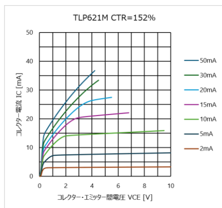
図 4.279 I_C - V_{CE} 特性 (CTR=152%)
