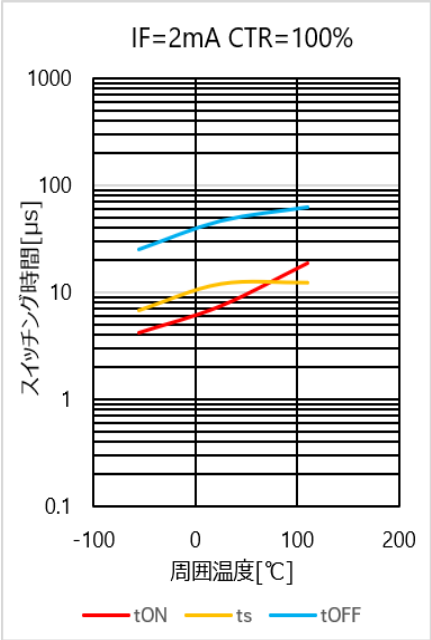
図 4.112 スイッチング時間 – Ta 特性(CTR=100%)
