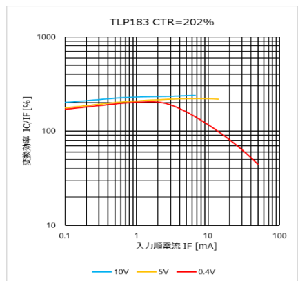
図 4.14 I_C / I_F - I_F 特性 (CTR = 202 %)
