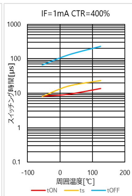
図 4.30 スイッチング時間 - T_a 特性(CTR = 400 %)
