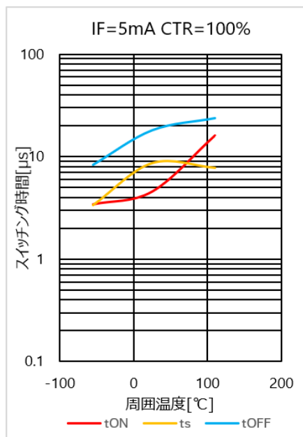
図 4.217 スwitchング時間 - T_a 特性( CTR=100\% )
