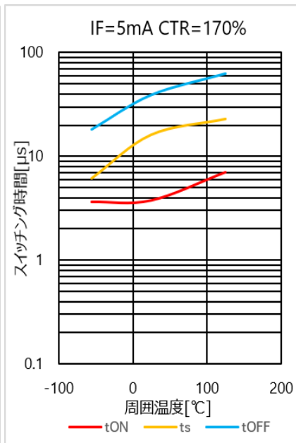
図 4.258 スwitchング時間 - T_a 特性(CTR=170%)
