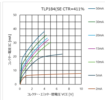
図 4.46 I_C - V_{CE} 特性 (CTR=411%)
