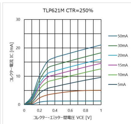
図 4.282 I_C - V_{CE} 特性 (CTR=250%)
