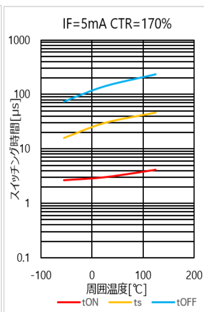
図 4.267 スイッチング時間 - Ta 特性(CTR=170%)
