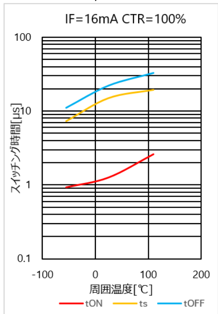
図 4.109 スwitchング時間 - T_a 特性(CTR=100%)
