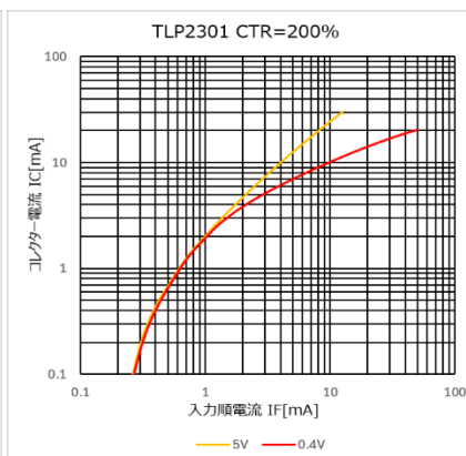
図 4.319 I_C - I_F 特性 (CTR=200%)
