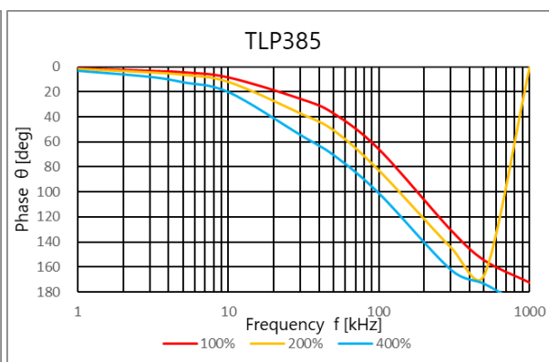
図 4.233 位相 \theta - 周波数
