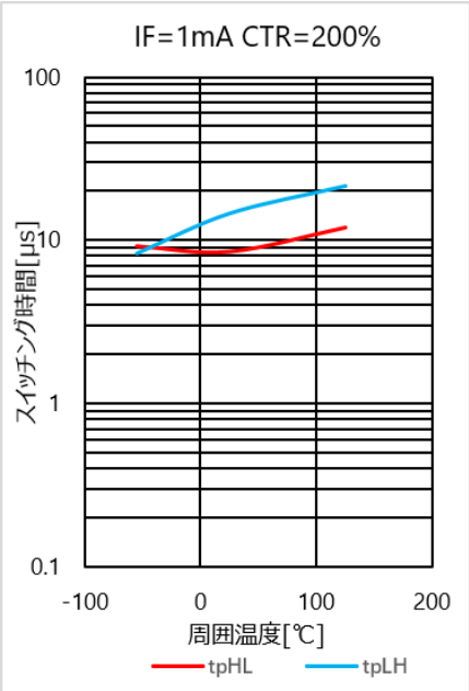
図 4.340 スイッチング時間 - Ta 特性(CTR=200%)
