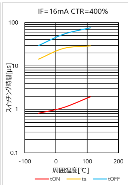
図 4.222 スwitchング時間 - T_a 特性( CTR=400\% )
