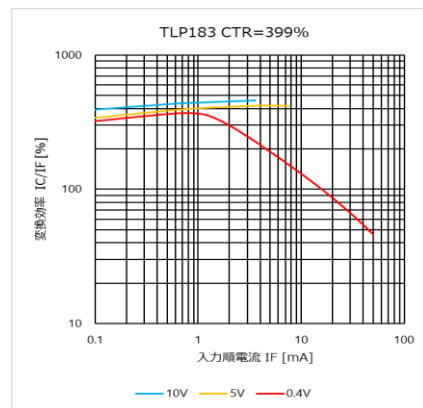
図 4.15 I_C / I_F - I_F 特性 (CTR = 399 %)
