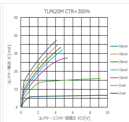
図 4.238 I_C - V_{CE} 特性 (CTR=300%)
