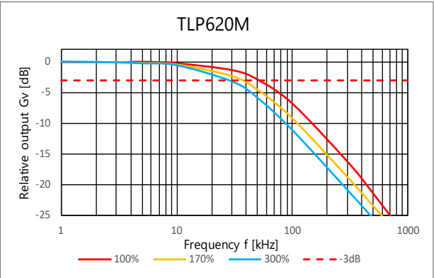
图 4.275 相对出力 Gv – 周波数
