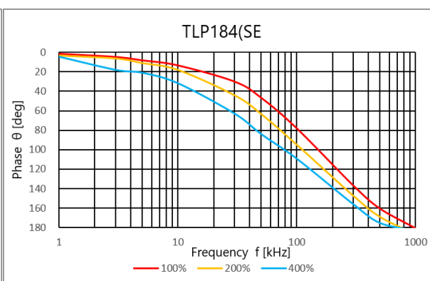
図 4.82 位相 \theta - 周波数
