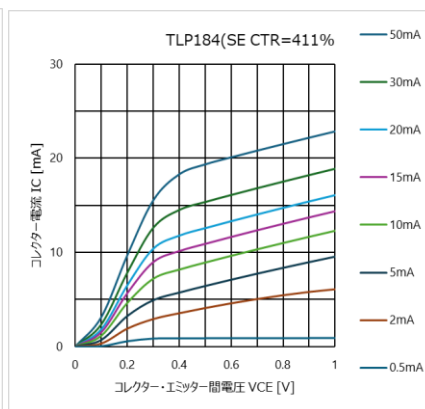
図 4.49 I_C - V_{CE} 特性 (CTR=411%)
