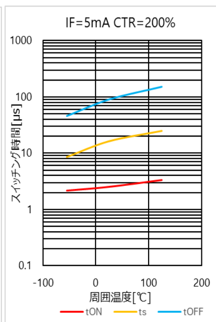
図 4.32 スイッチング時間 - T_a 特性(CTR = 200 %)
