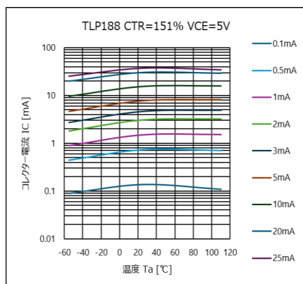
図 4.135 I_C - T_a 特性 (CTR=151%)
