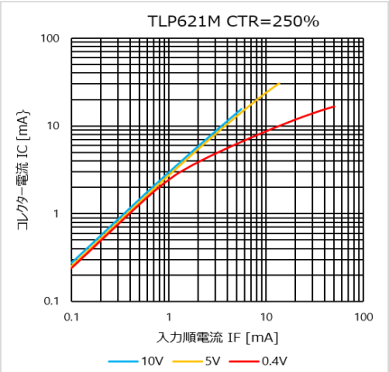
図 4.286 I C – I F 特性 (CTR=250%)
