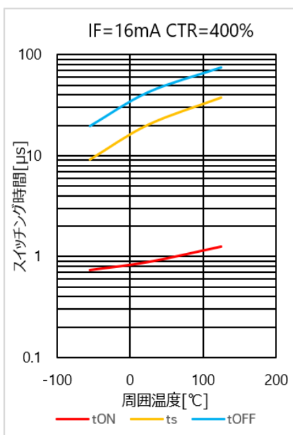
図 4.179 スwitchング時間 - T_a 特性(CTR=400%)
