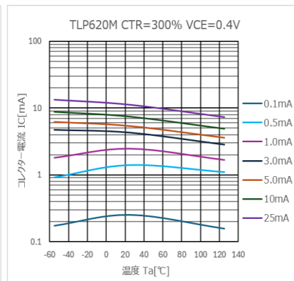
図 4.256 I_C - T_a 特性 (CTR=300%)
