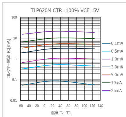
図 4.251 I_C - T_a 特性 (CTR=100%)
