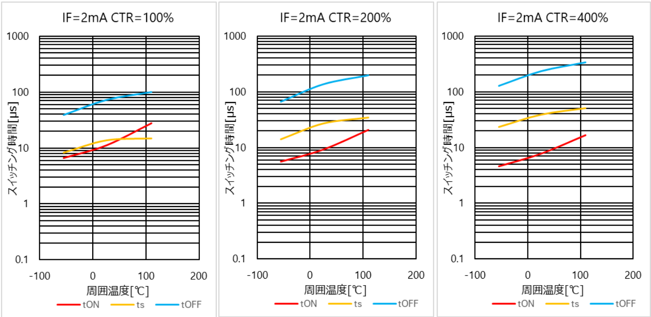
図 4.71 スイッチング時間 - Ta 特性(CTR=100%) 図 4.72 スイッチング時間 - Ta 特性(CTR=200%) 図 4.73 スイッチング時間 - Ta 特性(CTR=400%)
