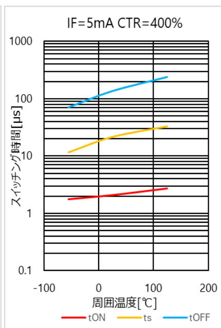
図 4.33 スイッチング時間 - T_a 特性(CTR = 400 %)
