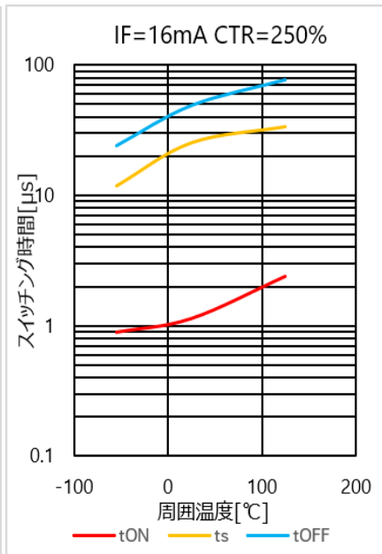
図 4.296 スwitchング時間 - T_a 特性(CTR=250%)
