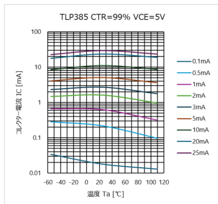
図 4.211 I_C - T_a 特性 (CTR=99%)
