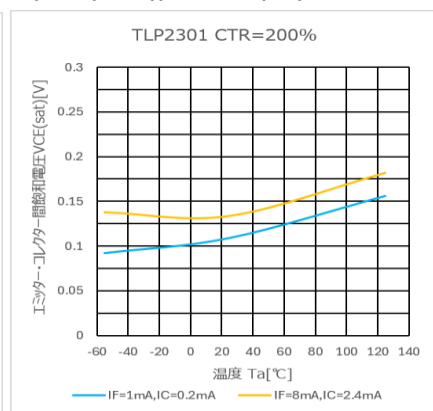
図 4.316 V_{CE} - T_a 特性 (CTR=200%)
