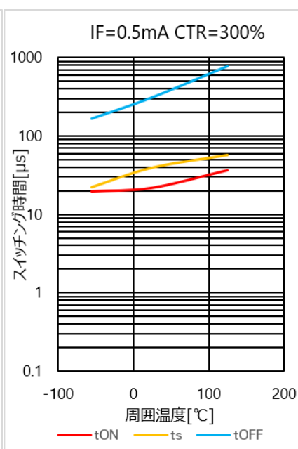
図 4.274 スイッチング時間 - Ta 特性(CTR=300%)
