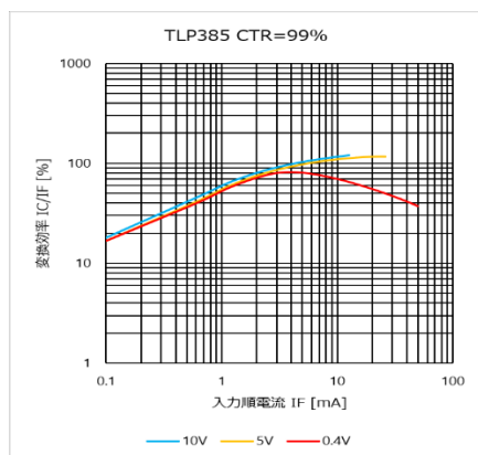
図 4.208 I_C/I_F - I_F 特性 (CTR=99%)
