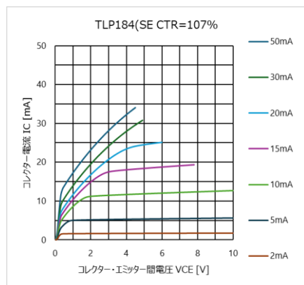
図 4.44 I_C - V_{CE} 特性 (CTR=107%)
