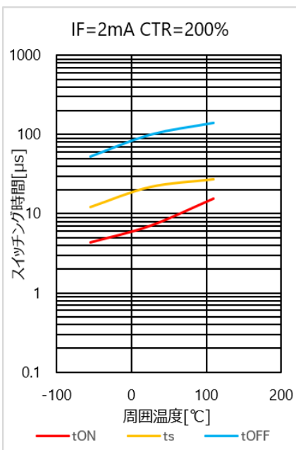
図 4.224 スイッチング時間 - Ta 特性(CTR=200%)
