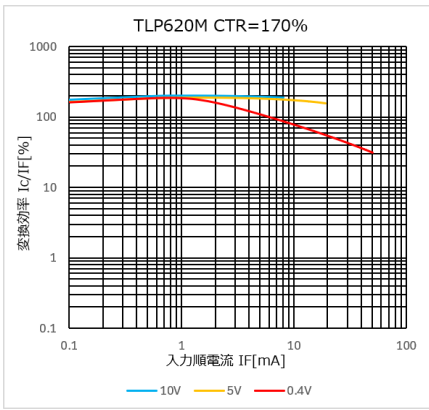
図 4.249 I c /I F – I F 特性 (CTR=170%)
