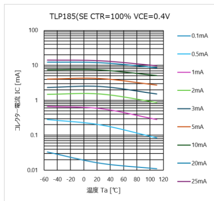
図 4.103 I_C - T_a 特性 (CTR=100%)
