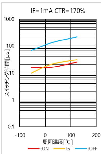
図 4.264 スイッチング時間 - Ta 特性(CTR=170%)
