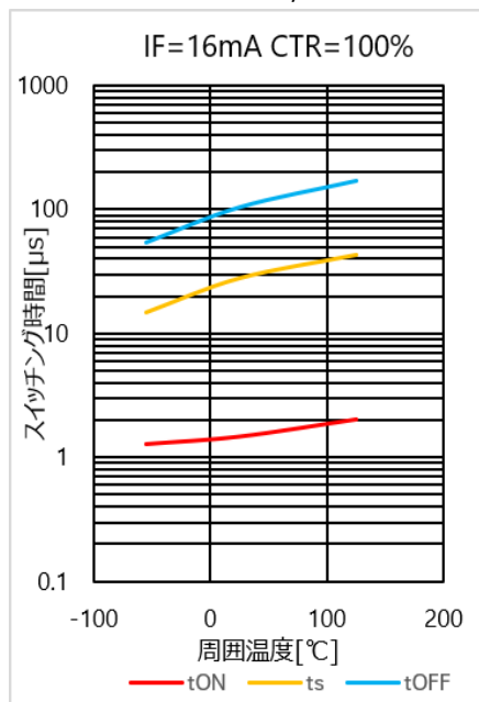
図 4.269 スイッチング時間 - Ta 特性(CTR=100%)
