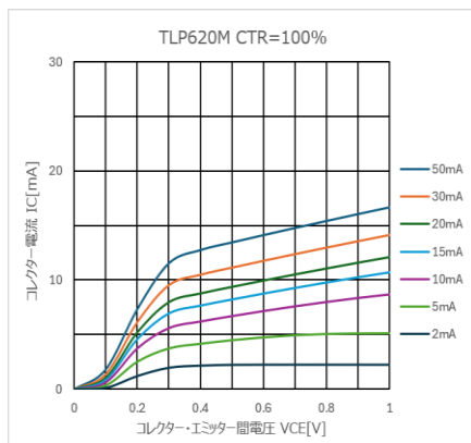
図 4.239 I_C - V_{CE} 特性 (CTR=100%)
