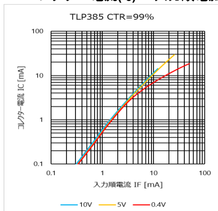
図 4.205 I_C - I_F 特性 (CTR=99%)
