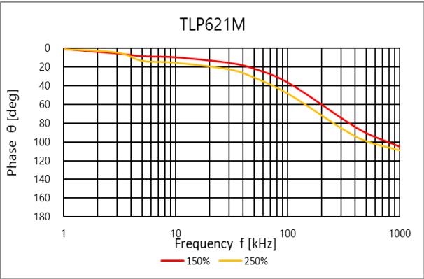
图 4.308 位相 \theta – 周波数
