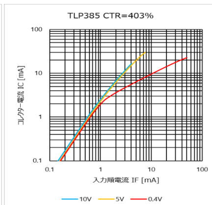
図 4.207 I_C - I_F 特性 (CTR=403%)
