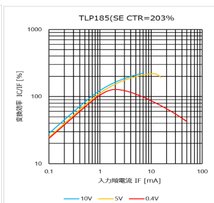
図 4.98 I_C/I_F - I_F 特性 (CTR=203%)
