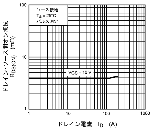
図 8.5 R_{DS(ON)} - I_D
