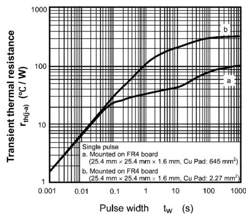
Fig. 8.13 r_{th(j-a)} - t_w
