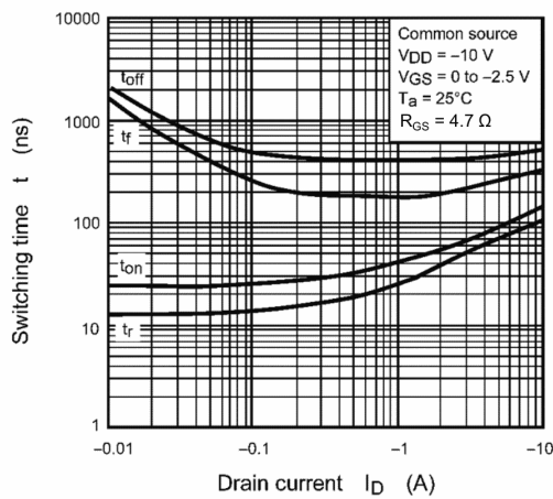
Fig. 8.11 t - I_D
