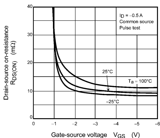
Fig. 8.3 R_{DS(ON)} - V_{GS}
