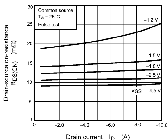
Fig. 8.5 R_{DS(ON)} - I_D
