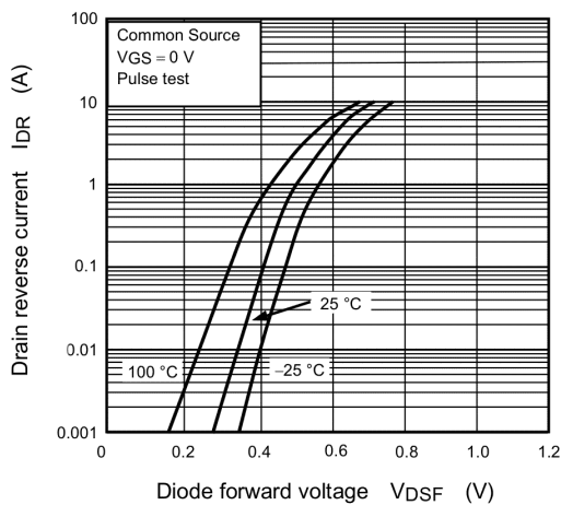
Fig. 8.9 I_{DR} - V_{DSF}
