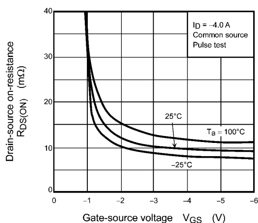
Fig. 8.4 R_{DS(ON)} - V_{GS}
