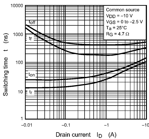
Fig. 8.11 t - I_D
