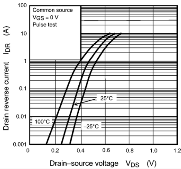
Fig. 8.9 I_{DR} - V_{DS}
