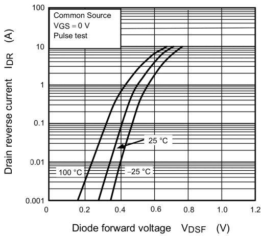
Fig. 9.9 I_{DR} - V_{DSF}
