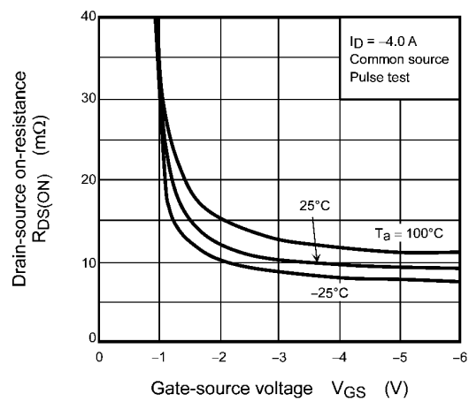
Fig. 8.4 R_{DS(ON)} - V_{GS}
