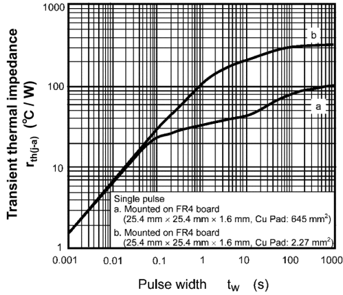
Fig. 9.13 r_{th(j-a)} - t_w
