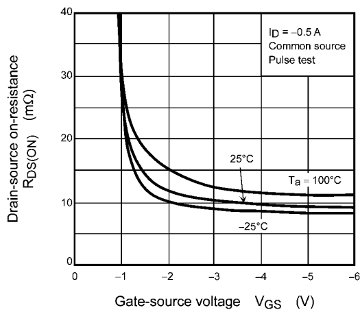
Fig. 8.3 R_{DS(ON)} - V_{GS}
