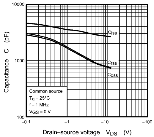
Fig. 9.10 C - V_{DS}
