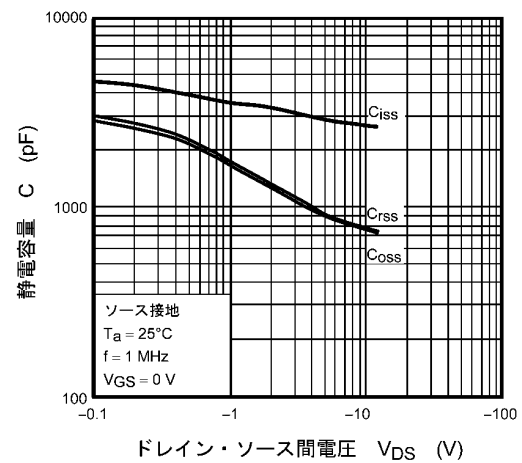
図 9.10 C - V_{DS}
