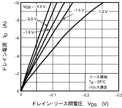
図 9.1 I_D - V_{DS}
