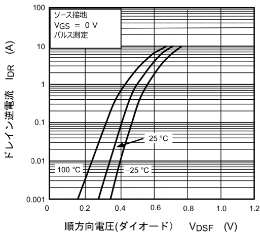
図 9.9 I_{DR} - V_{DSF}
