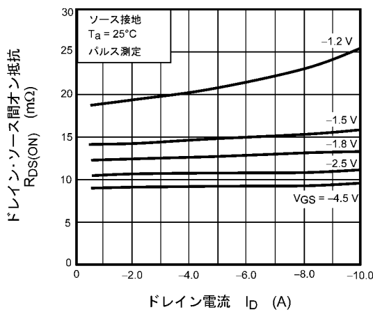
図 9.5 R_{DS(ON)} - I_D
