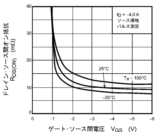
図 9.4 R_{DS(ON)} - V_{GS}
