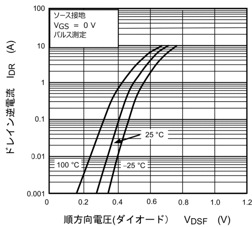
図 9.9 I_{DR} - V_{DSF}
