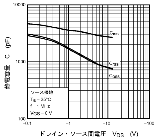
図 8.10 C - V_{DS}
