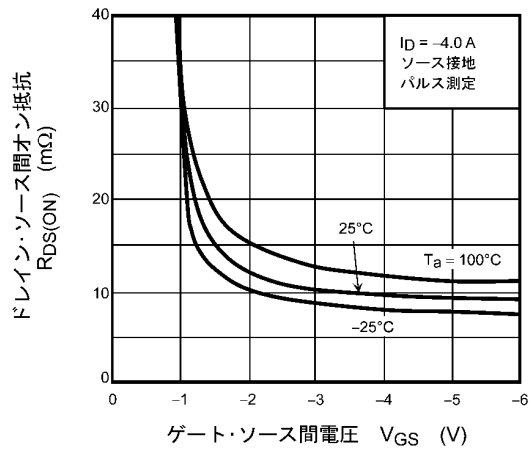
図 9.4 R_{DS(ON)} - V_{GS}
