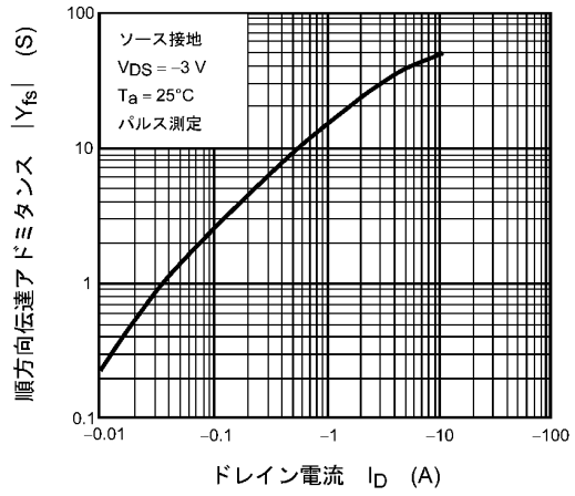
図 9.8 |Y_{fs}| - I_D
