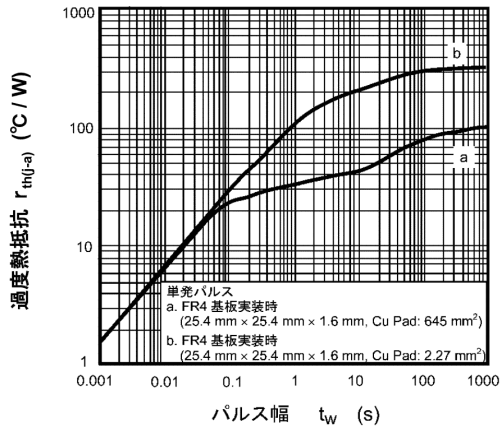
図 9.13 r_{th(j-a)} - t_w
