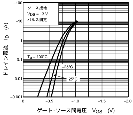
図 9.2 I_D - V_{GS}
