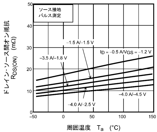
図 9.6 R_{DS(ON)} - T_a
