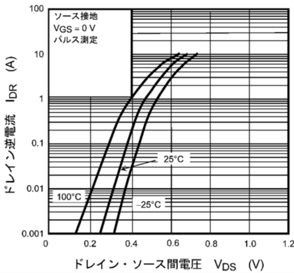
図 8.9 I_{DR} - V_{DS}
