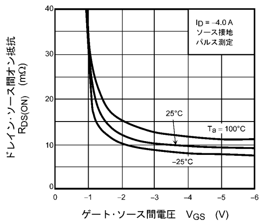
図 8.4 R_{DS(ON)} - V_{GS}
