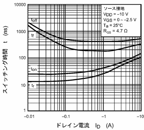
図 9.11 t - I_D
