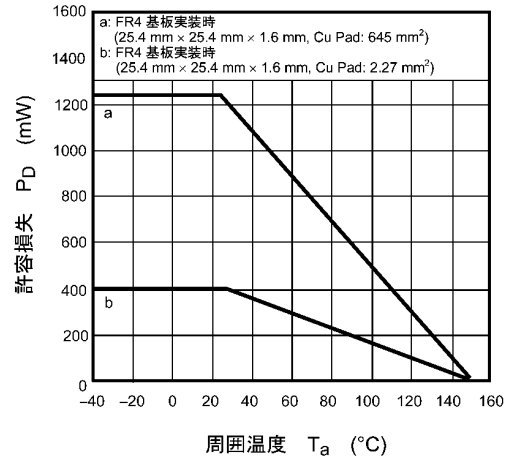
図 9.14 P_D - T_a
