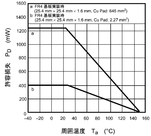
図 9.14 P_D - T_a
