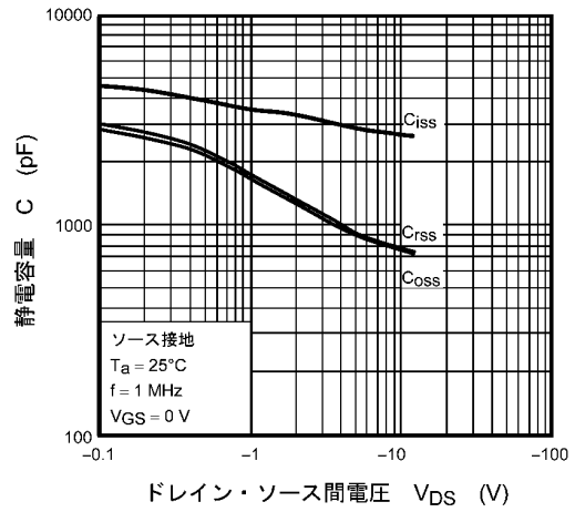
図 9.10 C - V_{DS}
