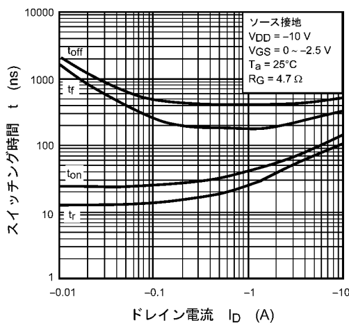
図 8.11 t - I_D
