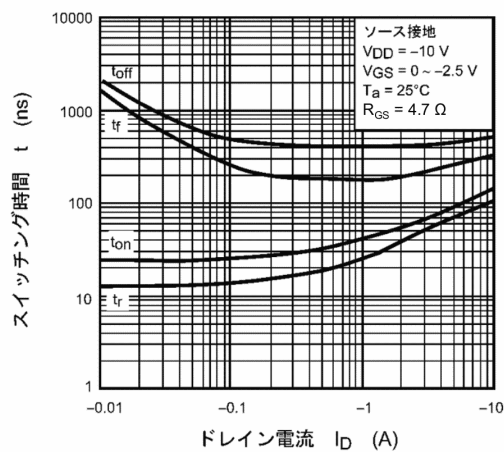
図 9.11 t - I_D
