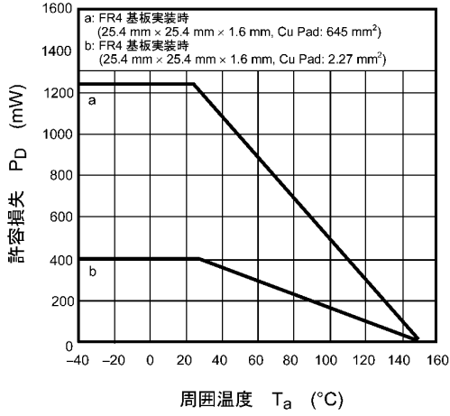
図 8.13 P_D - T_a
