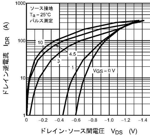
図 8.7 I_{DR} - V_{DS}
