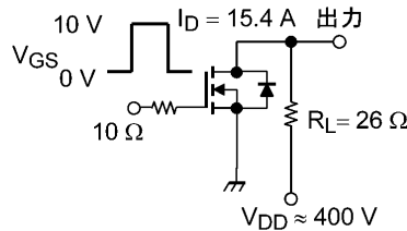
Duty \leq 1\% , t_w = 10\ \mu\text{s} 図 6.2.1 スwitchング時間の測定回路例
