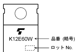
図 7.1 現品表示
