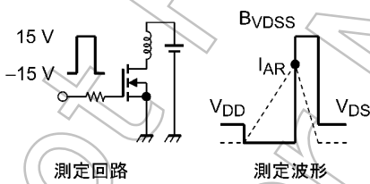
図 8.16 測定回路/測定波形
