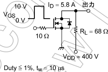
図 6.2.1 スwitching時間の測定回路例
