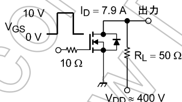
Duty \leq 1\% , t_w = 10\mu\text{s} 図 6.2.1 スwitching時間の測定回路例
