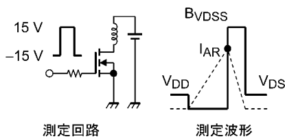
測定回路
