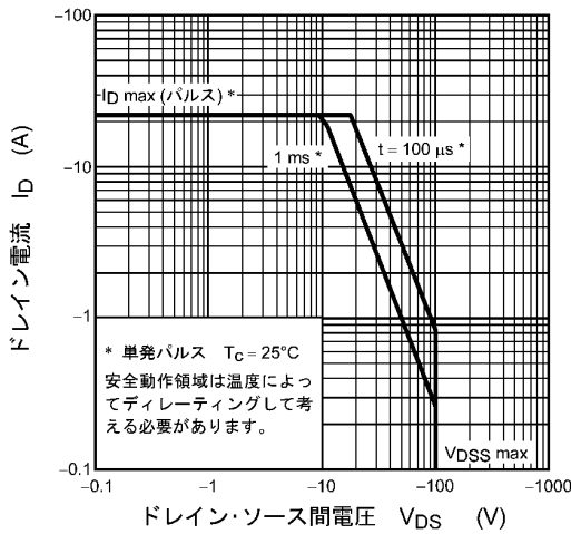
図 8.14 安全動作領域 (最大値 (保証値))
