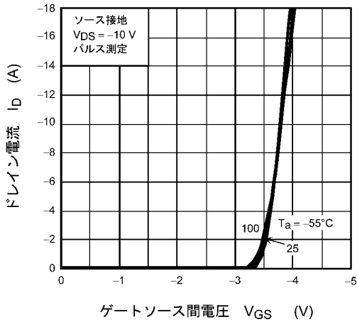
図 8.3 I_D - V_{GS}
