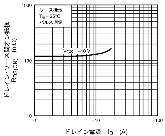
図 8.6 R_{DS(ON)} - I_D
