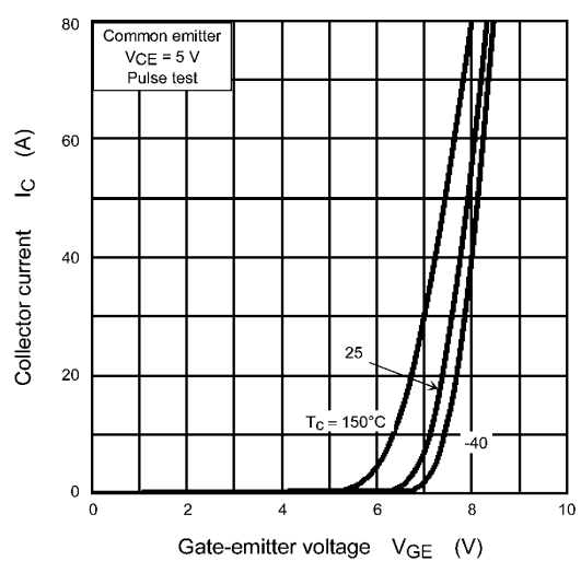
Fig. 8.4 I_C - V_{GE}
