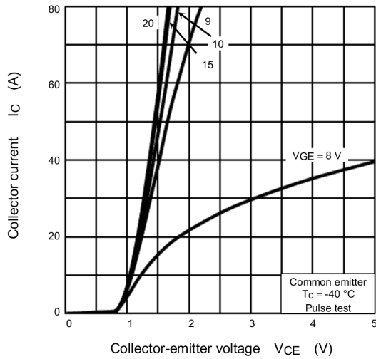
Fig. 8.3 I_C - V_{CE}
