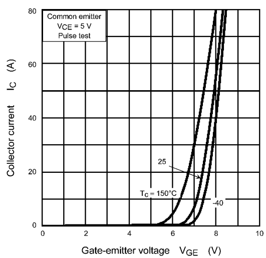
Fig. 8.4 I_C - V_{GE}
