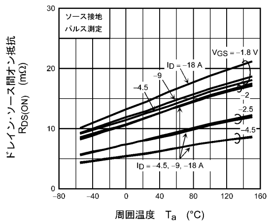
図 8.6 R_{DS(ON)} - T_a
