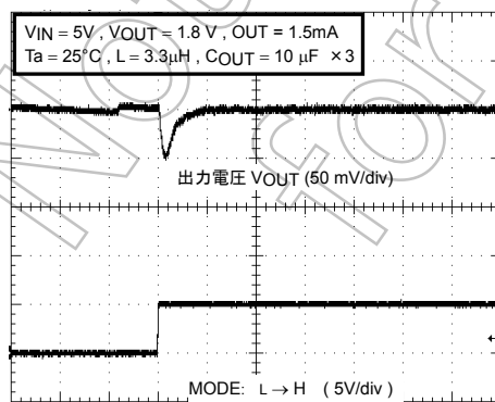
モード切換 I OUT =1.5mA (パルススキップ→連続 PWM)
