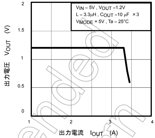
過電流特性
