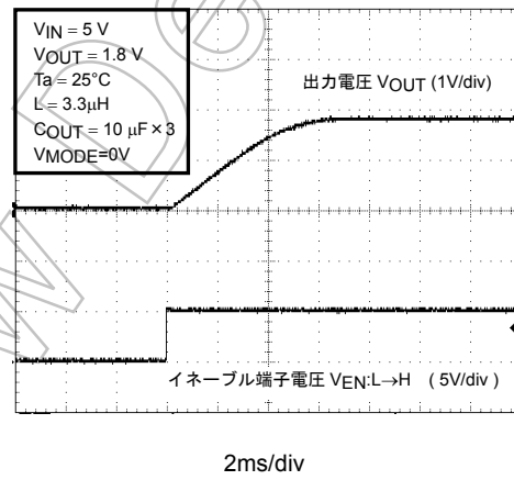
起動特性 (パルススキップ付きモード ソフトスタート時間)
