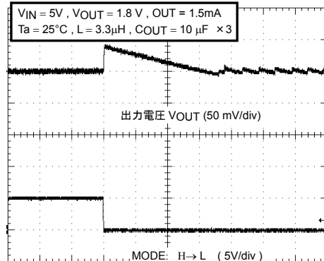
モード切換 I OUT =1.5mA (連続 PWM→パルススキップ)
