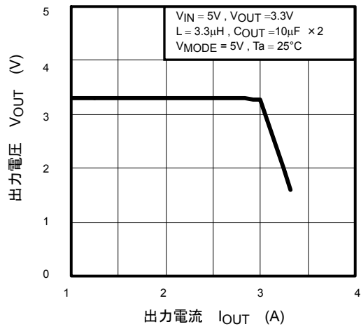
過電流特性
