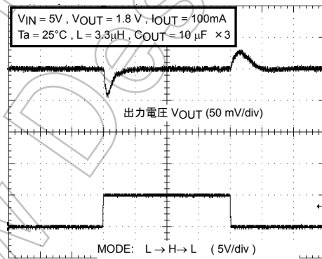
モード切換 I OUT =100mA (パルススキップ→連続 PWM→パルススキップ)
