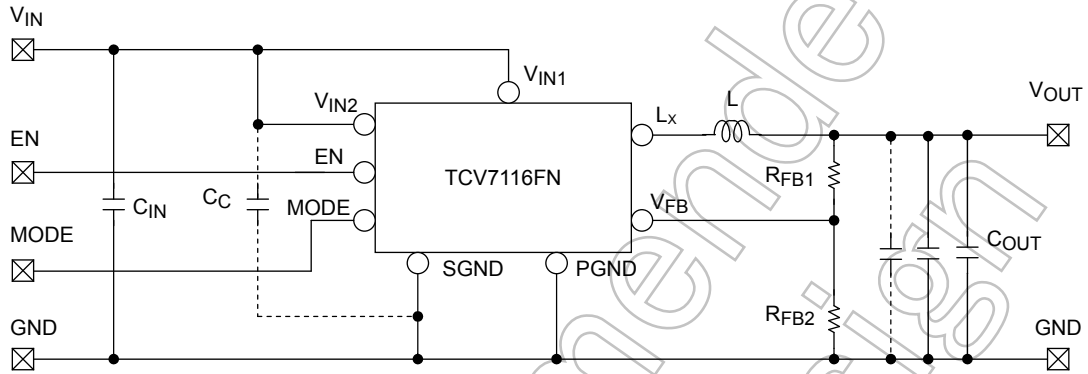
図 1 TCV7116FN 応用回路例
