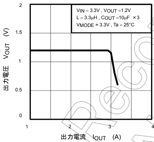
過電流特性
