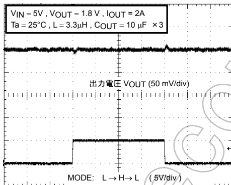
モード切換 I OUT =2A (パルススキップ→連続 PWM→パルススキップ)
