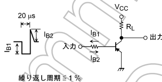
図 5.2.1 スwitchング時間の測定回路
