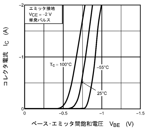
図 7.5 I_C - V_{BE}
