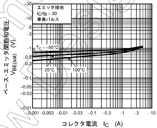
図 7.4 V_{be(sat)} - I_c
