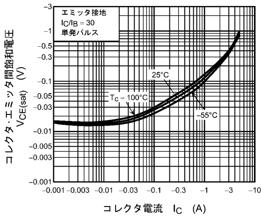
図 7.3 V_{CE(sat)} - I_C
