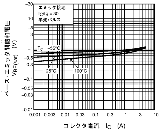
図 7.4 V_{BE(sat)} - I_C
