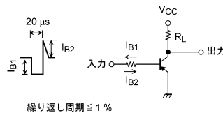
図 5.2.1 スwitching時間の測定回路
