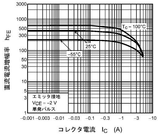
図 7.2 h_{FE} - I_C
