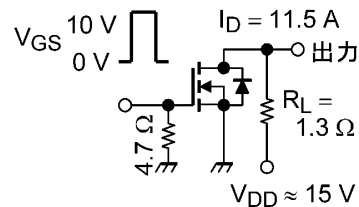
図 6.2.1 スwitchング時間の測定回路
