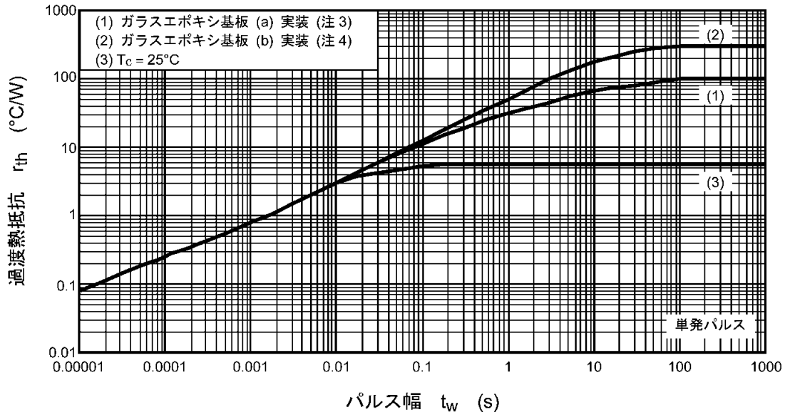
図 8.13 r_{th} - t_w (最大値 (保証値))
