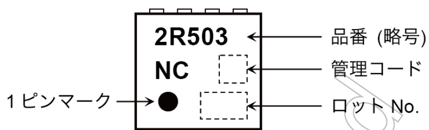
図 7.1 現品表示
