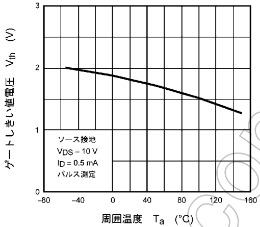
図 8.9 V_{th} - T_a
