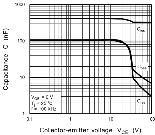
Fig. 7.3 C_{ies}, C_{oes}, C_{res} - V_{CE}
