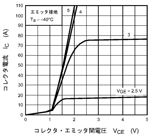
図 9.1 I_C - V_{CE}
