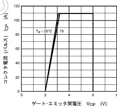
図 9.12 最小ゲート駆動電圧領域
