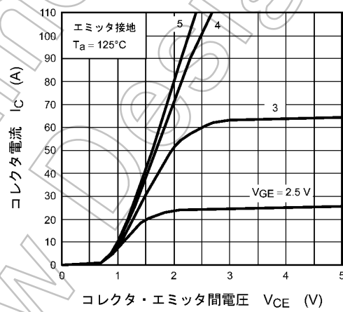
図 9.4 I_C - V_{CE}
