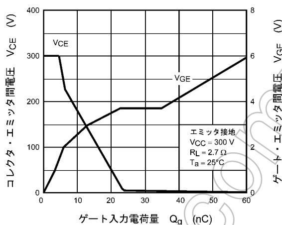
図 9.9 V_{CE}, V_{GE} - Q_g
