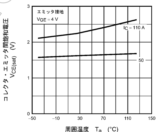
図 9.6 V_{CE(sat)} - T_a
