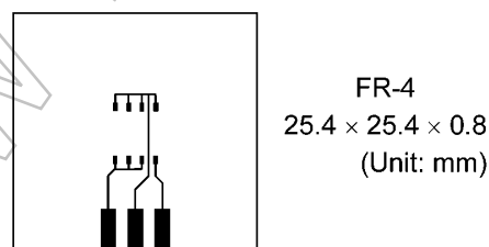
図 5.2 ガラスエポキシ基板 実装例b
