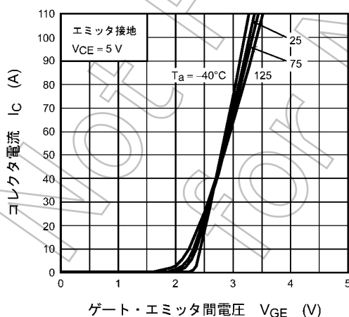
図 9.5 I_C - V_{GE}
