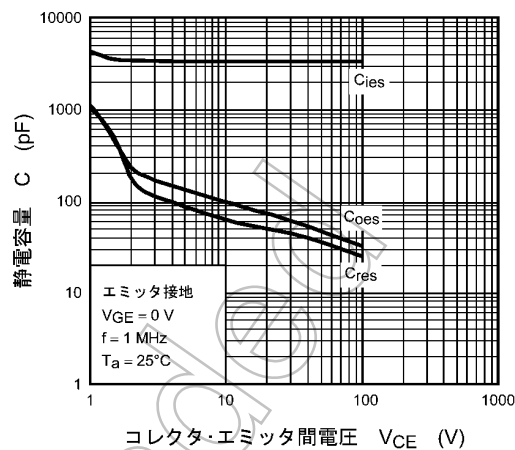
図 9.8 C - V_{CE}
