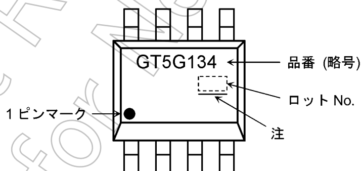
図 7.1 現品表示
