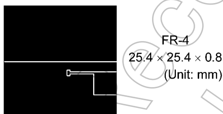
図 5.1 ガラスエポキシ基板 実装例a
