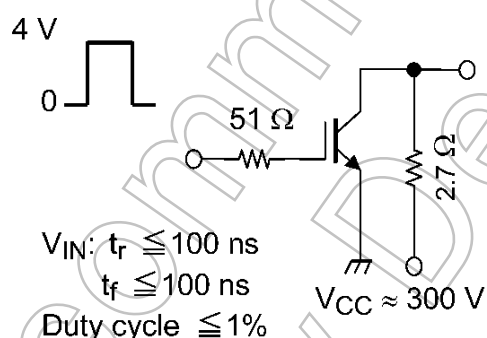
図 6.2.1 スwitchング時間の測定回路
