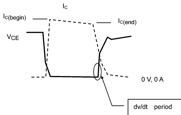
図 8.1 波形 (全体)
