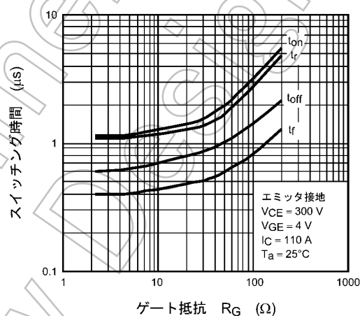
図 9.10 スwitching時間 - R_G
