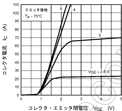
図 9.3 I_C - V_{CE}
