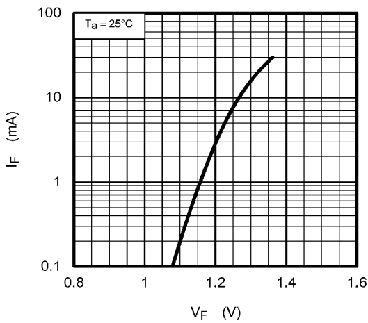
図 13.1.3 I_F - V_F
