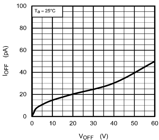
図 13.1.9 I_{OFF} - V_{OFF}
