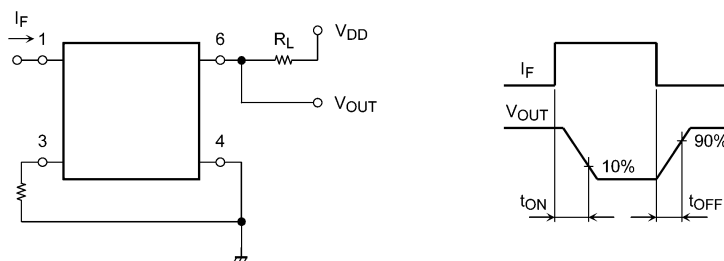
図 12.1 スイッチング時間測定回路, 波形
