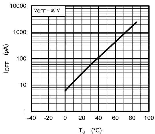
図 13.1.10 I_{OFF} - T_a
