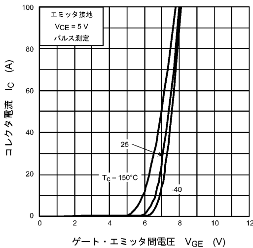
図 8.5 I_C - V_{GE}
