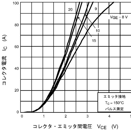
図 8.3 I_C - V_{CE}
