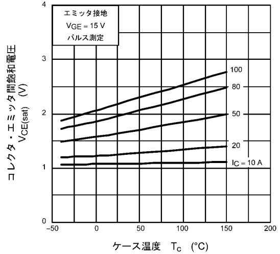
図 8.4 V_{CE(sat)} - T_C
