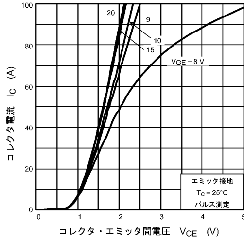
図 8.2 I_C - V_{CE}
