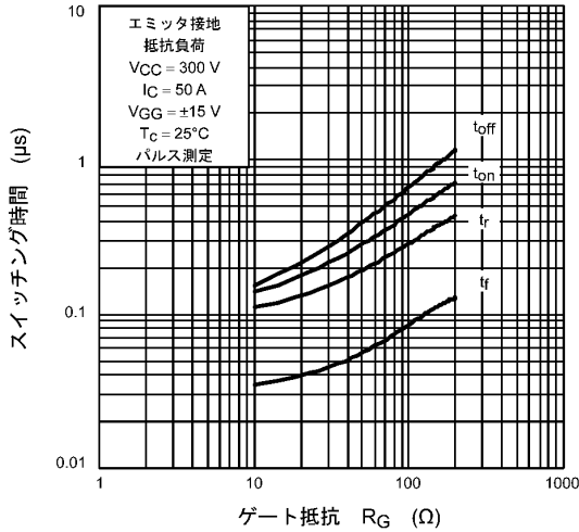
図 8.7 スイッチング時間 - R_G
