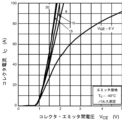
図 8.1 I_C - V_{CE}
