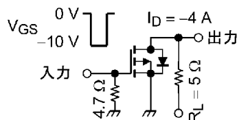
図 6.2.1 スwitching時間の測定回路例
