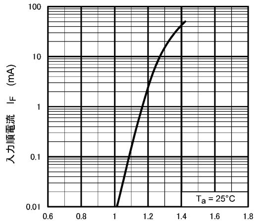
入力順電圧 V_F (V) 図 11.4 I_F - V_F
