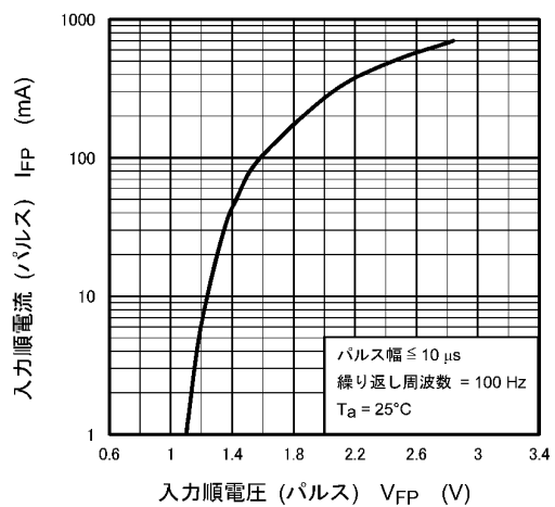
図 11.6 I_{FP} - V_{FP}
