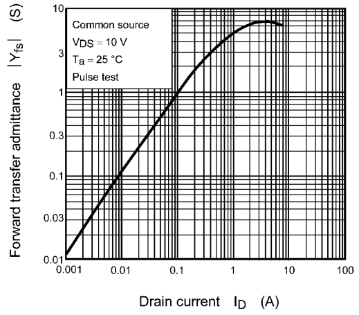
Fig. 8.8 |Y_{fs}| - I_D
