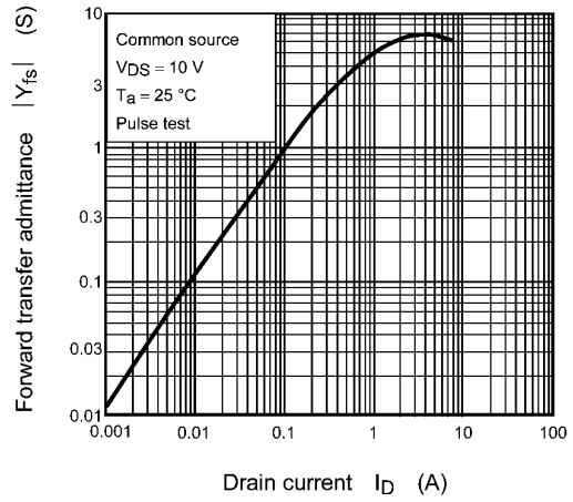
Fig. 8.8 |Y_{fs}| - I_D
