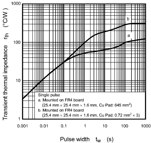
Fig. 8.13 r_{th} - t_w
