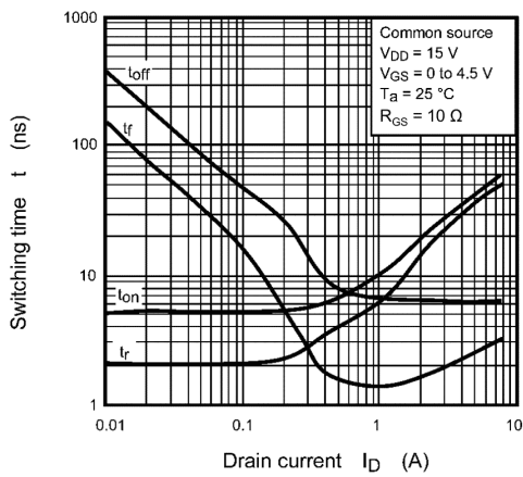
Fig. 8.11 t - I_D
