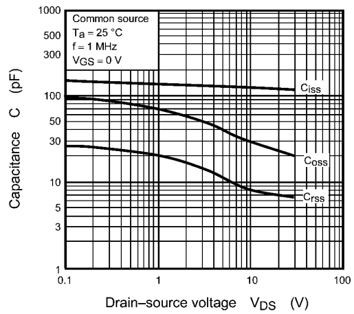
Fig. 8.10 C - V_{DS}
