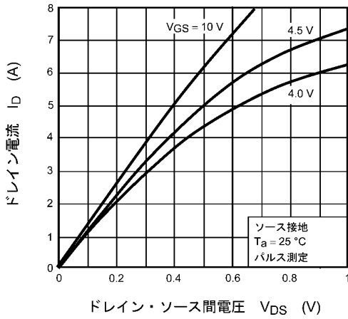
図 8.1 I_D - V_{DS}
