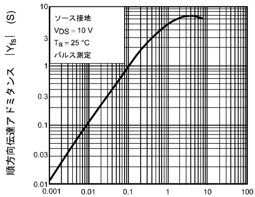
図 8.8 |Y_{fs}| - I_D
