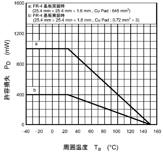
図 8.14 P_D - T_a
