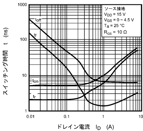
図 8.11 t - I_D
