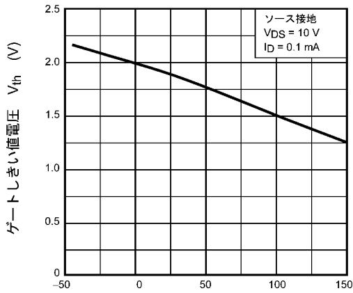
図 8.7 V_{th} - T_a
