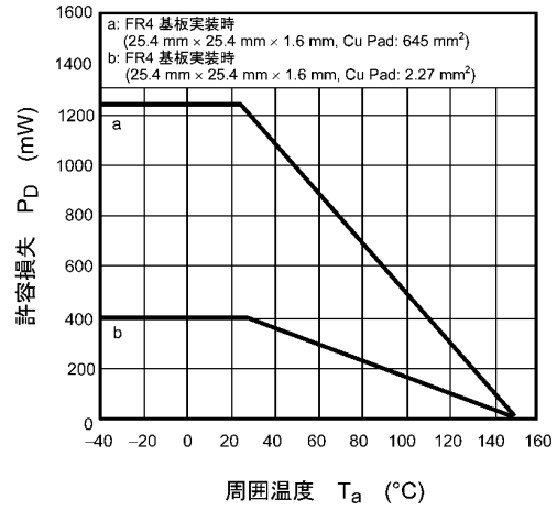
図 8.14 P_D - T_a
