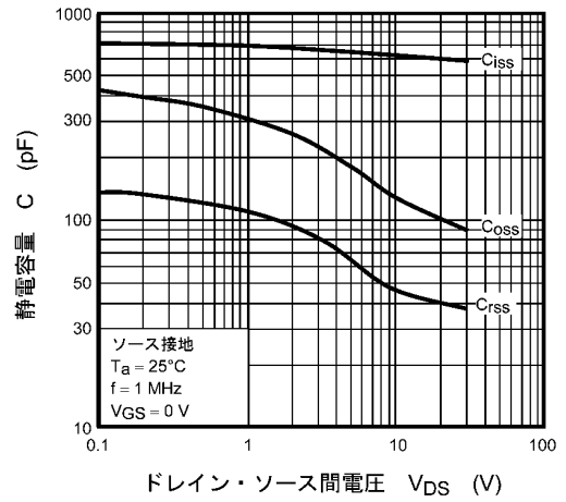
図 7.10 C - V_{DS}
