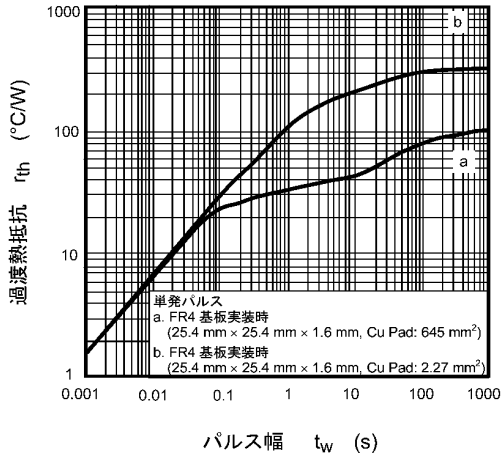
図 8.13 r_{th} - t_w
