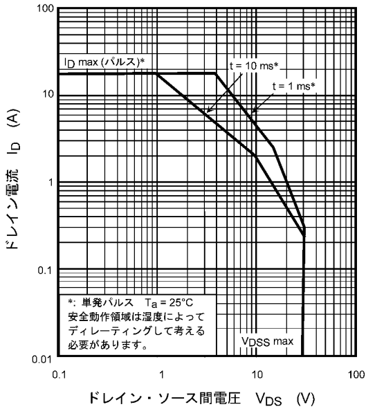
図 8.15 安全動作領域
