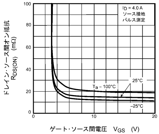
図 8.4 R_{DS(ON)} - V_{GS}
