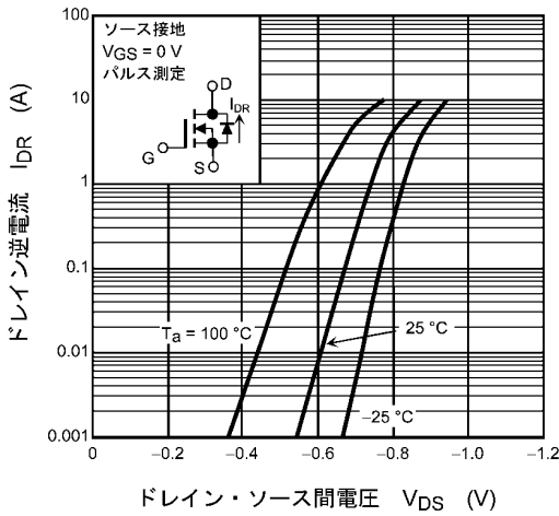
図 7.9 I_{DR} - V_{DS}
