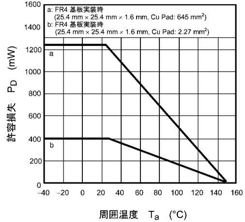
図 7.14 P_D - T_a
