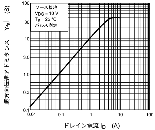
図 8.8 |Y_{fs}| - I_D
