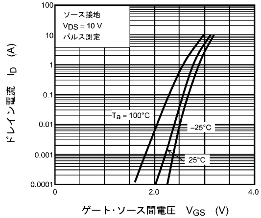
図 8.2 I_D - V_{GS}
