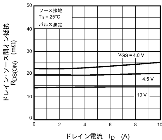
図 7.5 R_{DS(ON)} - I_D
