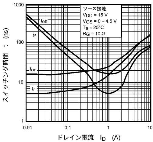
図 7.11 t - I_D
