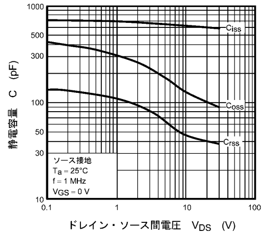
図 8.10 C - V_{DS}
