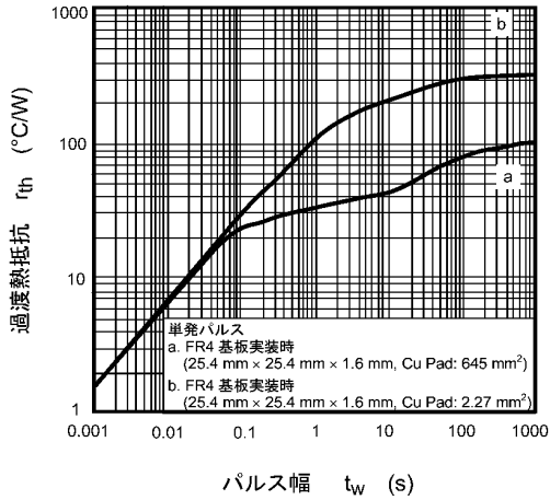
図 7.13 r_{th} - t_w
