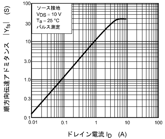
図 7.8 |Y_{fs}| - I_D
