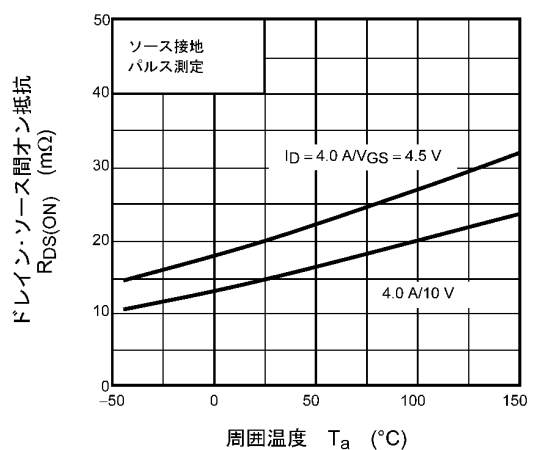
図 7.6 R_{DS(ON)} - T_a
