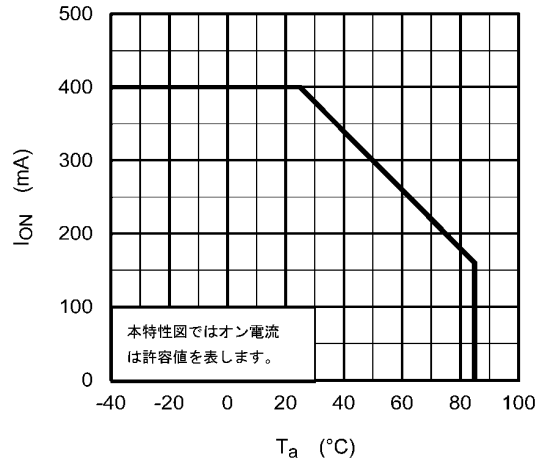
図 12.1.2 I_{ON} - T_a
