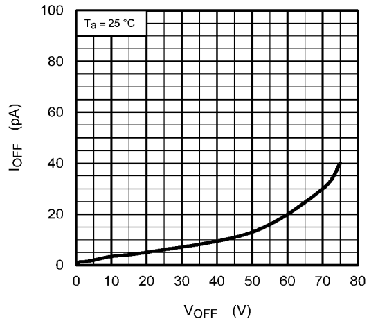
図 12.1.10 I_{OFF} - V_{OFF}
