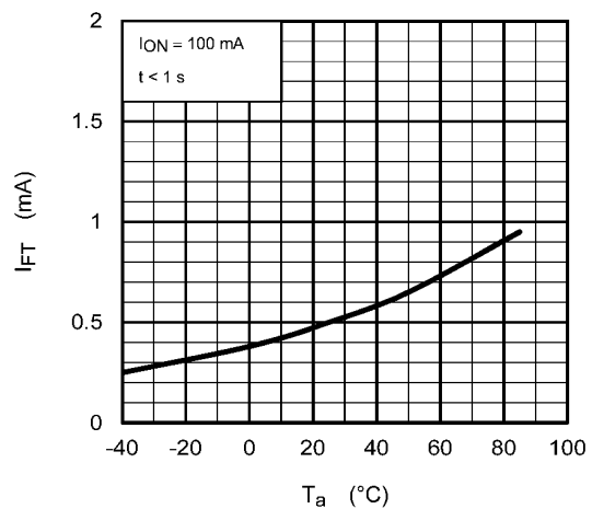
図 12.1.6 I_{FT} - T_a
