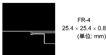
図 5.1 ガラスエポキシ基板 実装例a
