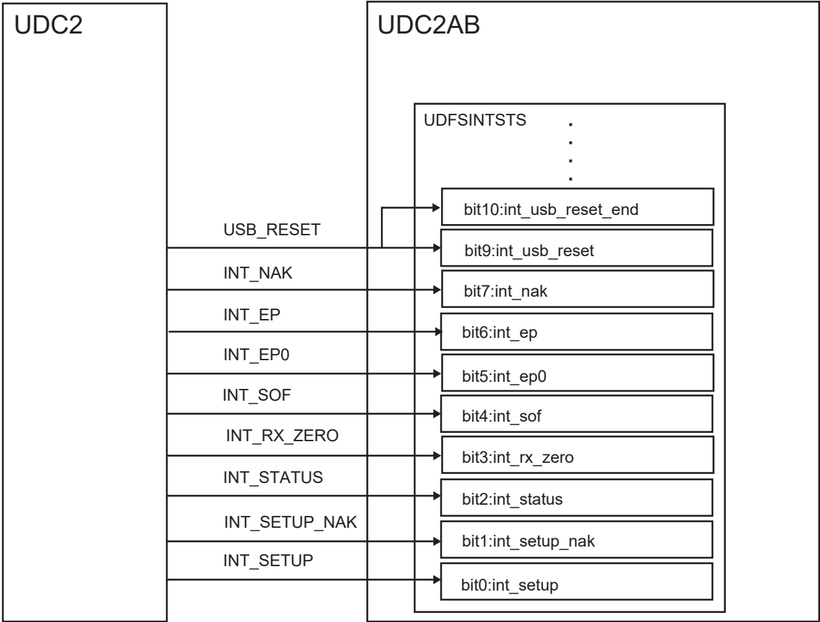
図 17-7 フラグ出力信号と割り込みビットの接続関係
