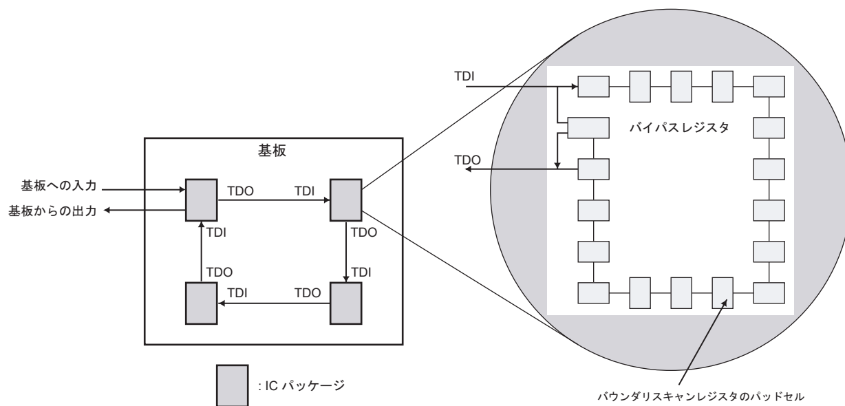
図 33-4 バイパスレジスタの機能
