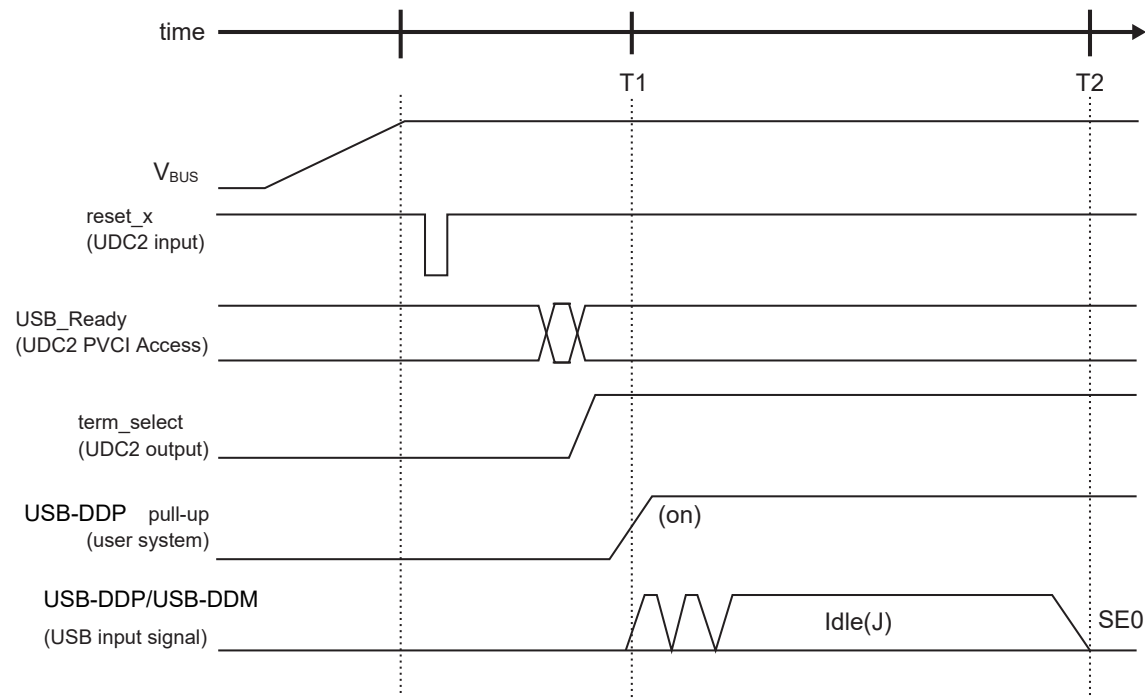
図 17-26 コネクト動作タイミング
