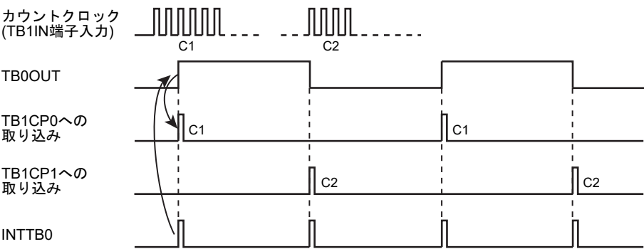
図 11-7 周波数測定
