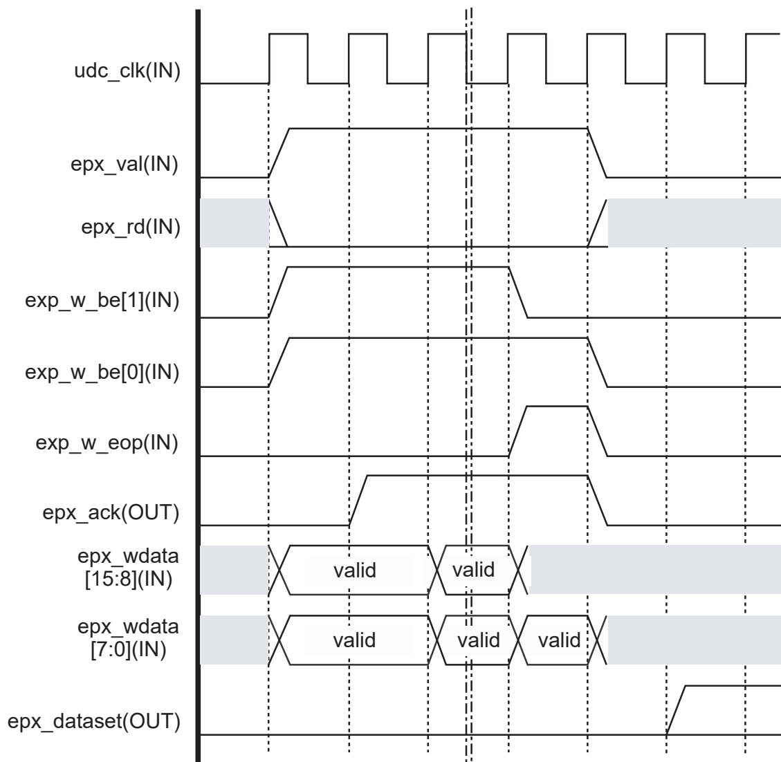
図 17-32 <max_pkt>=偶数で MPS(奇数)ライト時のアクセス (EP 直接アクセス)
