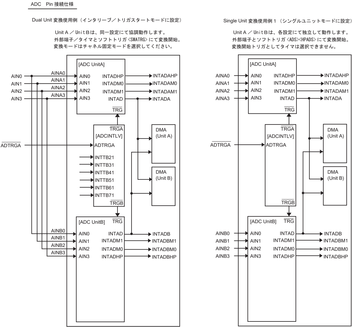
図 21-1 ブロック図 1
