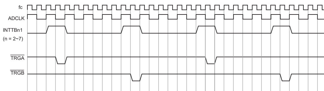
図 21-9 タイマトリガによるトリガスタート動作 (ADCLK=fc/2)
