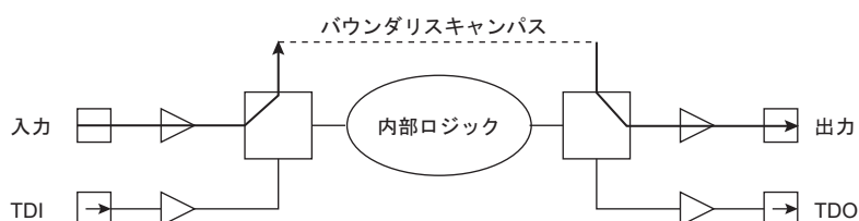
図 33-7 EXTEST 命令が選択されているときのテストデータの流れ
