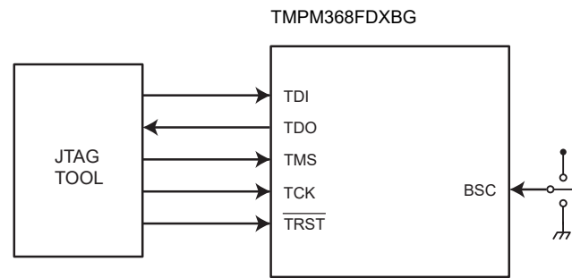
図 33-1 JTAG 開発ツールとの接続例
