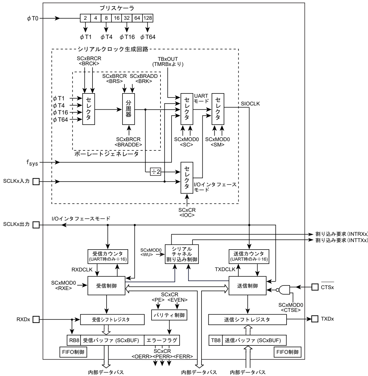
図 12-1 SIO/UART ブロック図
