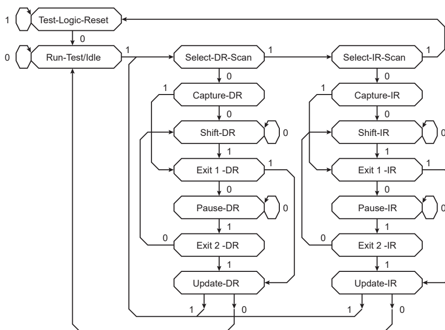
図 33-6 TAP コントローラの状態遷移図
