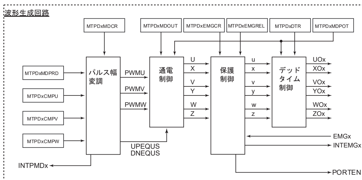
図 23-21 PMD 回路概略図
