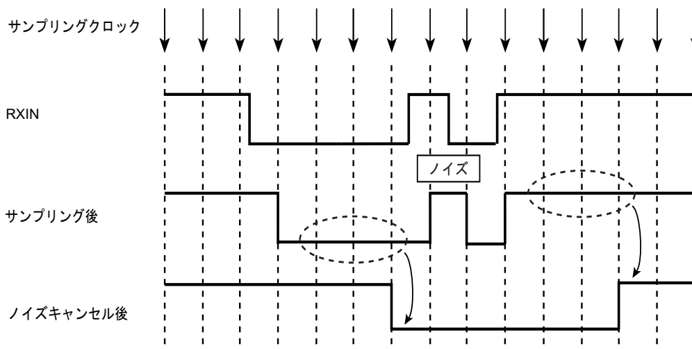
図 20-3 ノイズキャンセル(RMCRCR4<RMCNC[3:0]>="0011"(3 サイクル)の場合)
