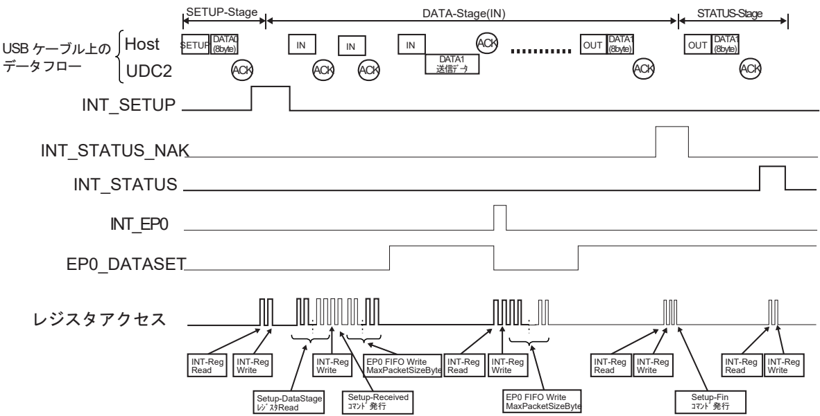
図 17-25 Control-RD 転送における INT_STATUS_NAK フラグの使用例
