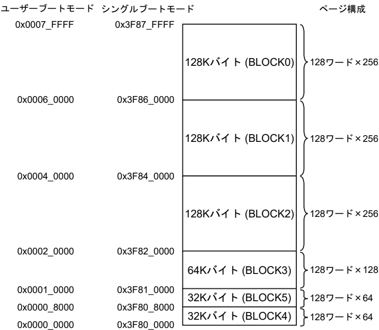
図 30-10 ブロック構成(TMPM368FDXBG)
