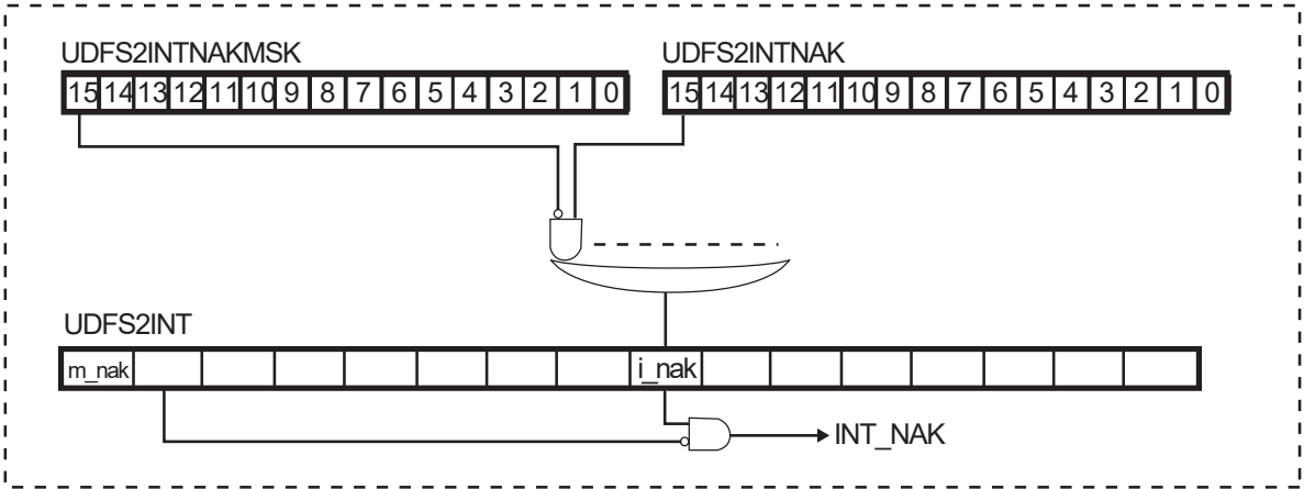
図 17-12 割り込みステータスとマスクレジスタ
