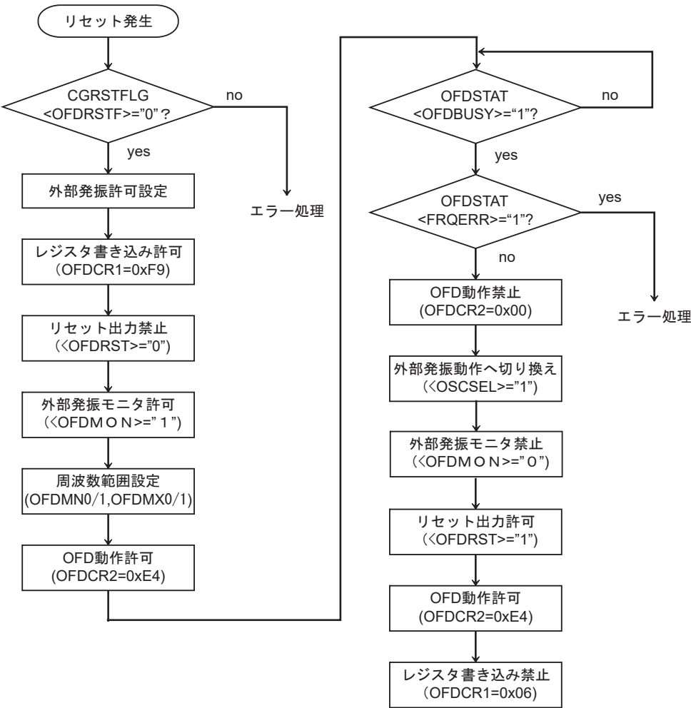
図 28-3 動作手順例
