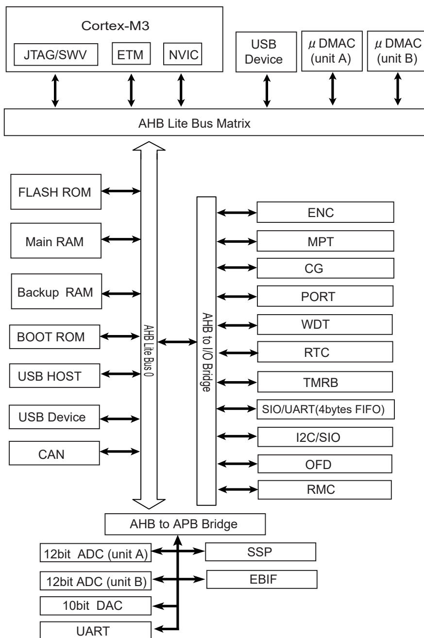
図 1-1 TMPM368FDXBG ブロック図
