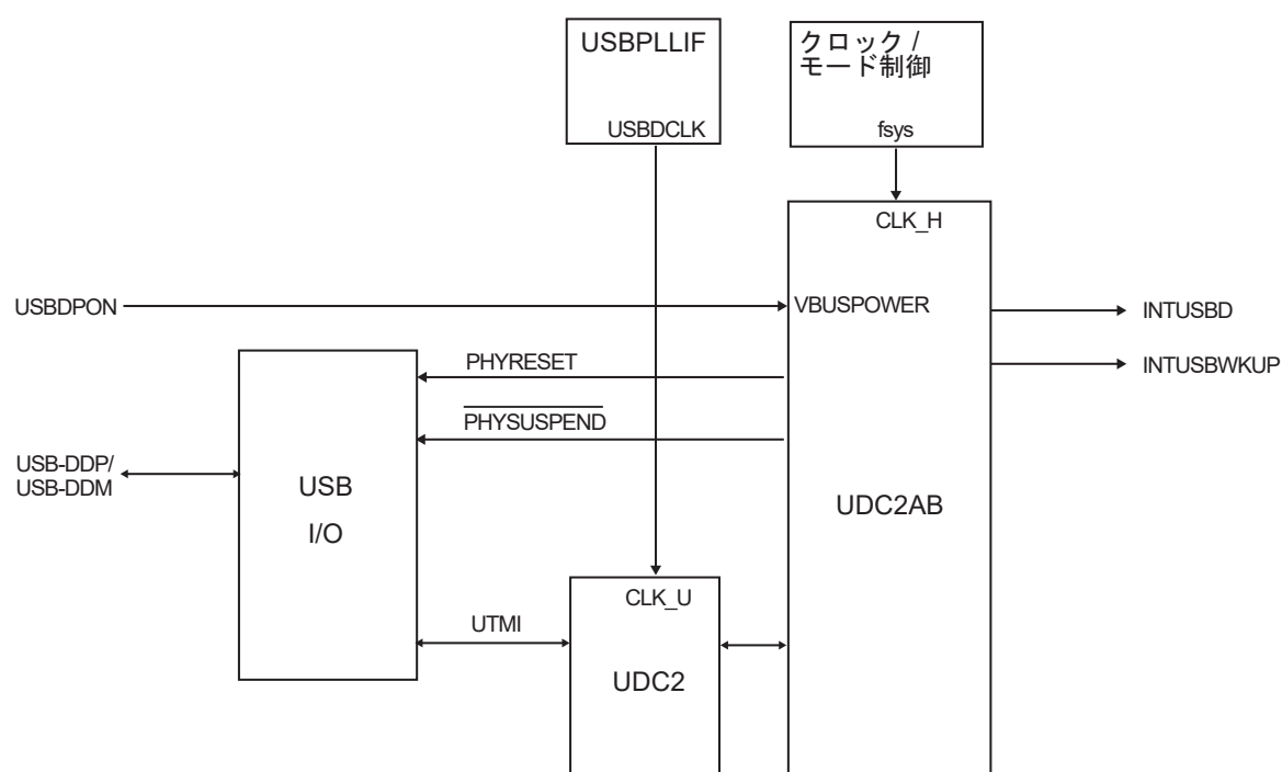
図 17-16 パワーマネージメント制御信号の接続図
