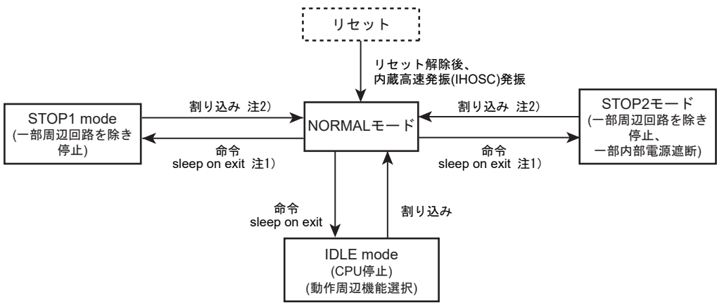
図 5-2 モード状態遷移図
