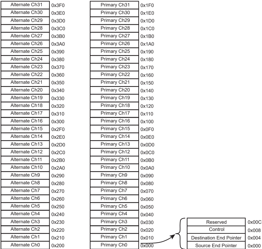
図 8-2 制御データのメモリマップ
