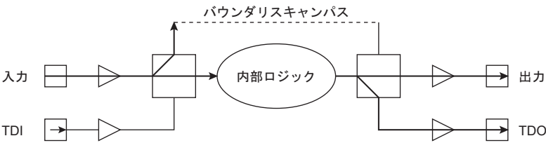
図 33-8 SAMPLE が選択されているときのテストデータの流れ
