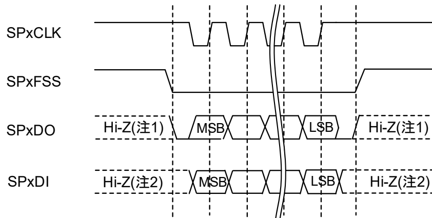
図 15-9 SPI フレームフォーマット (&lt;SPO&gt;=1 &amp; &lt;SPH&gt;=1)
