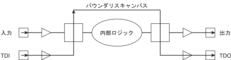
図 33-9 PRELOAD が選択されているときのテストデータの流れ
