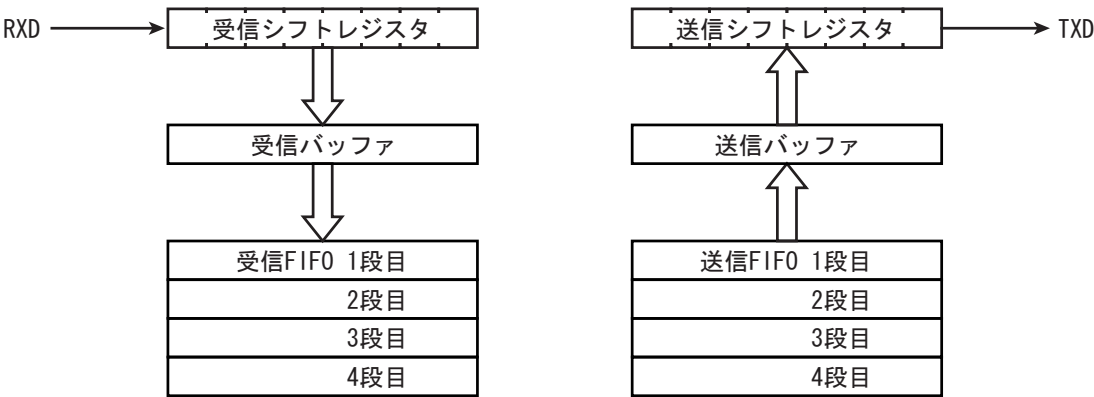
図 12-3 バッファと FIFO の構成
