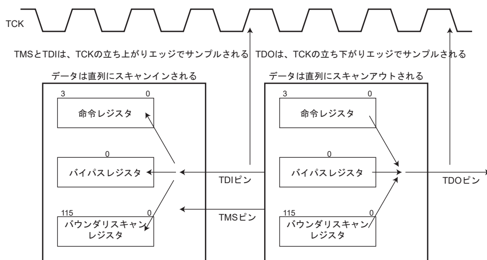
図 33-5 JTAG テストアクセスポート
