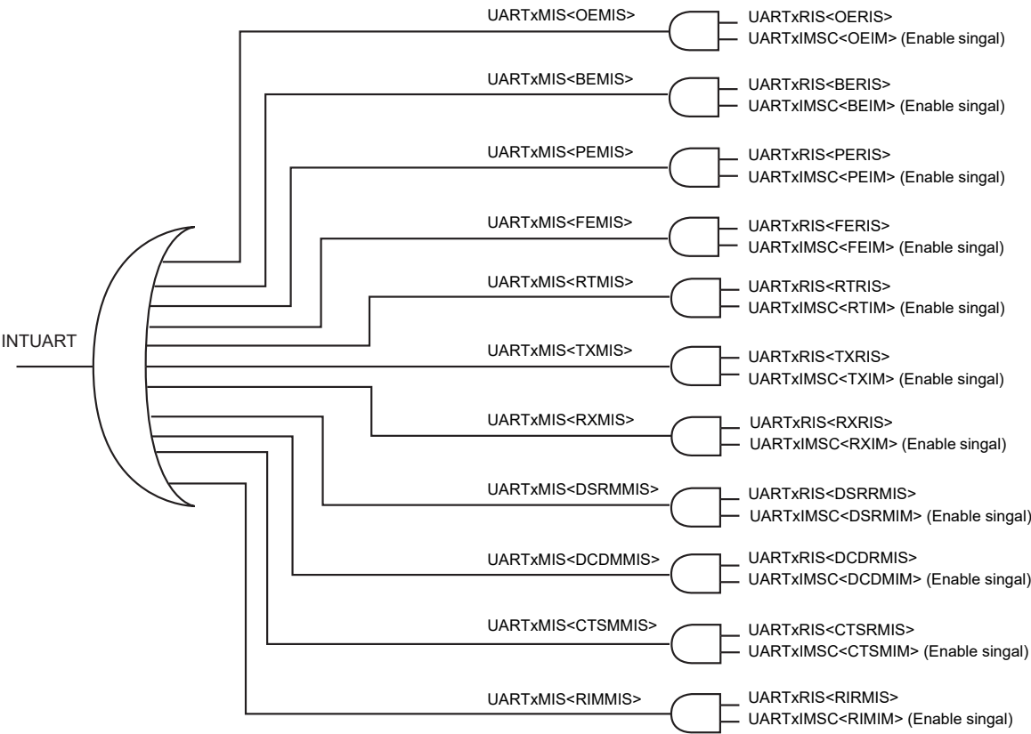
図 13-2 UART 割り込みブロック
