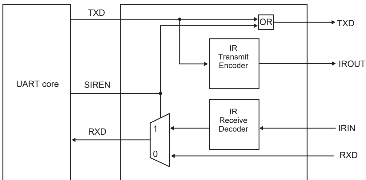
図 13-3 IrDA 回路のブロックダイヤグラム
