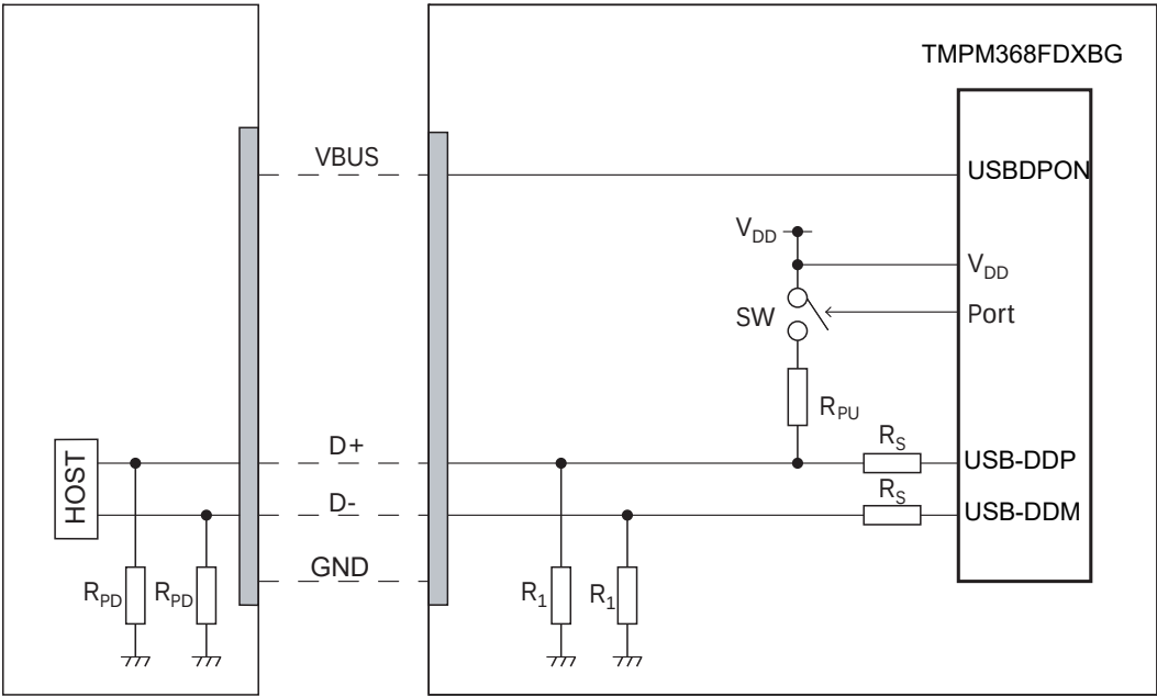
図 17-6 USB バスと TMPM368FDXBG の接続例
