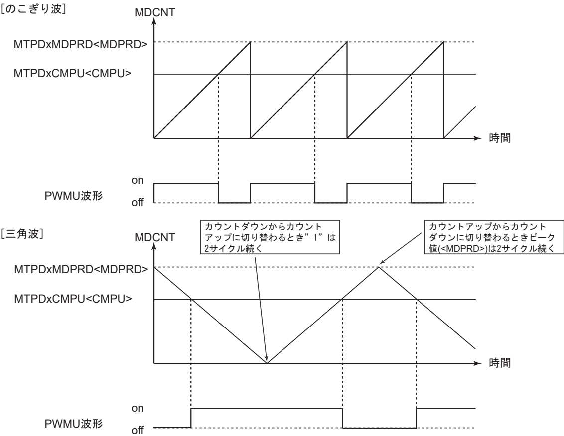
図 21-23 PWM 波形
