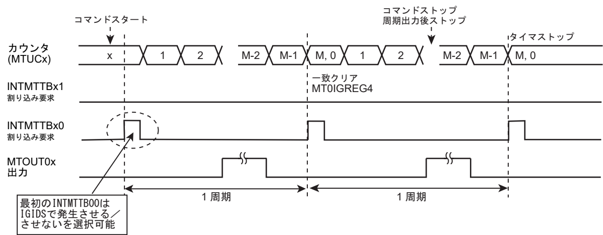
図 21-7 周期割り込み動作
