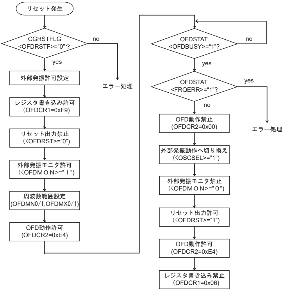
図 26-3 動作手順例
