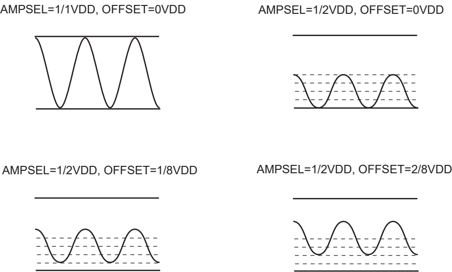
図 20-2 正弦波出力波形
