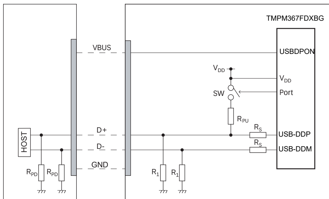
図 17-6 USB バスと TMPM367FDXBG の接続例
