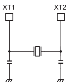
図 33-2 低周波発振回路例
