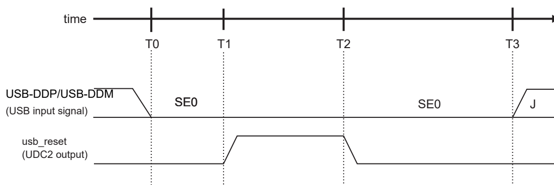
図 17-27 リセット動作タイミング図
