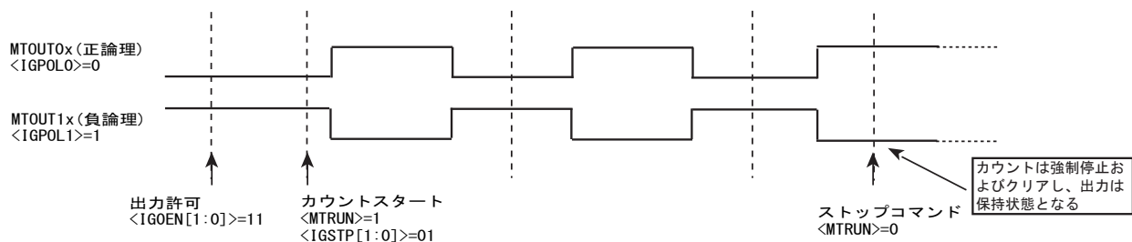
図 21-14 出力保持状態でカウント停止
