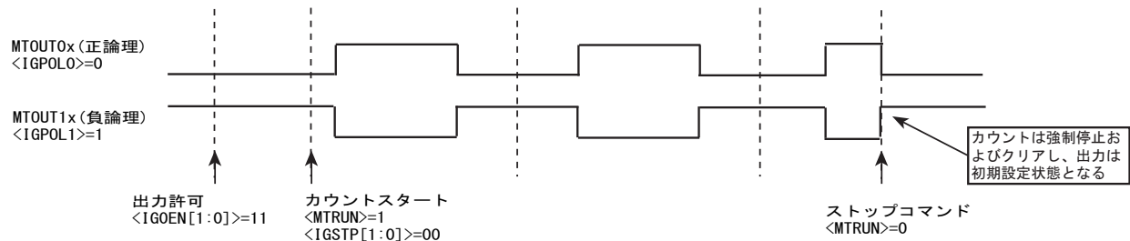
図 21-13 出力初期状態でカウント停止
