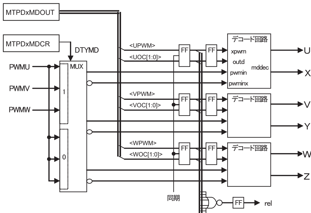
図 21-24 通電制御回路概略図
