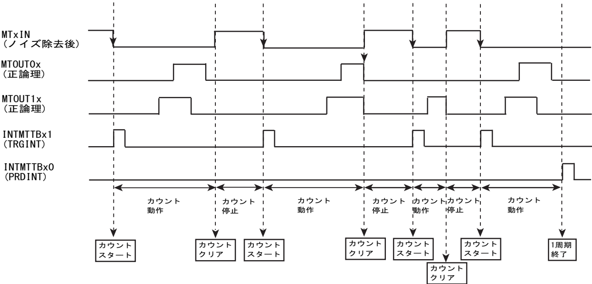
図 21-18 トリガ常時受け付け
