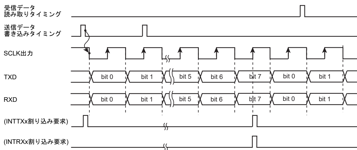
<WBUF> = "1" (ダブルバッファ許可)の場合
