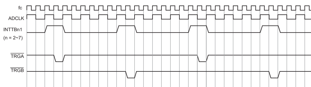
図 19-9 タイマトリガによるトリガスタート動作 (ADCLK=fc/2)
