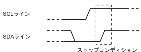
図 14-6 ストップコンディションの発生
