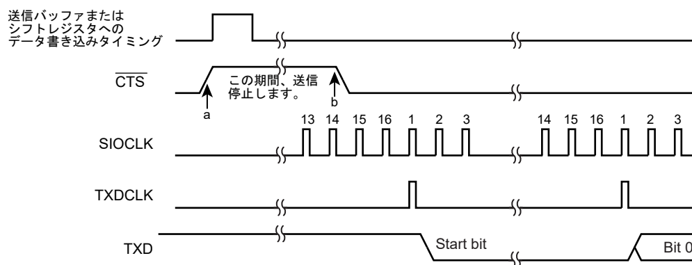
図 12-9 \overline{CTS} 信号のタイミング
