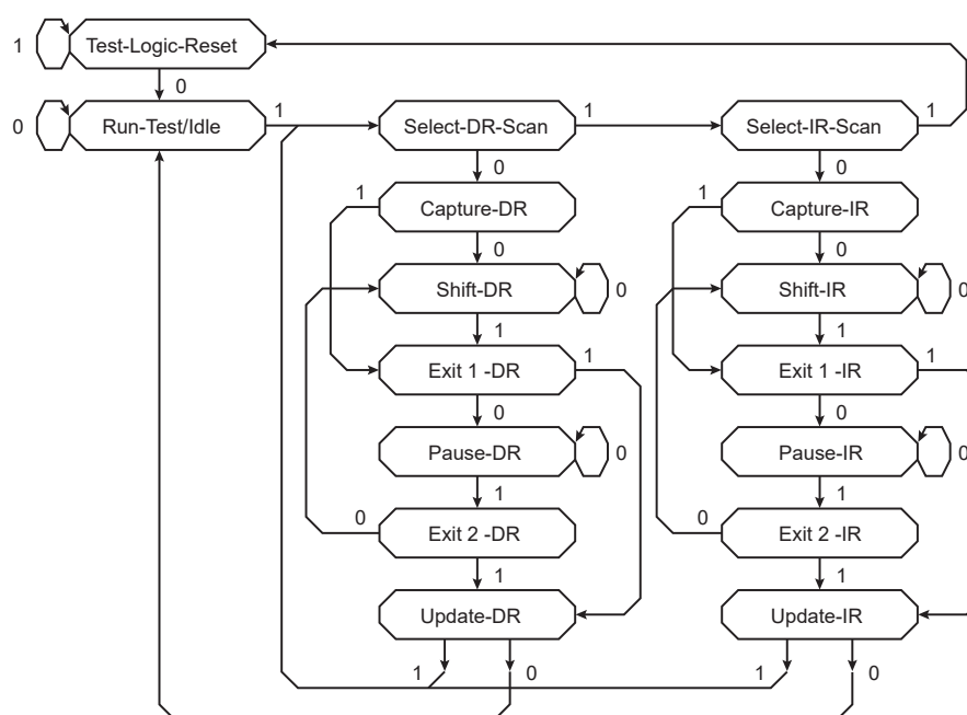
図 31-6 TAP コントローラの状態遷移図
