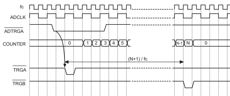
図 19-8 外部トリガによるインターリーブ動作 ( ADCLK=fc/2 )
