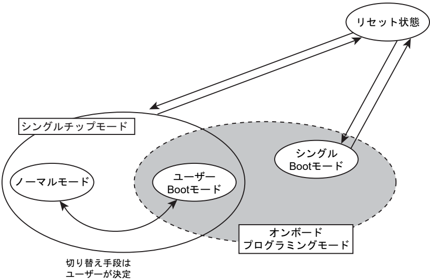
図 28-2 モード遷移図
