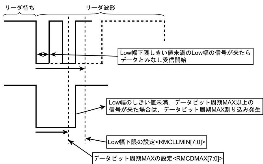
図 18-8 リーダ待ち状態なしでのリーダーなしのリモコン信号の場合 (RMCRCR2<RMCLD>="1"の時)
