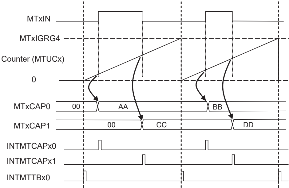
図 21-10 キャプチャ動作
