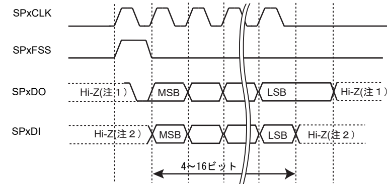
図 15-2 SSI フレームフォーマット（シングル転送送受信）
