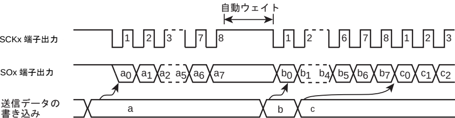
図 14-15 自動ウェイト機能
