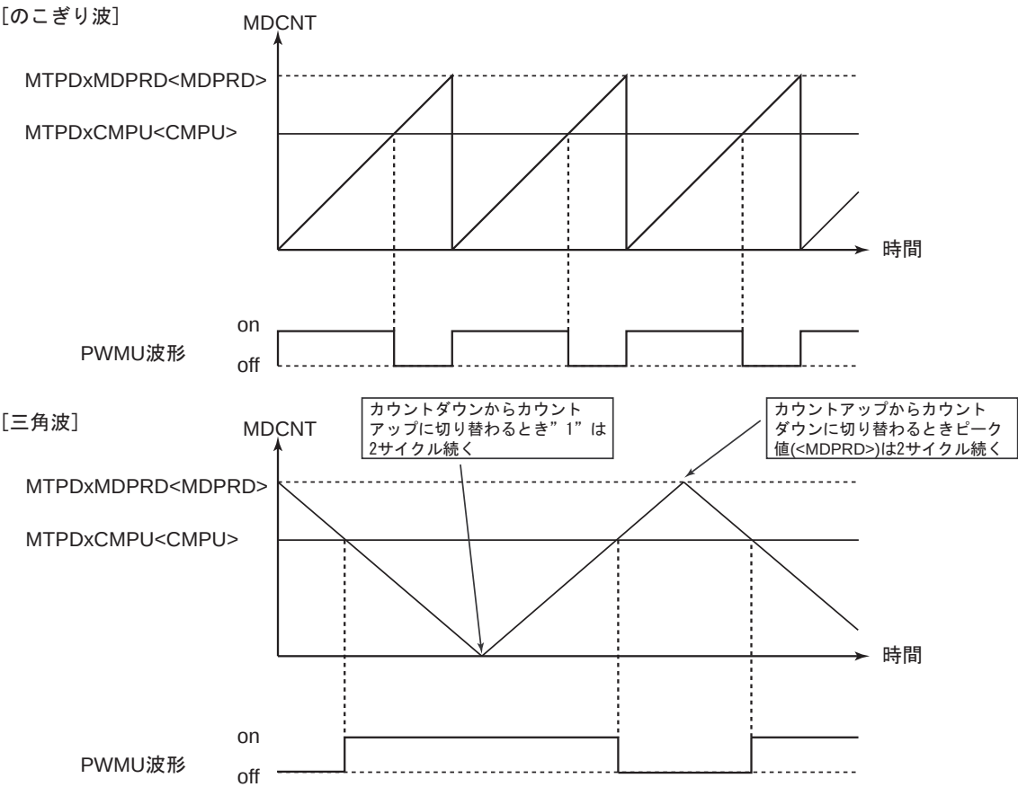
図 24-23 PWM 波形
