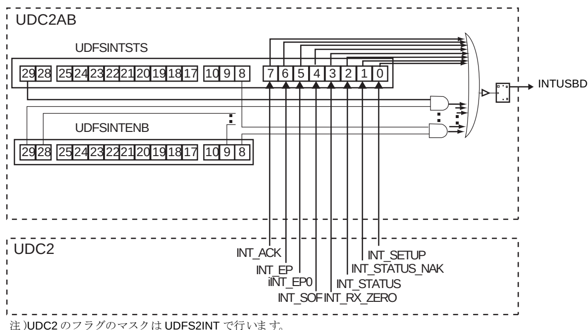
図 17-13 INTUSBD とレジスタの関係
