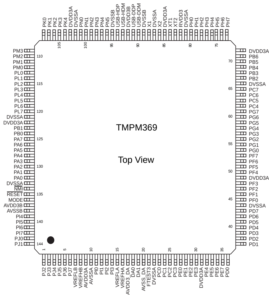
図 1-2 ピン配置図
