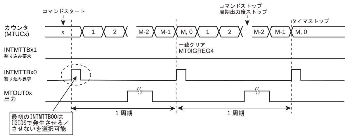
図 24-7 周期割り込み動作
