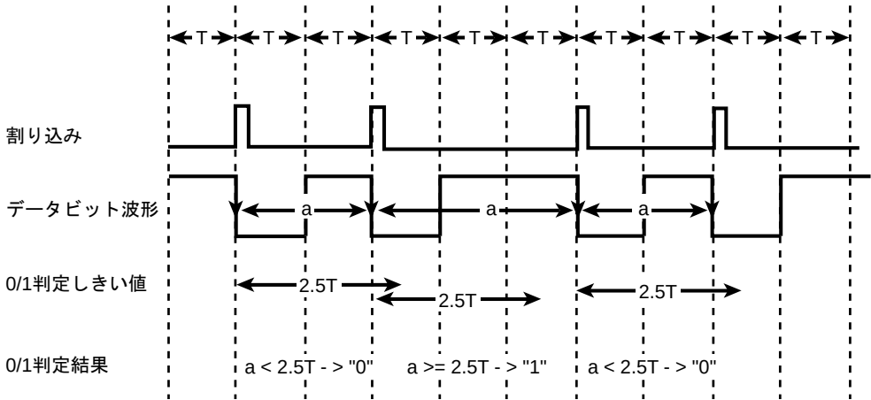
図 21-5 データビットの 0/1 判断の方法(しきい値 2.5T の場合)
