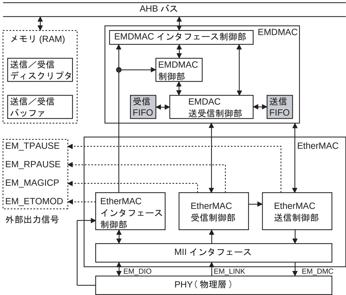
図 20-1 EtherMAC の構成
