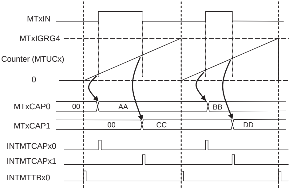
図 24-10 キャプチャ動作
