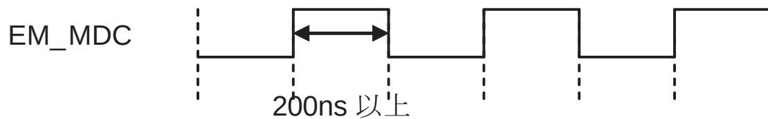
図 20-14 EM_MDC 信号
