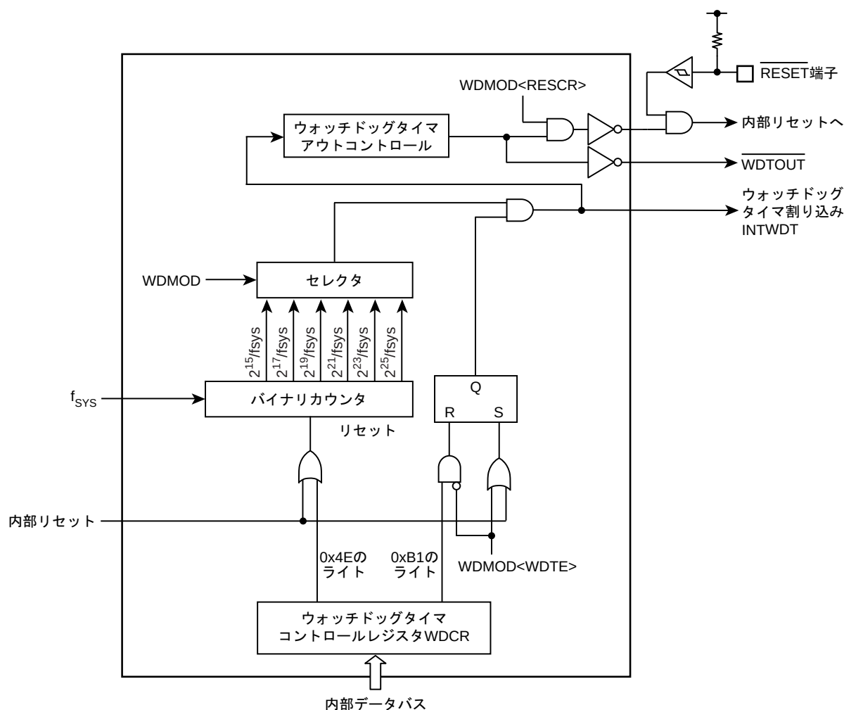
図 30-1 ウォッチドッグタイマのブロック図
