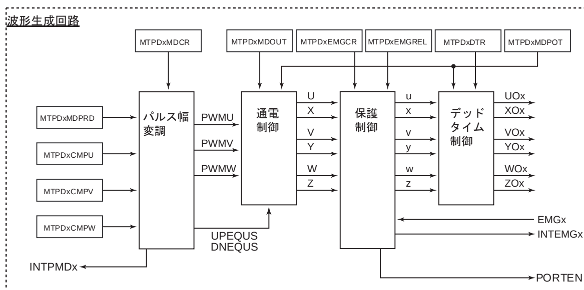
図 24-21 PMD 回路概略図
