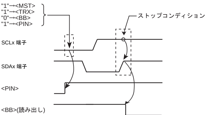
図 14-13 ストップコンディションの発生
