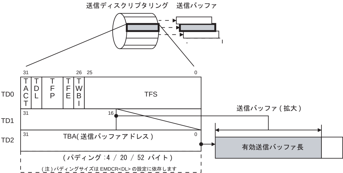
図 20-4 送信ディスクリプタと送信バッファの関係
