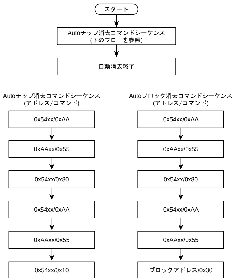
図 31-12 自動消去
