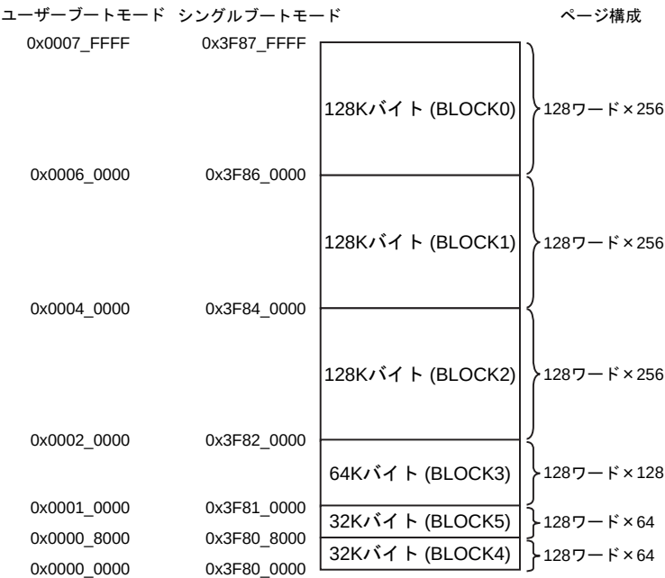
図 31-10 ブロック構成(TMPM369FDFG/XBG)
