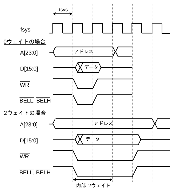
図 10-6 ライトオペレーションタイミング
