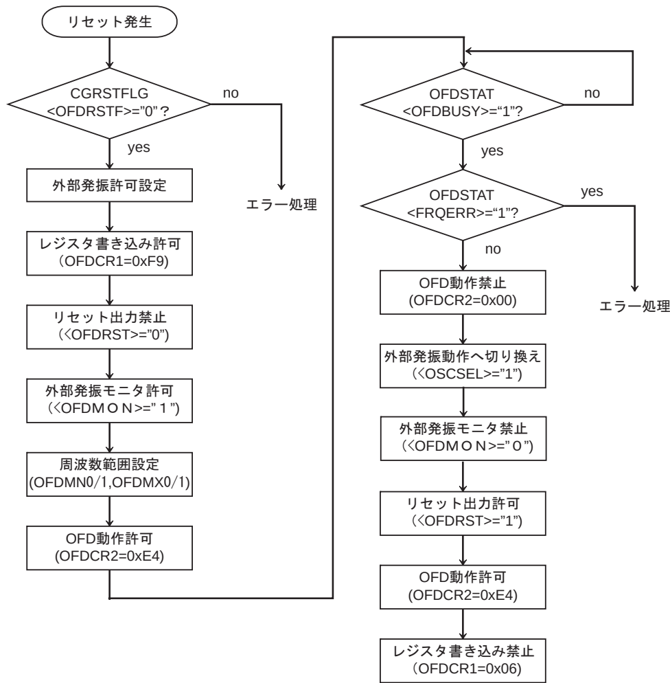
図 29-3 動作手順例
