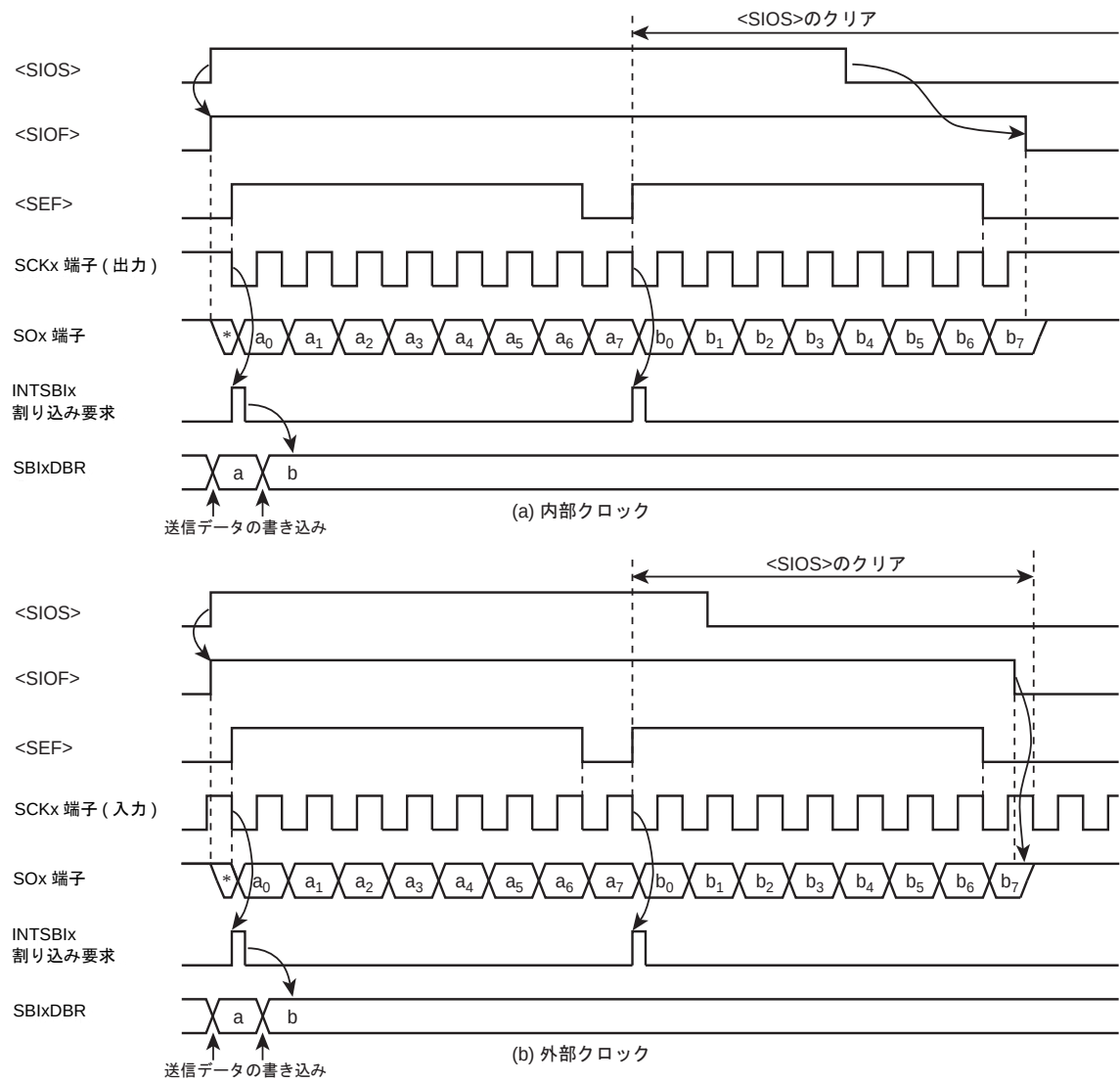
図 14-18 送信モード
