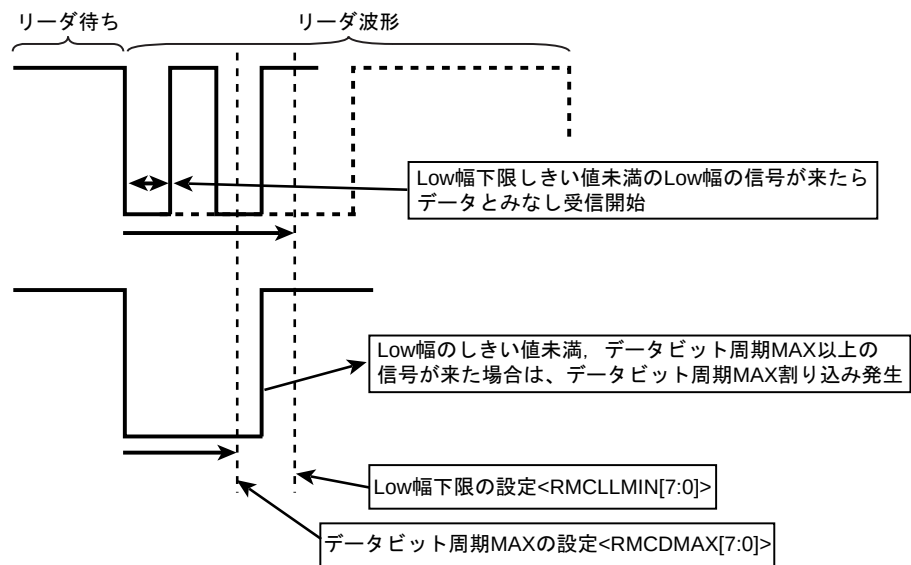
図 21-8 リーダ待ち状態なしでのリーダーなしのリモコン信号の場合 (RMCRCR2<RMCLD>="1"の時)
