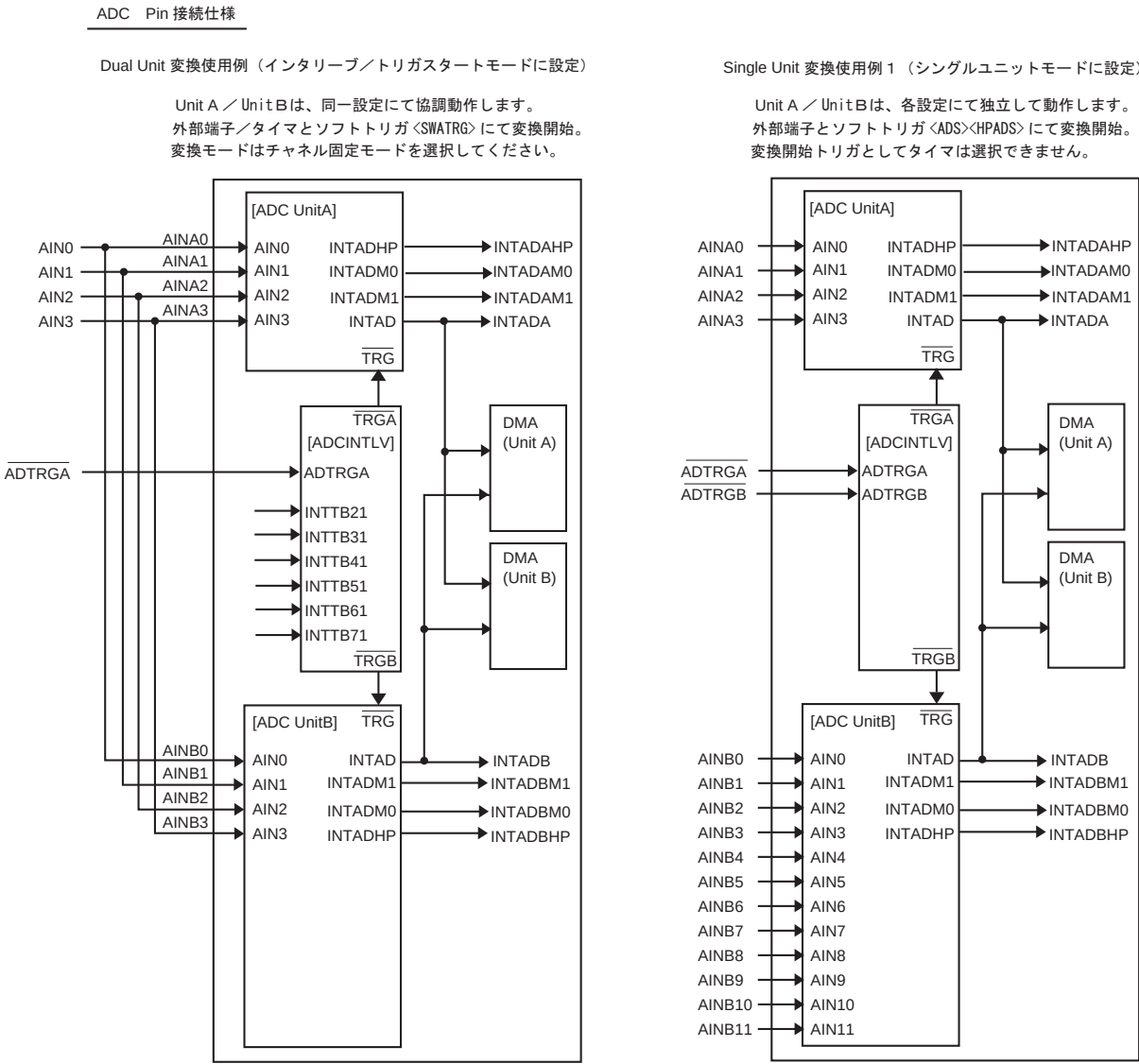
図 22-1 ブロック図 1
