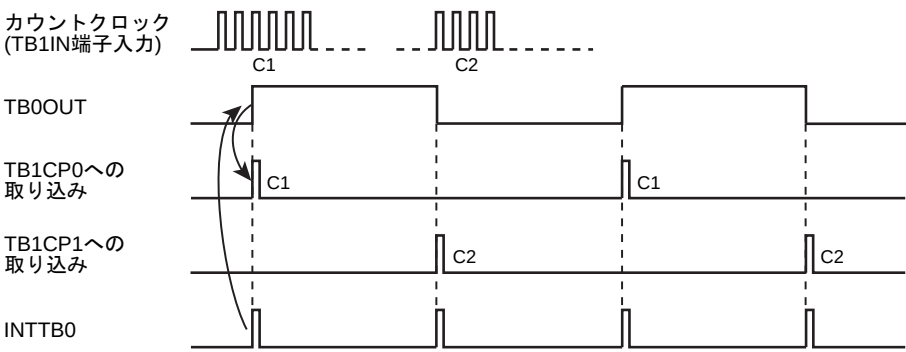
図 11-7 周波数測定
