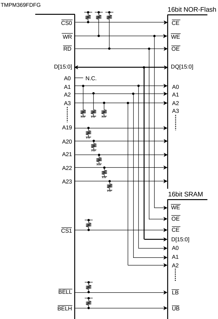
図 10-19 外部 16 ビット SRAM、NOR-Flash 接続例(セパレートバス)
