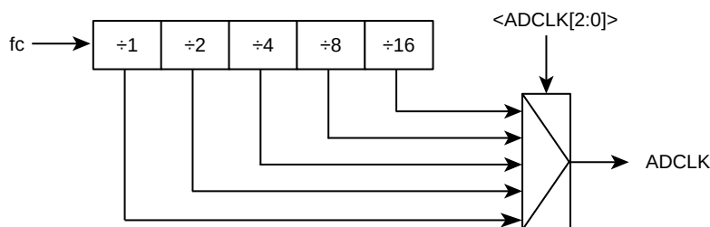
図 22-4 AD 変換クロック(ADCLK)
