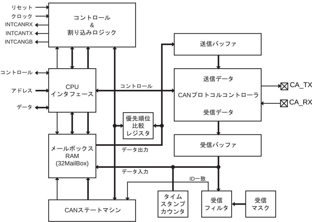
図 19-1 CAN コントローラのブロック図
