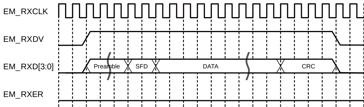
図 20-8 MII フレーム受信タイミング(正常受信時)
