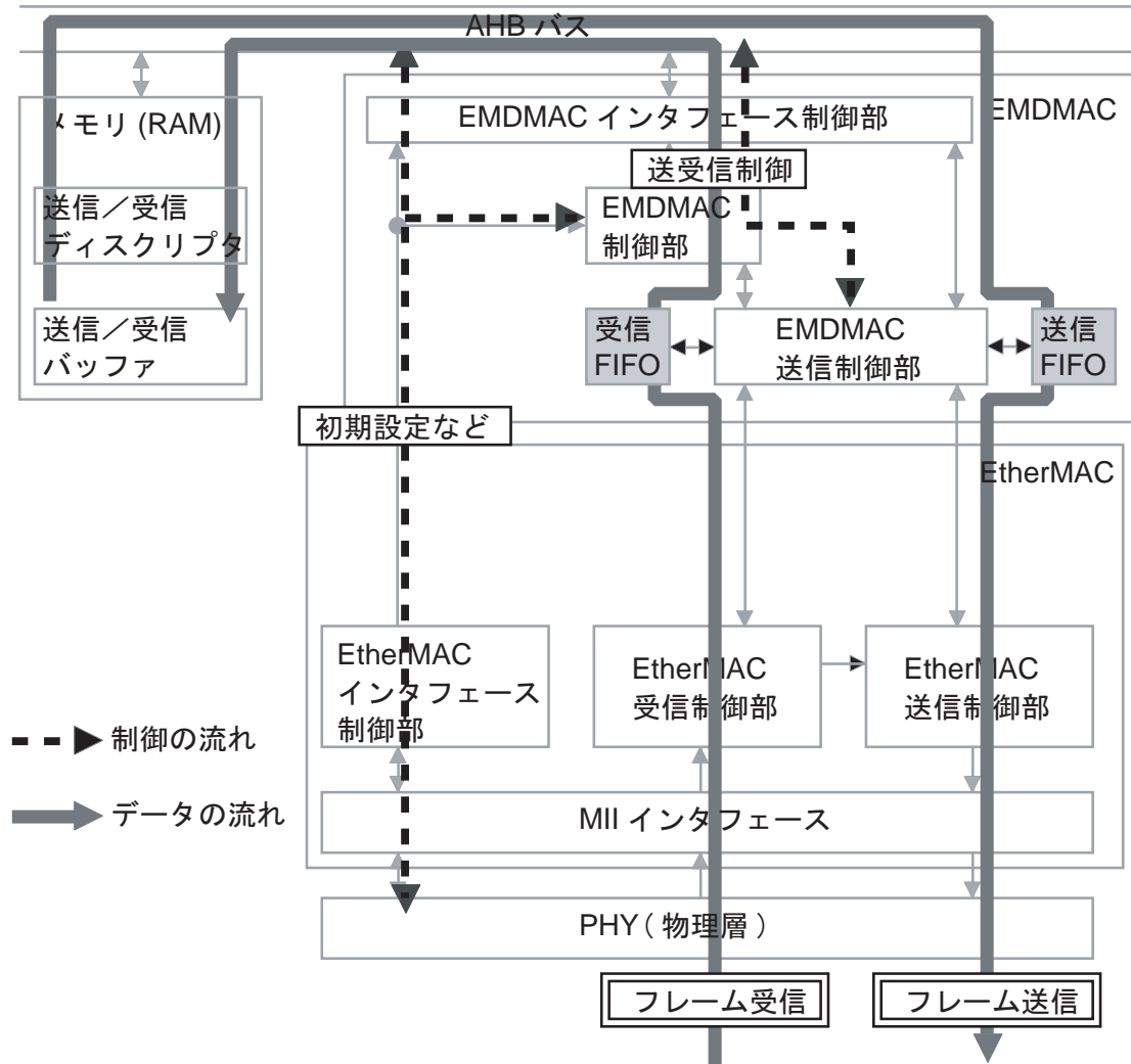
図 20-2 制御とフレームデータの流れ
