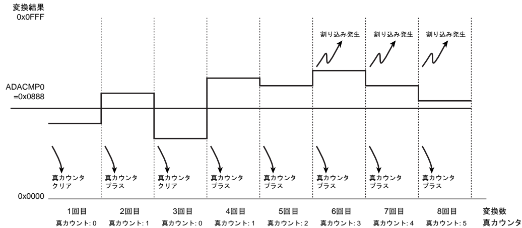
図 22-5 AD 監視機能（チャンネル固定リピート、判定カウント連続方式）
