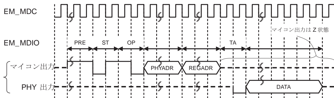
図 20-16 MII 制御フレームタイミング(リード時)
