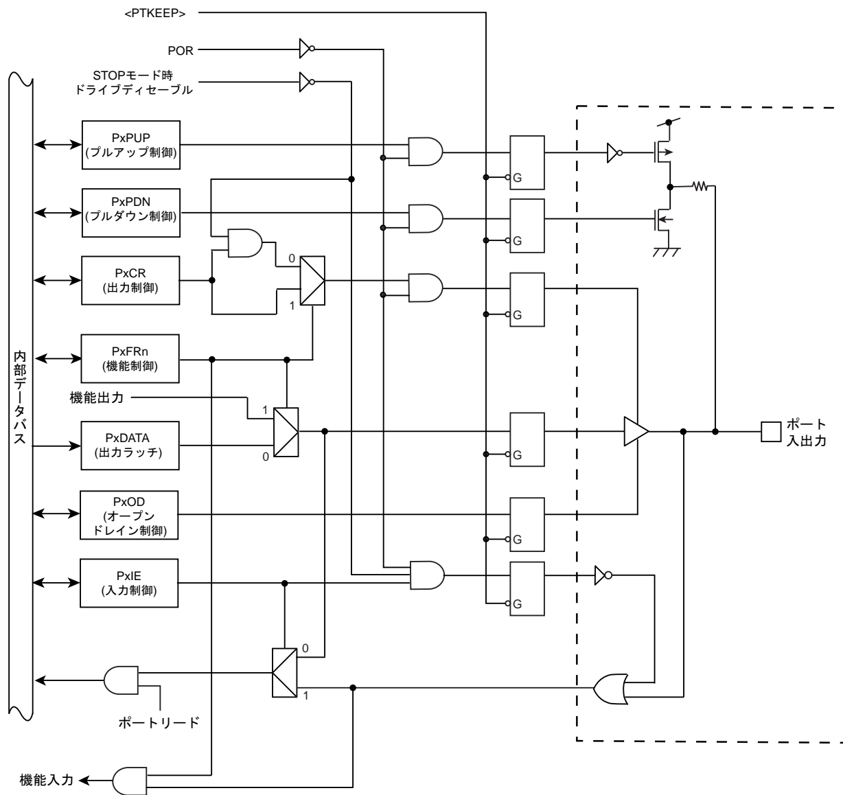
図 9-9 ポートタイプ FT9
