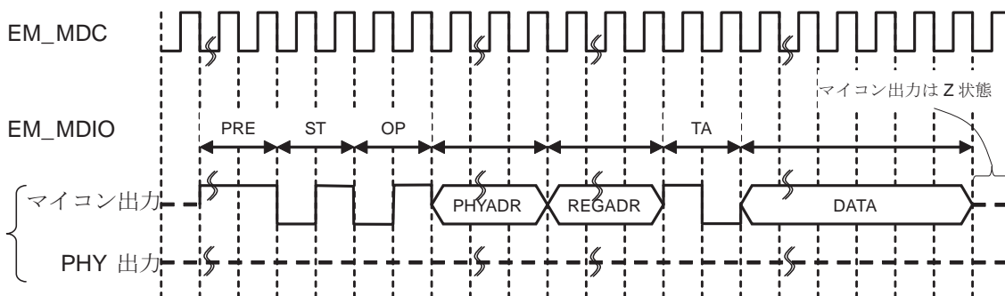
図 20-15 MII 制御フレームタイミング(ライト時)
