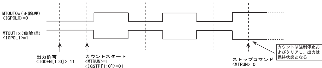
図 24-14 出力保持状態でカウント停止
