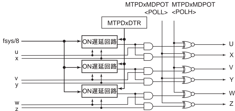
図 24-26 デッドタイム回路概略図
