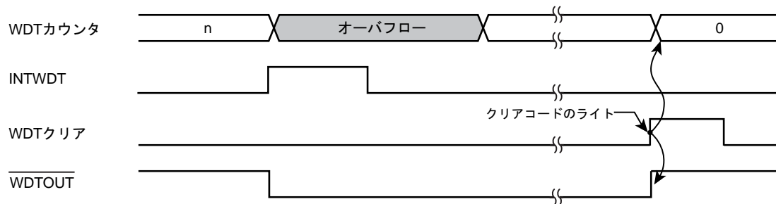
図 30-2 INTWDT 割り込み発生
