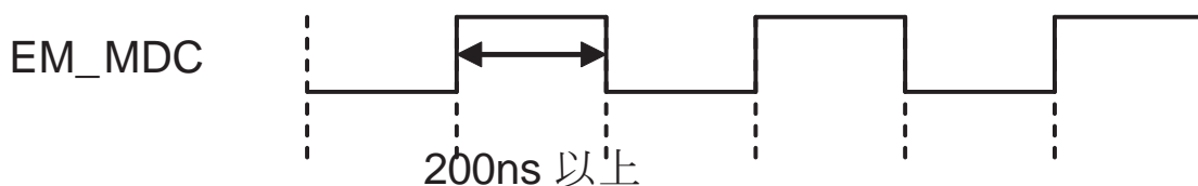
図 20-14 EM_MDC 信号
