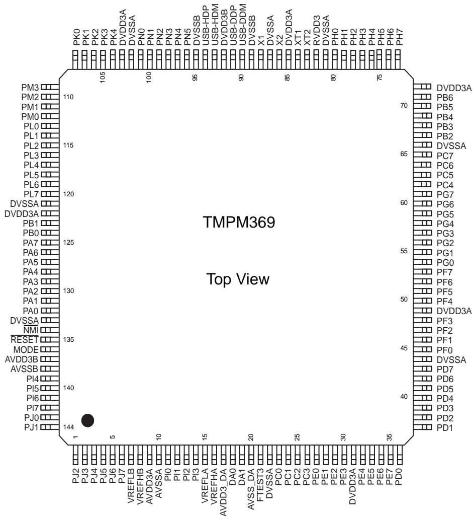
図 1-2 ピン配置図
