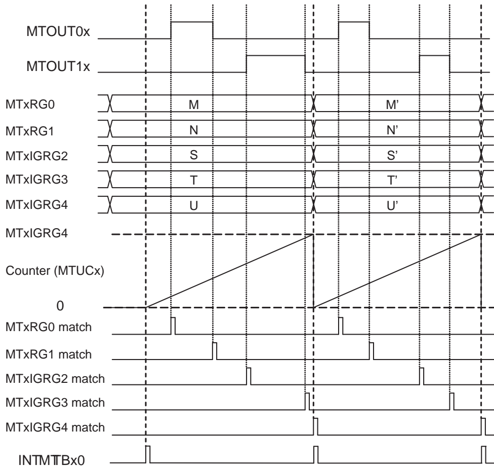
図 24-8 IGBT モード基本タイミング
