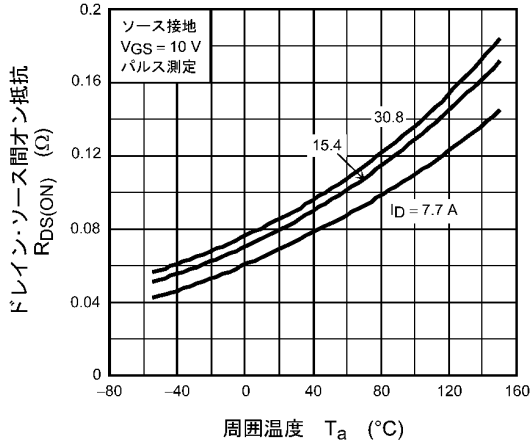
図 8.7 R_{DS(ON)} - T_a
