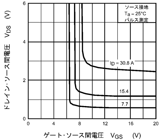
図 8.4 V_{DS} - V_{GS}
