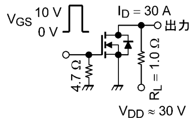
図 6.2.1 スwitching時間の測定回路
