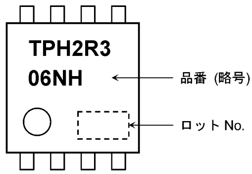
図 7.1 現品表示
