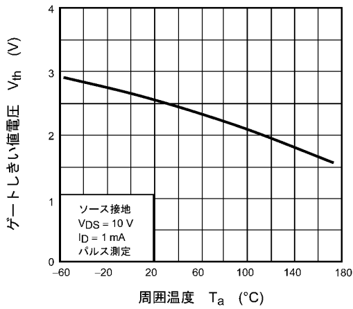
図 8.9 V_{th} - T_a (注7)
