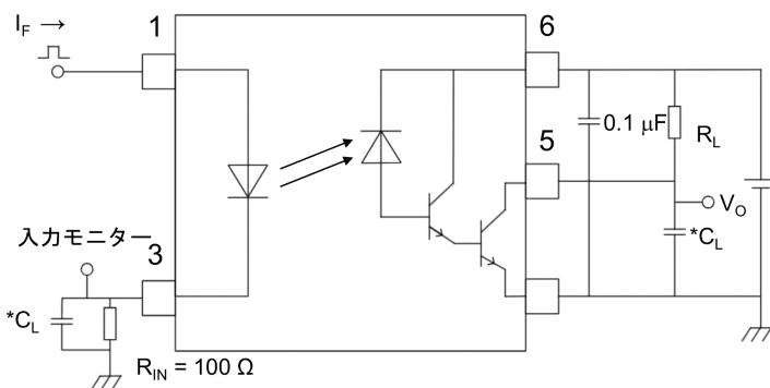
図 12.1.6 伝搬遅延時間測定回路, 波形
