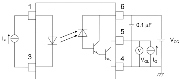
図 12.1.5 V OL 測定回路
