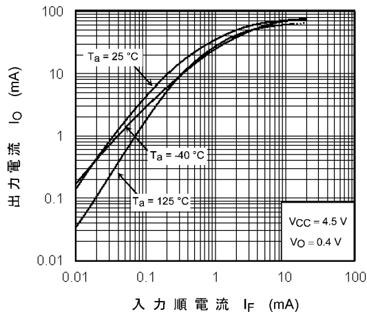
图 12.2.7 I_O - I_F
