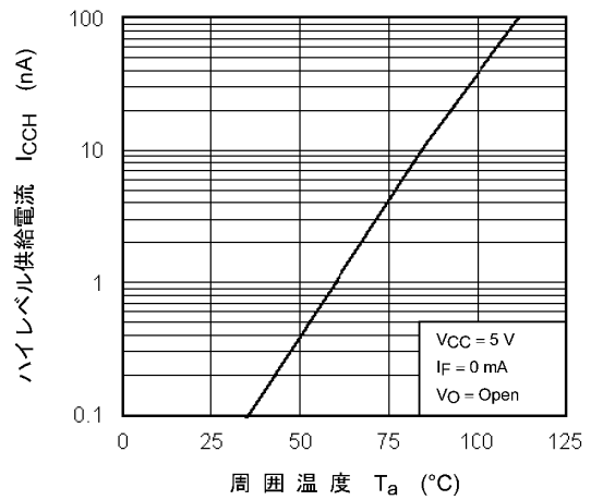
図 12.2.4 I_{CCH} - T_a
