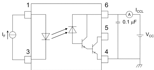
図 12.1.3 I CCL 測定回路
