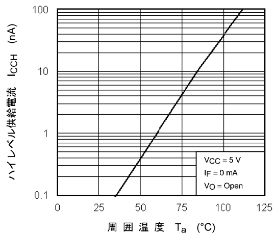
図 12.2.4 I_{CCH} - T_a
