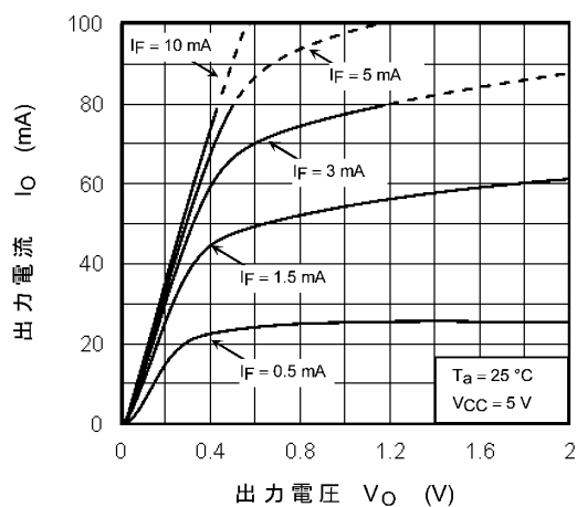
图 12.2.11 I_O - V_O
