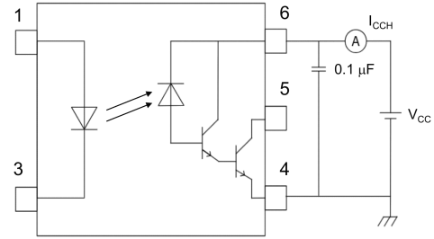
図 12.1.2 I CCH 測定回路
