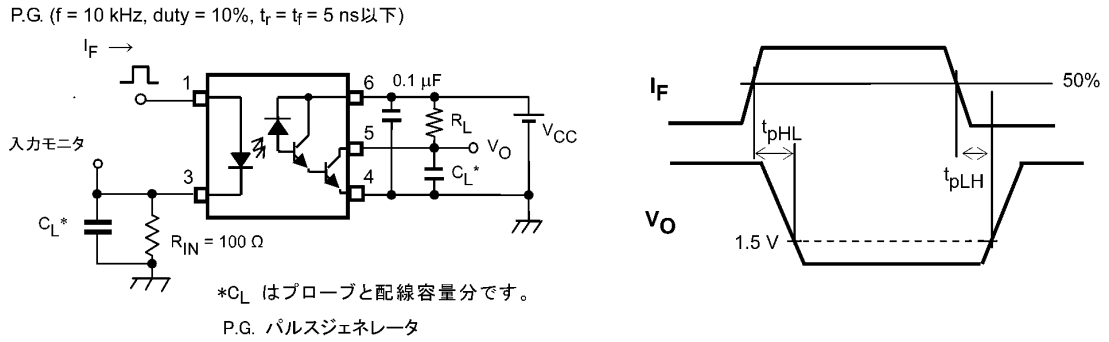
図 12.1.1 伝搬遅延時間測定回路, 波形
