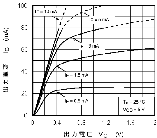
图 12.2.11 I_O - V_O
