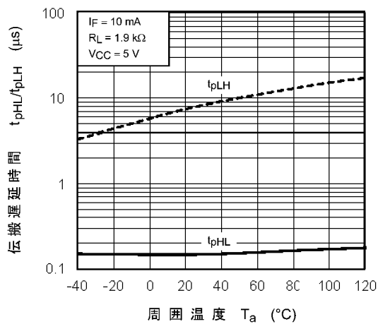
図 12.2.15 t_{pHL}, t_{pLH} - T_a
