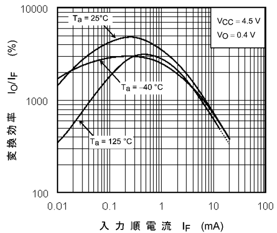
图 12.2.8 I_O/I_F - I_F
