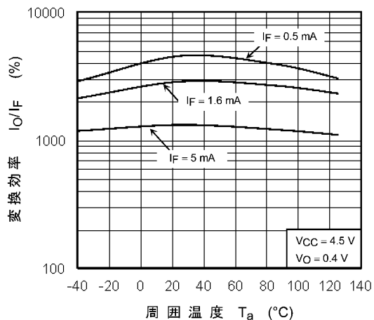
图 12.2.9 I_O/I_F - T_a
