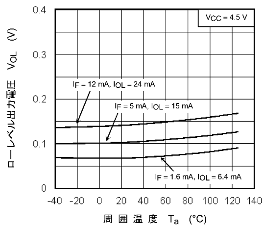
図 12.2.6 V_{OL} - T_a
