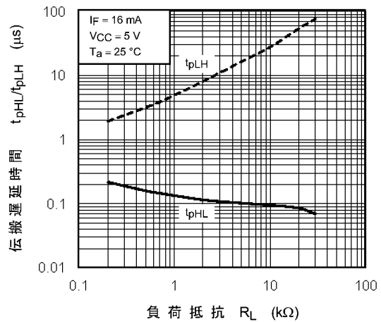
図 12.2.18 t_{pHL}, t_{pLH} - R_L
