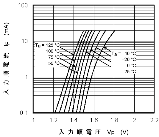
図 12.2.1 I_F - V_F
