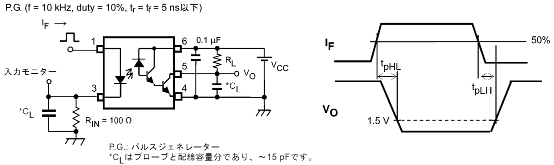
図 12.1.1 伝搬遅延時間測定回路, 波形
