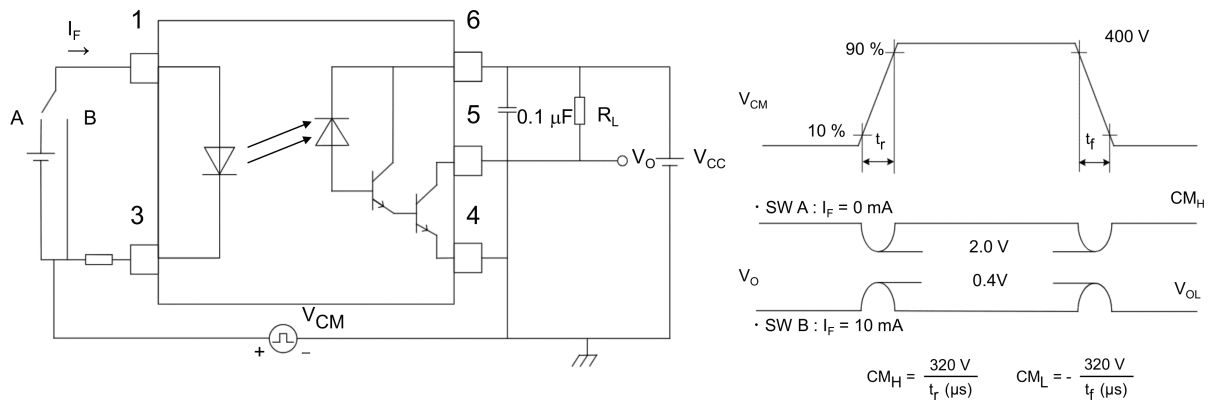
図 12.1.7 コモンモード過渡耐性測定回路, 波形
