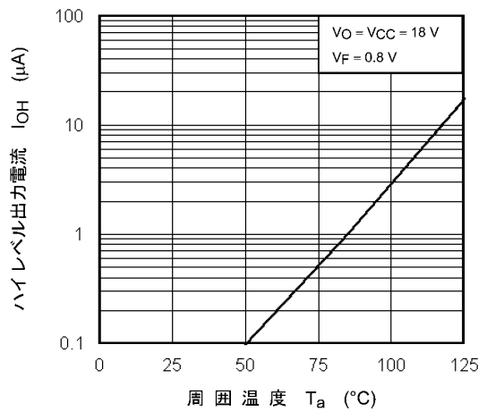
図 12.2.3 I_{OH} - T_a
