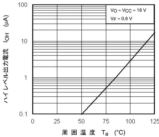
図 12.2.3 I_{OH} - T_a
