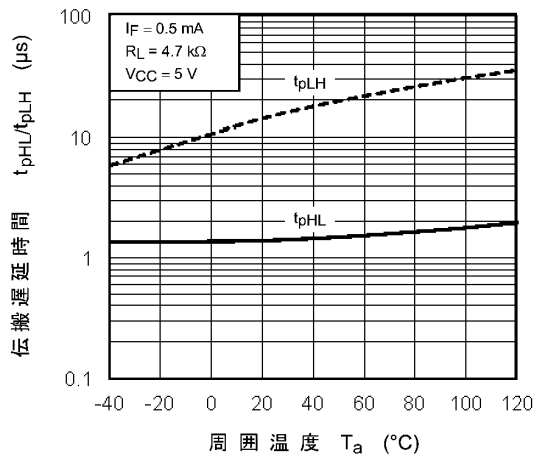
図 12.2.13 t_{pHL}, t_{pLH} - T_a
