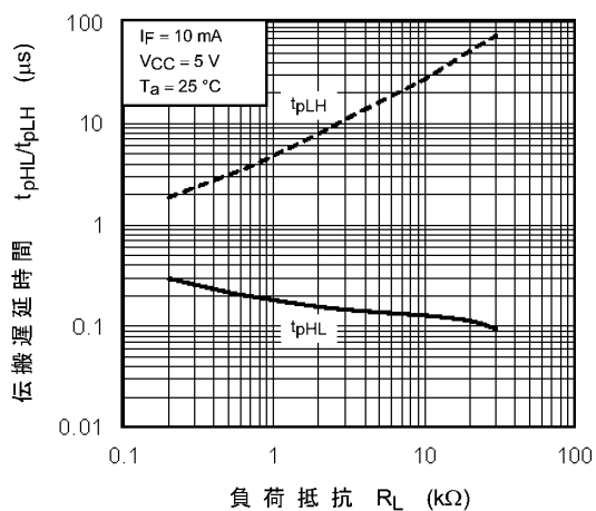
図 12.2.17 t_{pHL}, t_{pLH} - R_L
