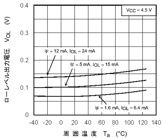
図 12.2.6 V_{OL} - T_a
