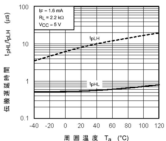
图 12.2.12 t_{pHL}, t_{pLH} - T_a
