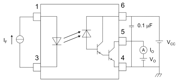
図 12.1.4 I O 測定回路
