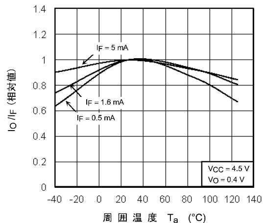
图 12.2.10 I_O/I_F - T_a
