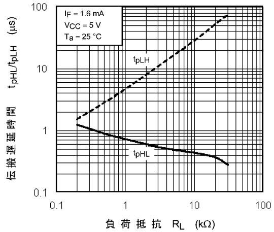
図 12.2.16 t_{pHL}, t_{pLH} - R_L
