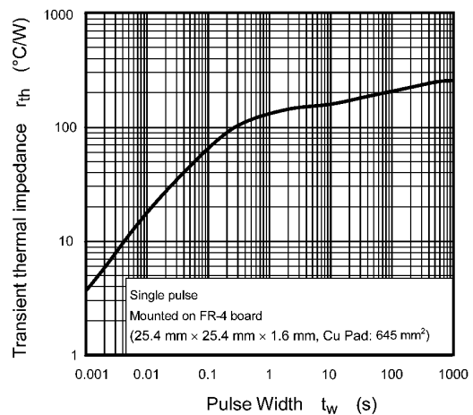
Fig. 7.12 r_{th} - t_w
