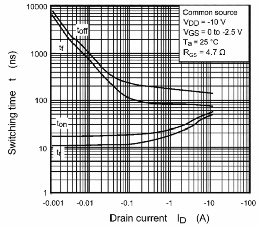
Fig. 7.10 t - I_D
