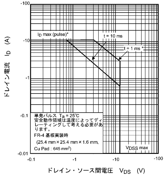
図 7.14 安全動作領域
