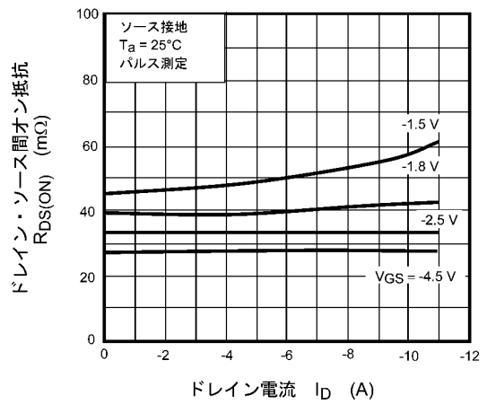
図 7.4 R_{DS(ON)} - I_D
