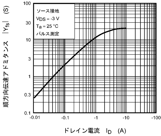
図 7.7 |Y_{fs}| - I_D
