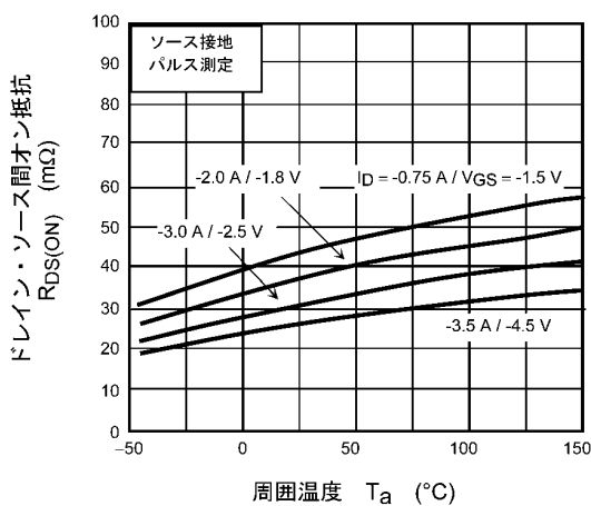
図 7.5 R_{DS(ON)} - T_a
