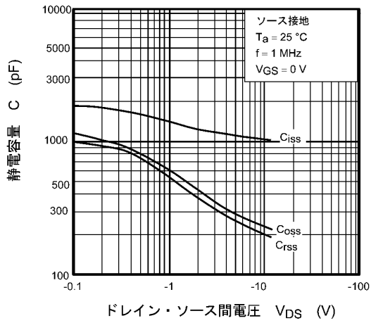
図 7.9 C - V_{DS}
