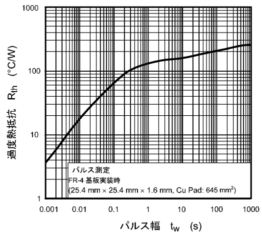
図 7.12 r_{th} - t_w
