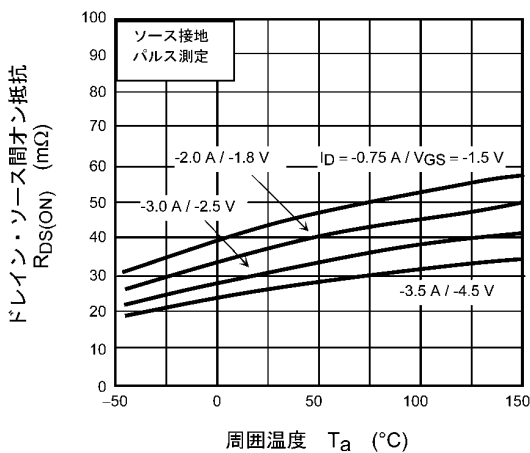
図 7.5 R_{DS(ON)} - T_a
