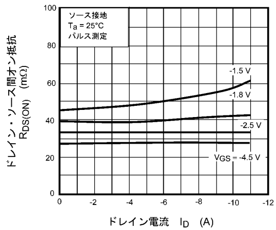
図 7.4 R_{DS(ON)} - I_D
