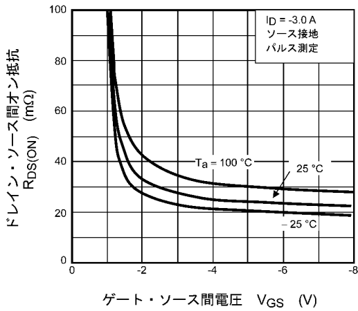
図 7.3 R_{DS(ON)} - V_{GS}
