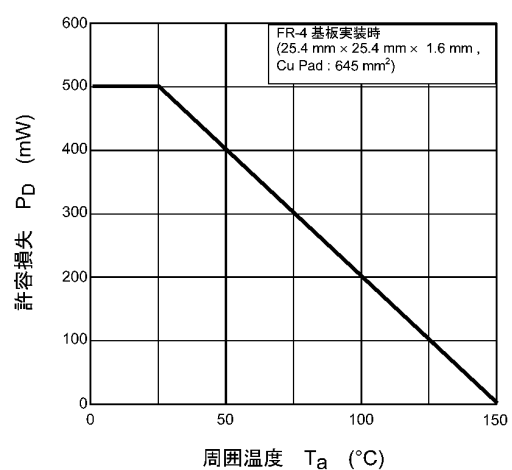
図 7.12 P_D - T_a
