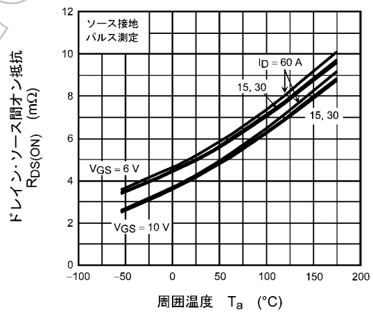
図 8.6 R_{DS(ON)} - T_a (注7)
