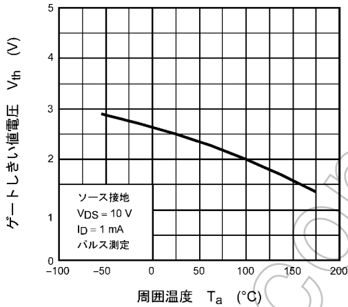
図 8.9 V_{th} - T_a (注7)
