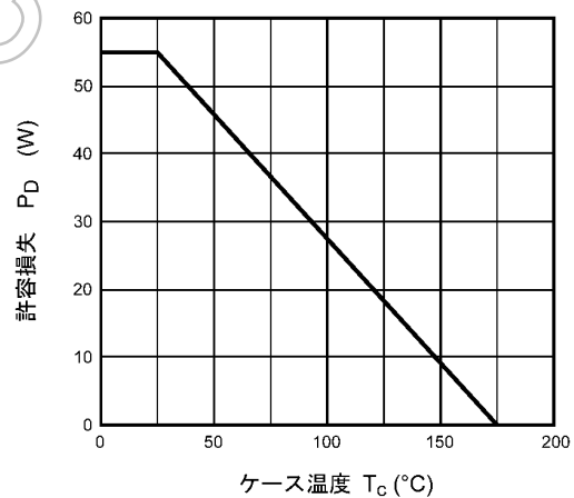
図 8.12 P_D - T_c (注7) (最大値 (保証値))
