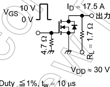
図 6.2.1 スイッチング時間の測定回路例
