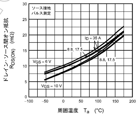
図 8.6 R_{DS(ON)} - T_a (注7)
