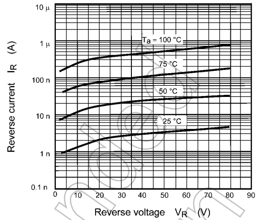
Fig. 7.2.2 I_R - V_R
