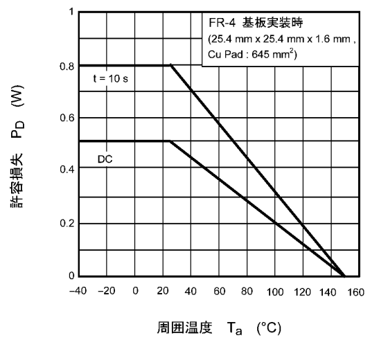
図 7.1.12 P_D - T_a
