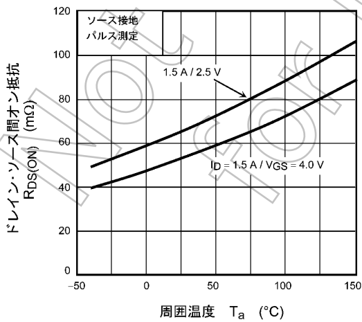
図 7.1.5 R_{DS(ON)} - T_a
