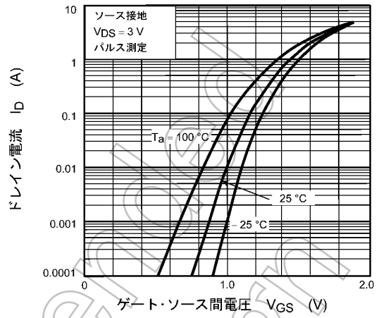
図 7.1.2 I_D - V_{GS}
