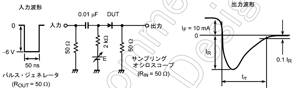
図 5.5.1 逆回復時間の測定回路/波形
