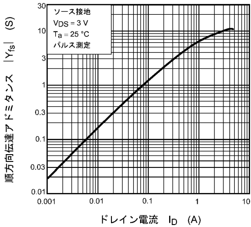
図 7.1.7 |Y_{fs}| - I_D
