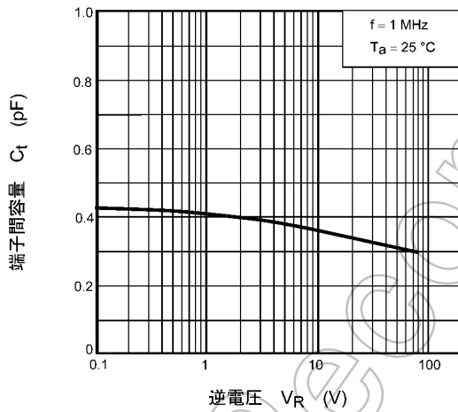
図 7.2.3 C_t - V_R
