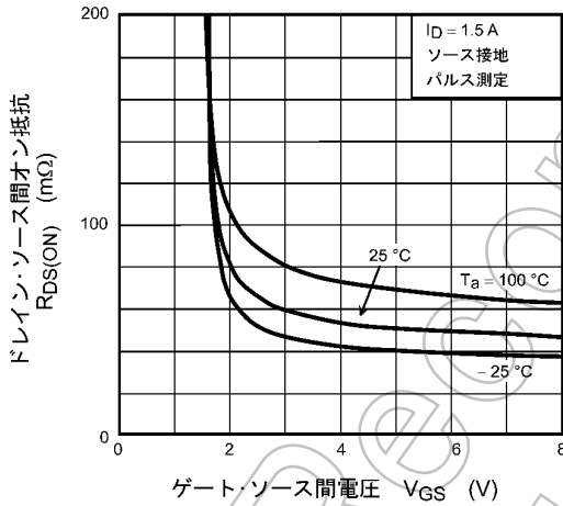
図 7.1.3 R_{DS(ON)} - V_{GS}
