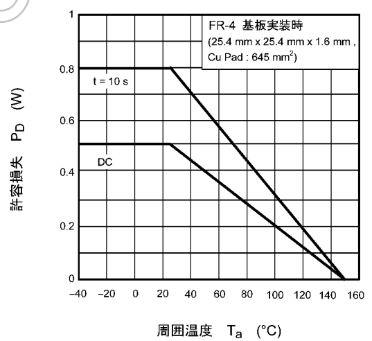
図 7.1.12 P_D - T_a
