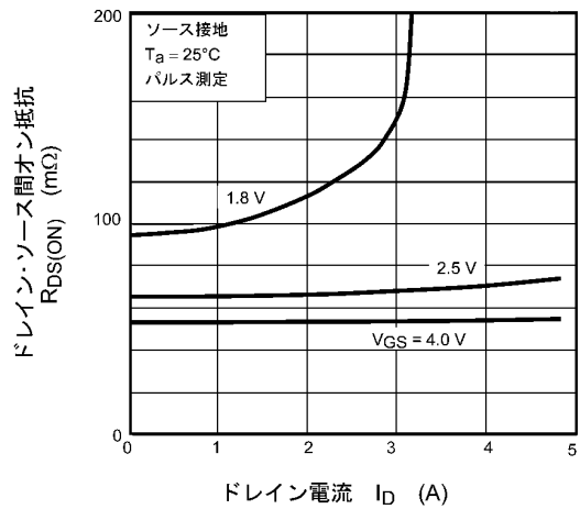
図 7.1.4 R_{DS(ON)} - I_D
