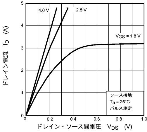
図 7.1.1 I_D - V_{DS}
