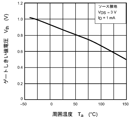
図 7.1.6 V_{th} - T_a
