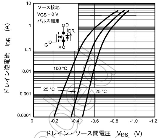
図 7.1.8 I_{DR} - V_{DS}
