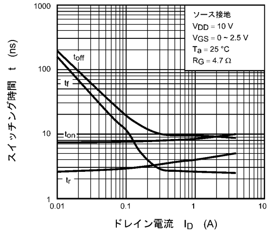
図 7.1.10 t - I_D
