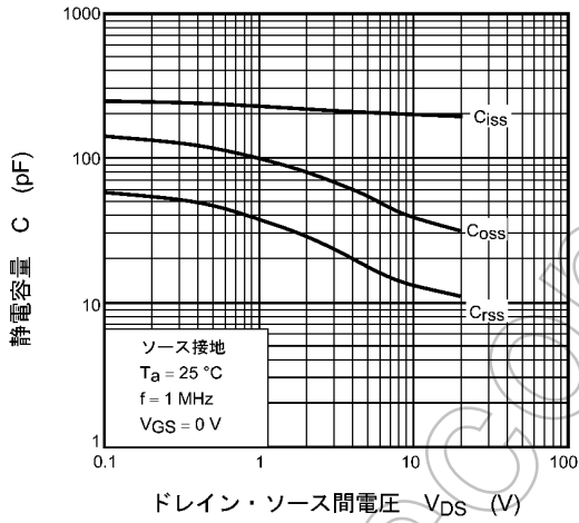
図 7.1.9 C - V_{DS}
