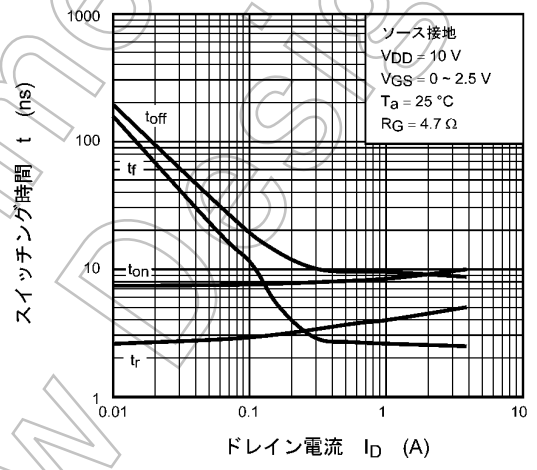
図 7.1.10 t - I_D
