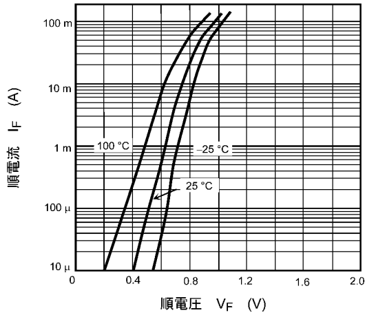
図 7.2.1 I_F - V_F
