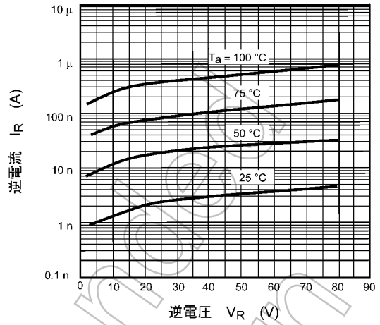
図 7.2.2 I_R - V_R
