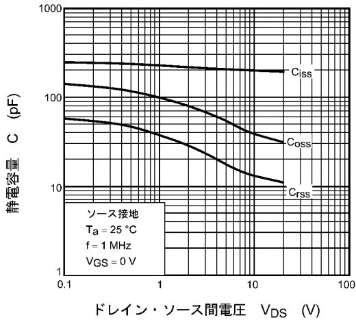
図 7.1.9 C - V_{DS}
