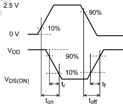
図 5.2.2 入力波形/出力波形
