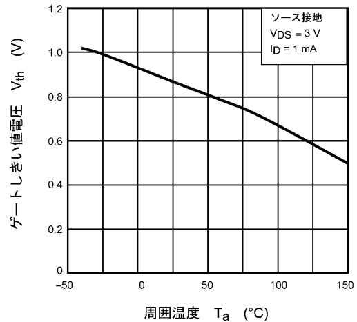
図 7.1.6 V_{th} - T_a
