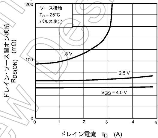
図 7.1.4 R_{DS(ON)} - I_D
