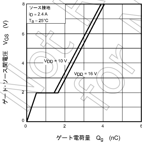
図 7.1.11 ダイナミック入力特性
