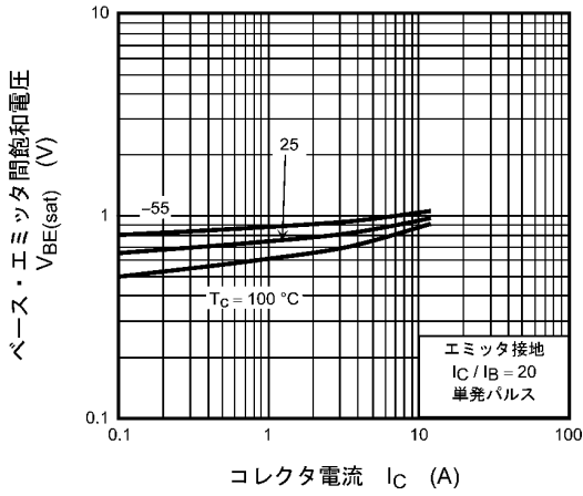
図 7.7 V_{BE(sat)} - I_C
