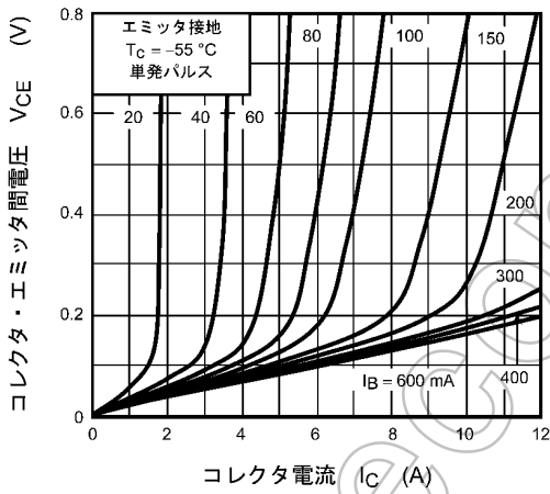
図 7.3 V_{ce} - I_c
