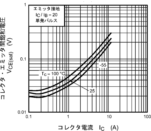
図 7.6 V_{ce(sat)} - I_c
