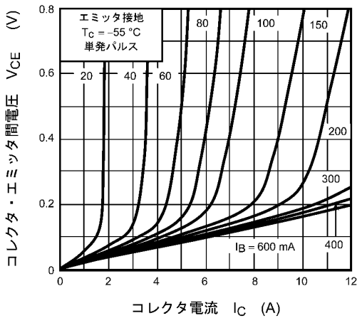
図 7.3 V_{CE} - I_c
