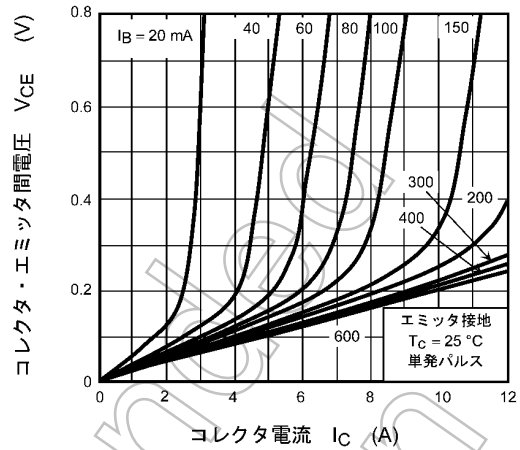
図 7.2 V_{ce} - I_c
