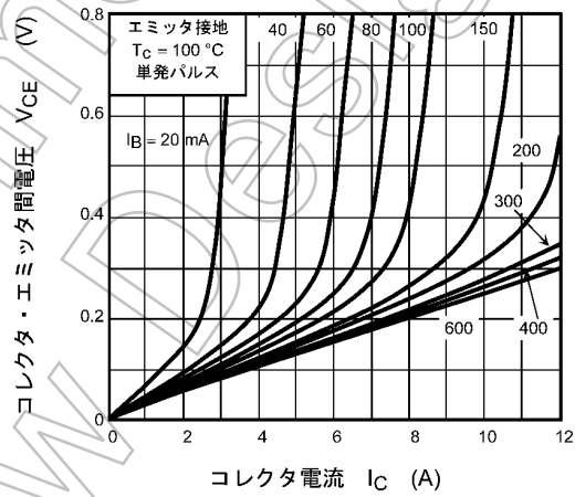
図 7.4 V_{ce} - I_c
