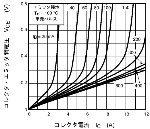
図 7.4 V_{CE} - I_c
