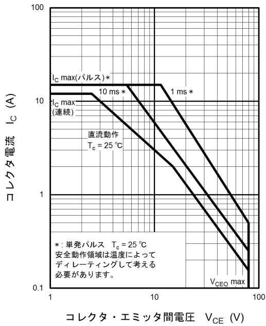
図 7.11 安全動作領域 (最大値 (保証値))
