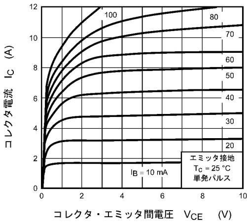
図 7.1 I_c - V_{ce}
