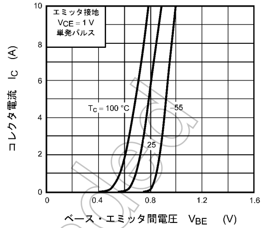
図 7.8 I_C - V_{BE}
