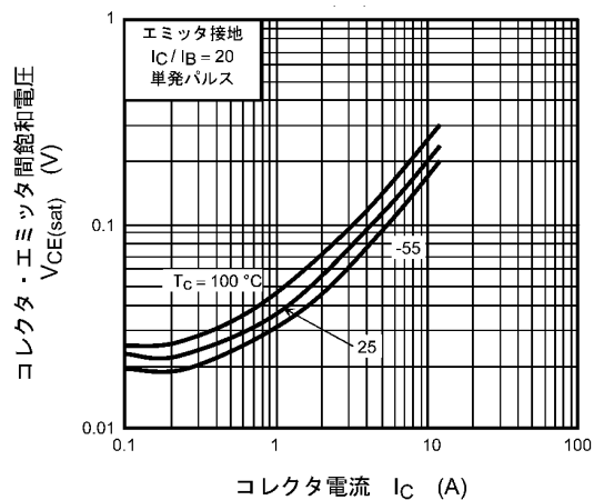
図 7.6 V_{CE(sat)} - I_c
