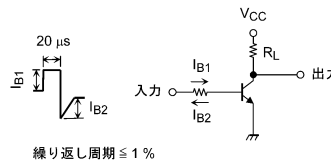
図 5.2.1 スwitching時間の測定回路
