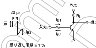
図 5.2.1 スwitchング時間の測定回路
